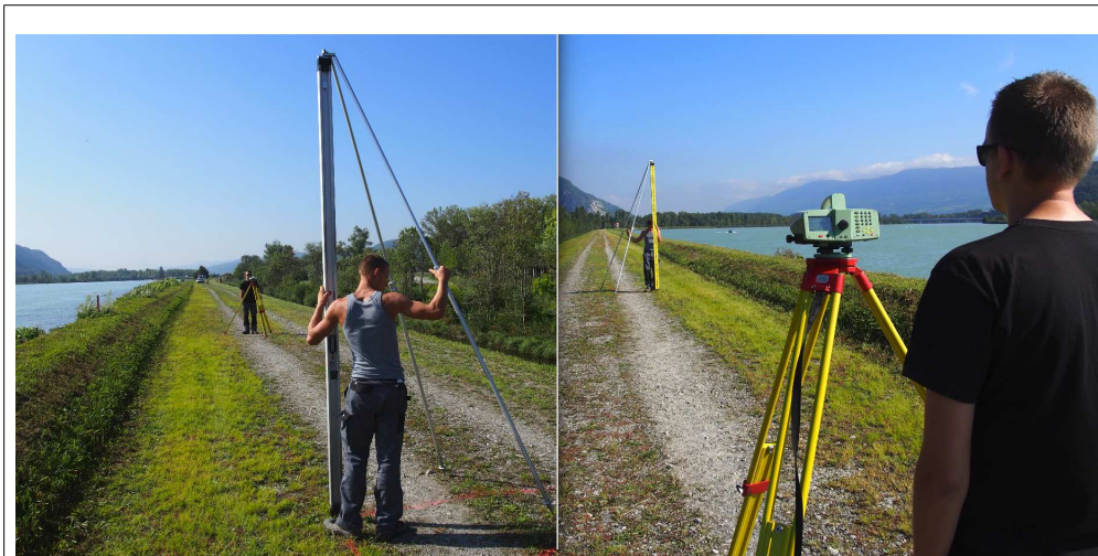
Illustration 74: Rattachement altimétrique des repères topographiques
