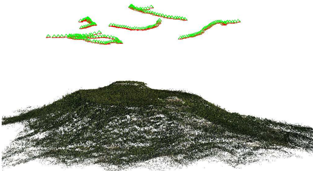
Figure 50: Résultat du calcul d'aérottriangulation (relatif). Position 3D des points homologues et des sommets de prise de vue orientés
