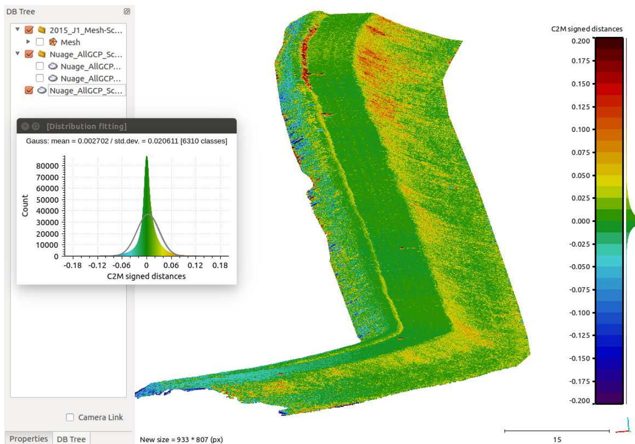
Figure 90: Test de répétabilité entre Palliere-2015a et Palliere-2015b, tous générés en utilisant 71 points d'appui. La comparaison nuage à maillage, effectuée avec le logiciel CloudCompare, fait apparaître de faibles écarts sur le chemin, dépourvu de végétation. En revanche, les zones enherbées sont plus complexes à modéliser.
