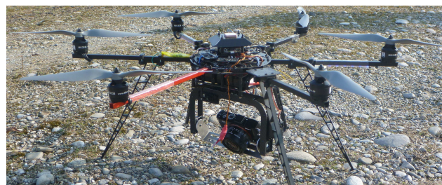
Figure 42: Mikrocopter HexaXL de l'IGN avec le Sony DSC-RX1 sur une nacelle gyroscopiquement stabilisée
