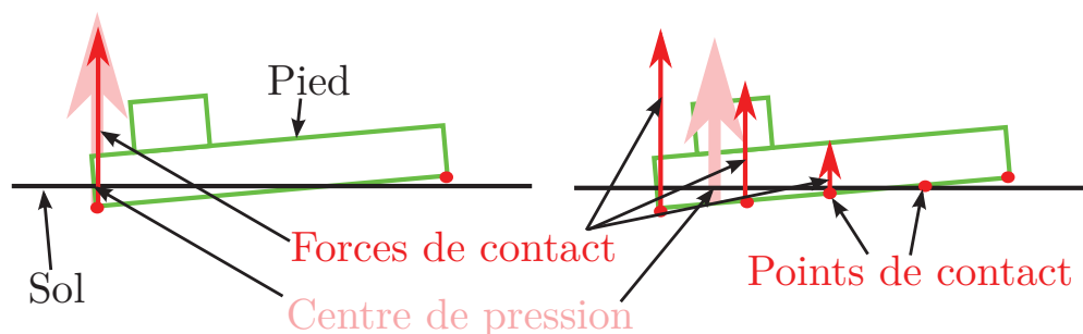
Figure 4.3: La multiplication des points de contact permet un calcul précis du centre de pression dans le polygone de sustentation quand le pied n'est pas parfaitement à plat.
