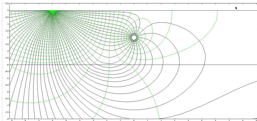
FIGURE 3.2.27 – Lignes de courant et équipotentielles en sol b-couche.
