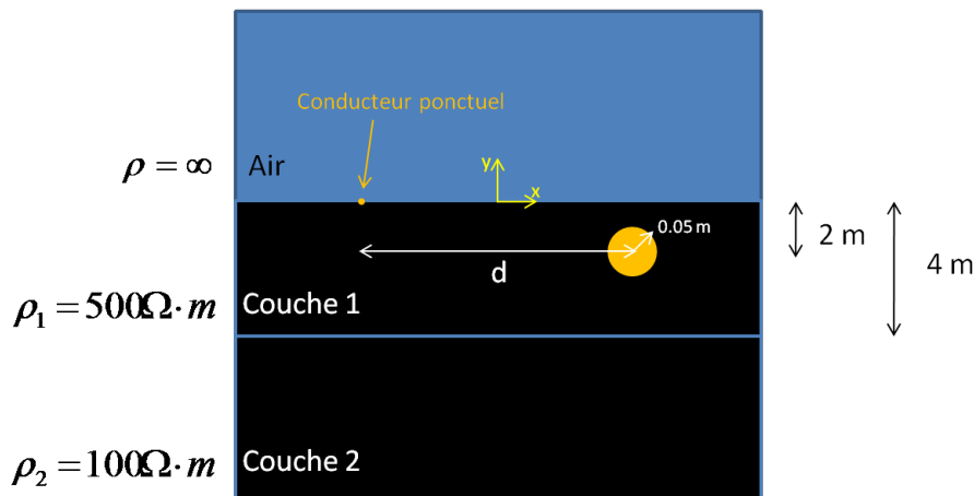
FIGURE 3.2.26 – Configuration étudiée, avec un conducteur ponctuel en surface et un conducteur cylindrique enterré en sol multicouche
