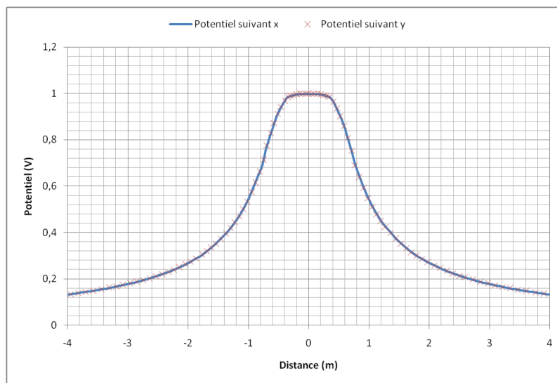
FIGURE 3.4.4 – Superposition du potentiel suivant x et suivant y , pour une plaque enterrée sous tension.
