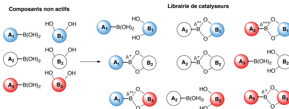
Schéma 3. Génération in situ d'une librairie de catalyseurs à partir de composants non actifs.
