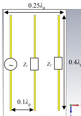
Figure I.32 Réseau planaire à deux éléments parasites
