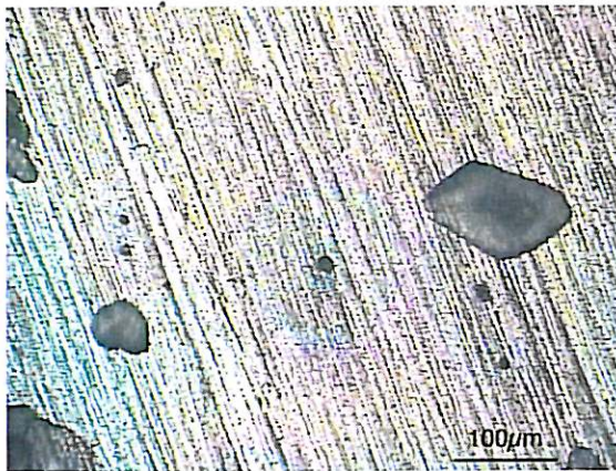
Figure II.B-10 : Photo optique ex-situ de la surface de l'acier X70 après 28 jours sous PC (-1125mV/ECS) dans l'eau siliceuse aérée.
