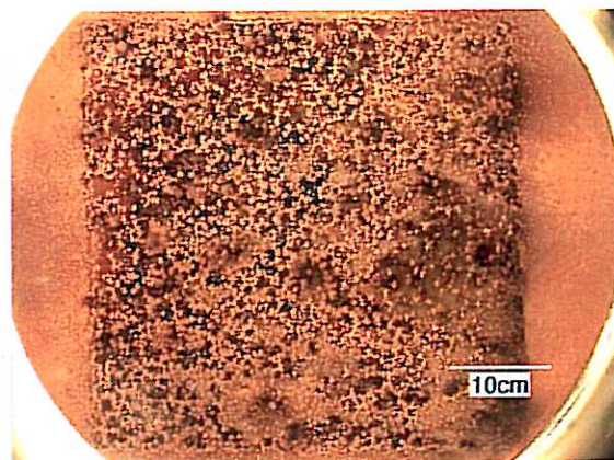
Figure II.A-6 : Photo optique de la surface de l'acier X70, après 28 jours de CL dans l'eau siliceuse aérée.
