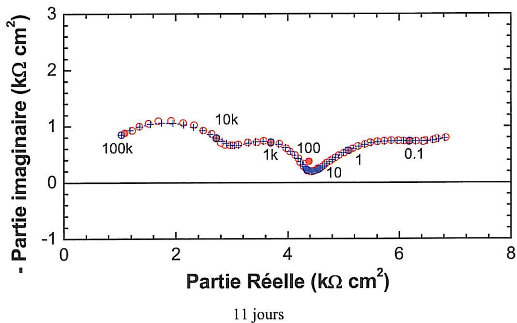
Figure II.A-16 : Diagrammes d'impédances de l'acier X70 laissé au potentiel de circuit ouvert, en fonction du temps d'immersion dans l'eau siliceuse aérée, rond : expérimental – croix : modèle électrique
