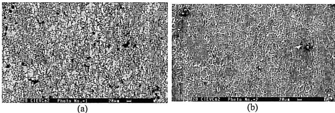
Figure III.A-12 : Images MEB de la surface de l'acier, après 28 jours de CL, dans l'eau carbonatée désaérée saturée en calcite. (a) Electrons rétrodiffusés. (b) Electrons secondaires.
