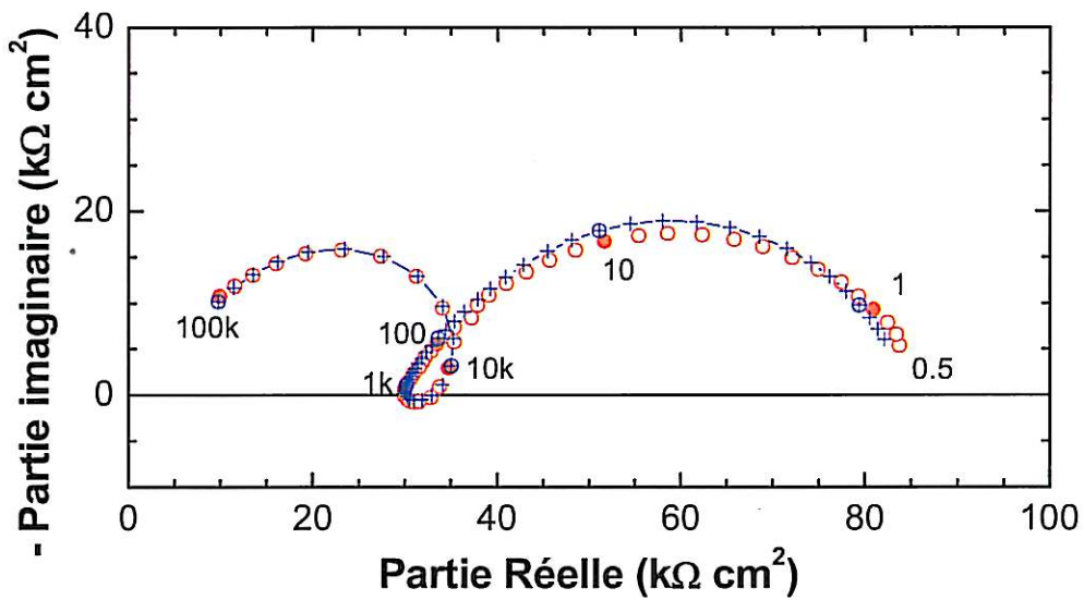
Figure IV.B-9 : Diagrammes d'impédances de l'acier X70, laissé au potentiel de circuit pendant 14 jours suivi de 14 jours sous polarisation cathodique à -1125mV/ECS, en fonction du temps d'immersion dans l'eau bi-carbonatée désaérée, rond : expérimental – croix : modèle électrique
