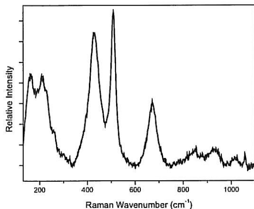
Figure III.A-2 : Spectre Raman in-situ enregistré sur une zone sombre à la surface de l'acier X70, après 21 heures de CL ( \approx -655\text{mV/ECS} ) dans une solution bi-carbonatée désaérée synthétique.
