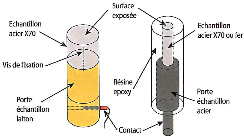
Figure IV.C-2 : Echantillons montés sur les porte-échantillons associés à la cellule spectro-électrochimique
