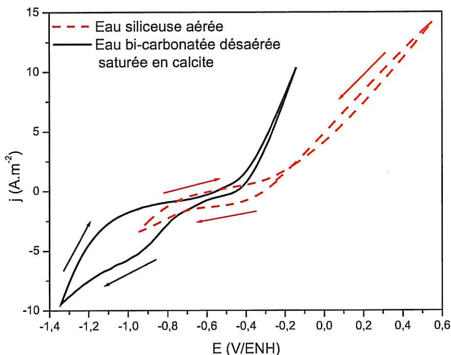
Figure IV.C-1 : Voltammogrammes cycliques de l'acier X70 dans l'eau siliceuse aérée (rouge - gras) et dans l'eau bi-carbonatée désaérée saturée en calcite (noir). La vitesse de balayage en potentiel est de 20\text{mV}\cdot\text{s}^{-1} .
