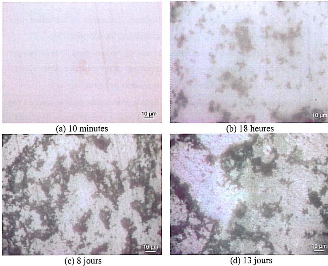
Figure I.B-5 : Photos optiques in-situ de la surface de l'acier X70 sous PC (-925mV/ECS) dans l'eau siliceuse aérée après (a) 10 minutes, (b) 18 heures, (c) 8 jours et (d) 13 jours.
