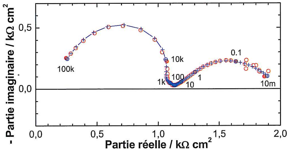
Figure IV.A-9 : Diagrammes d'impédances de l'acier X70, laissé au potentiel de circuit pendant 14 jours suivi de 14 jours sous polarisation cathodique à -1125\text{mV/ECS} , en fonction du temps d'immersion dans l'eau siliceuse aérée, rond : expérimental – croix : modèle électrique
