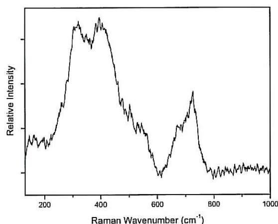
Figure II.B-13 : Spectre Raman ex-situ enregistré sur les produits de corrosion marron formés à la surface de l'acier X70, sous le dépôt, après 28 jours sous PC (-1125mV/ECS) dans l'eau siliceuse aérée (Figure II.B-12).
