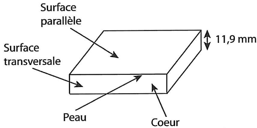
Figure III.B-1 : Surfaces de l'acier X70 attaquées chimiquement.
