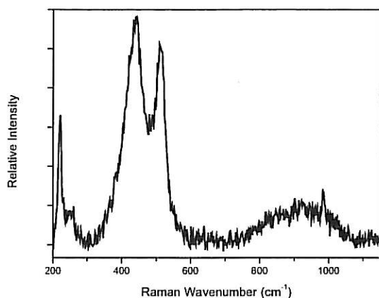
Figure V.B-8 : Spectre Raman ex-situ, enregistré sur un cristal verdâtre. Compiègne – PC permanente
