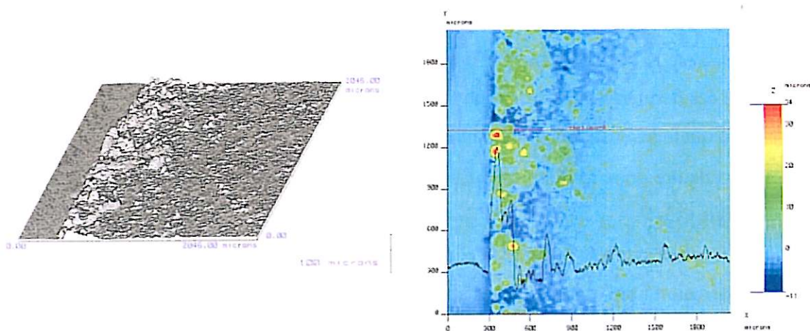
Figure II.B-18 : Cartographie topographique (MMB) de la surface de l'acier X70 décapée, après 4 semaines sous PC ( -1125\text{mV/ECS} ) dans l'eau siliceuse aérée - pas de mesure = 2\mu\text{m} , S = 4,194\text{mm}^2 .
