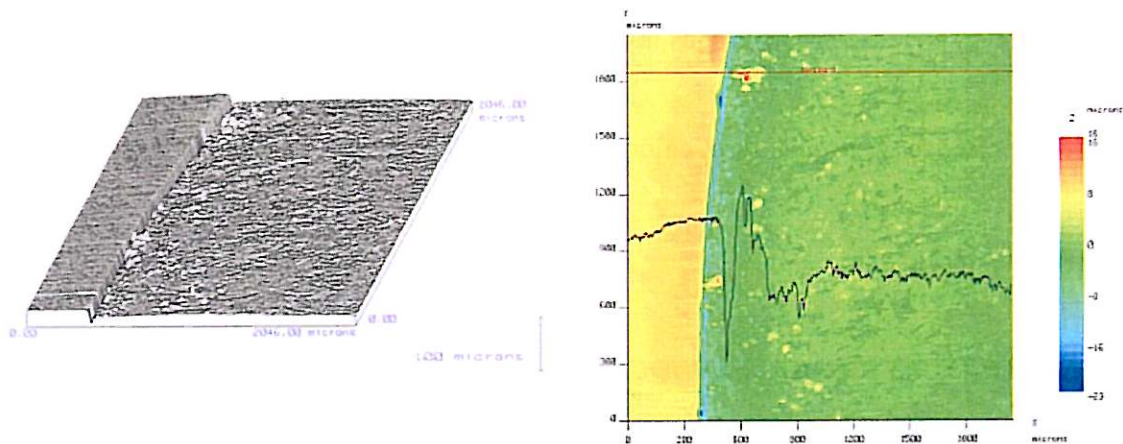
Figure IV.B-10 : Cartographies topographiques (MMB) de la surface de l'acier X70 décapée, après 2 semaines de CL et 2 semaines sous PC ( -1125\text{mV/ECS} ), dans l'eau carbonatée désaérée – pas de mesure = 2\ \mu\text{m} , S = 4,194\text{mm}^2 .
