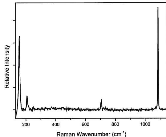
Figure IV.A-7 : Spectre Raman ex-situ d'un cristal d'aragonite isolé, formé à la surface de l'acier X70 après 14 jours de CL et 14 jours sous PC ( -1125\text{mV/ECS} ) dans l'eau siliceuse aérée.
