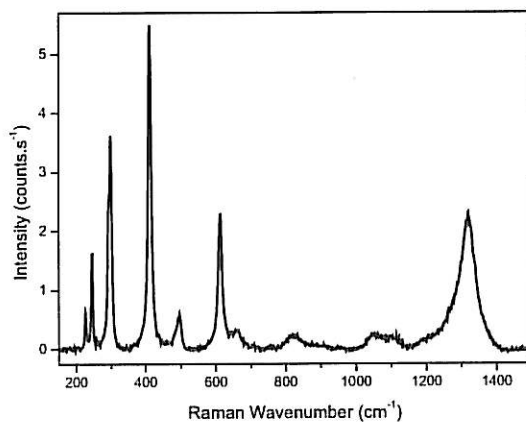
Figure II.A-3 : Spectre Raman d'hématite \alpha-Fe_2O_3 200s - 0,1mW
