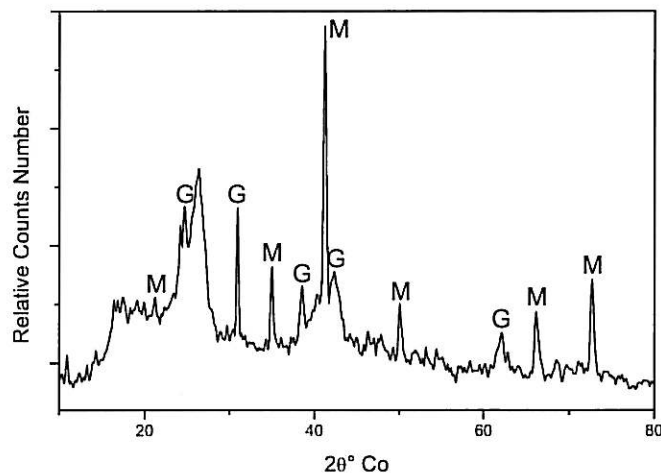
Figure V.B-7 : Diffractogramme X des produits de corrosion prélevés sous le décollement ouvert et conservés dans l'acétone. Saint Saturnin – CL (M : magnétite, G : goethite)
