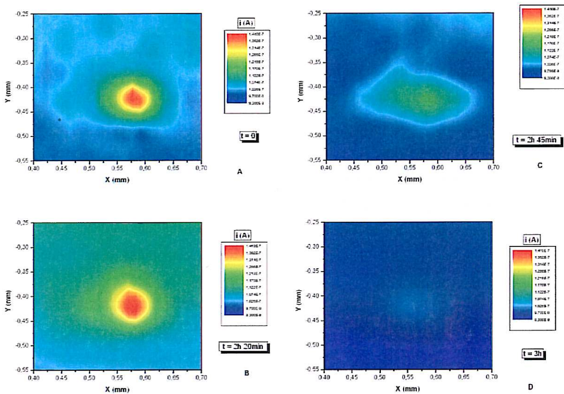
Figure I.C-6 : Images SECM de l'acier X70 dans 50\text{mmol.l}^{-1} de KI, V_x=100\mu\text{m/s} – \Delta y=20\mu\text{m} – E_{\text{Tip}}=200\text{mV/ESS} – substrat non polarisé
