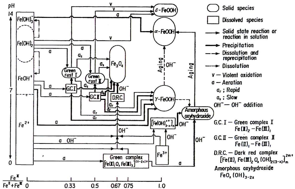
Figure III.D-1 : Diagramme schématique des procédés de formation et d'évolution des oxydes et oxyhydroxydes de fer intermédiaires en solution aqueuse à température ambiante [20].
