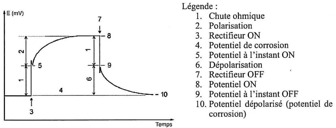
Figure II.C-1 : Diagramme de polarisation cathodique
