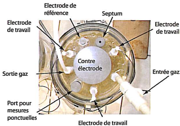
Figure IV.B-2 : Couvercle de la cellule électrochimique classique
