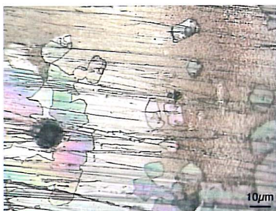
Figure II.B-12 : Photo optique ex-situ de la surface de l'acier X70, après 28 jours sous PC (-1125mV/ECS) dans l'eau siliceuse aérée, et après décollement de la couche formée.
