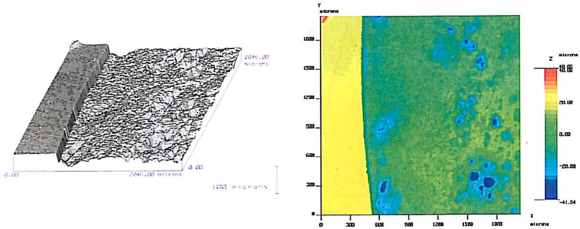
Figure III.A-14 : Cartographies topographiques (MMB) de la surface de l'acier X70 décapée, après 4 semaines de CL dans l'eau bi-carbonatée désaérée pas de mesure = 2 \mu\text{m} , S = 4,194\text{mm}^2 .
