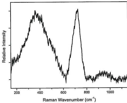
Figure II.A-7 : Spectre Raman ex-situ enregistré sur la face externe de la couche de corrosion formée à la surface de l'acier X70, après 28 jours de CL dans l'eau siliceuse aérée.
