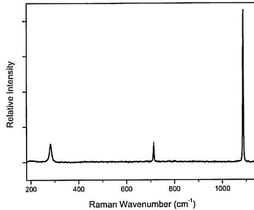
Figure I.A-5 : Spectre Raman in-situ enregistré sur un petit cristal, à la surface de l'acier X70, après 90 minutes de CL (-659mV/ECS), dans l'eau bi-carbonatée désaérée saturée en calcite.
