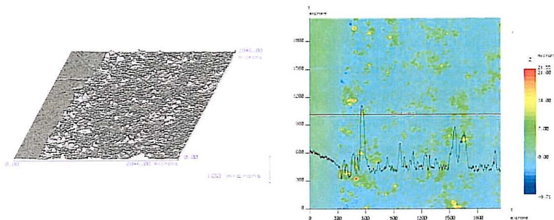
Figure III.B-8 : Cartographies topographiques de la surface de l'acier X70 décapée, après 4 semaines sous PC ( -1125\text{mV/ECS} ) dans l'eau bi-carbonatée désaérée - pas de mesure = 2\mu\text{m} , S = 4,194\text{mm}^2 .
