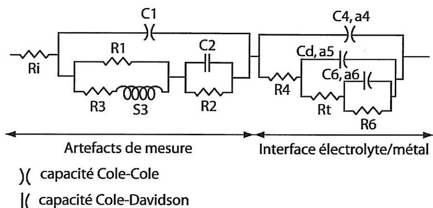
Figure V.C-1 : Circuit électrique équivalent [12]
