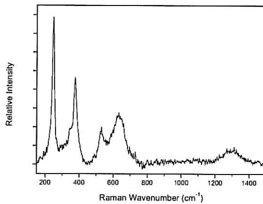
Figure V.B-3 : Spectre Raman ex-situ, enregistré sur des cristaux oranges. Saint Saturnin – PC permanente.
