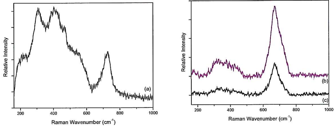
Figure II.A-13 : Spectres Raman ex-situ enregistrés sur une piqûre observée après 28 de CL dans l'eau siliceuse aérée (Figure II.A-12) (a) Centre de la piqûre 1. (b) Zone circulaire intermédiaire 2 (mauve). (c) Zone circulaire externe 3 (claire).
