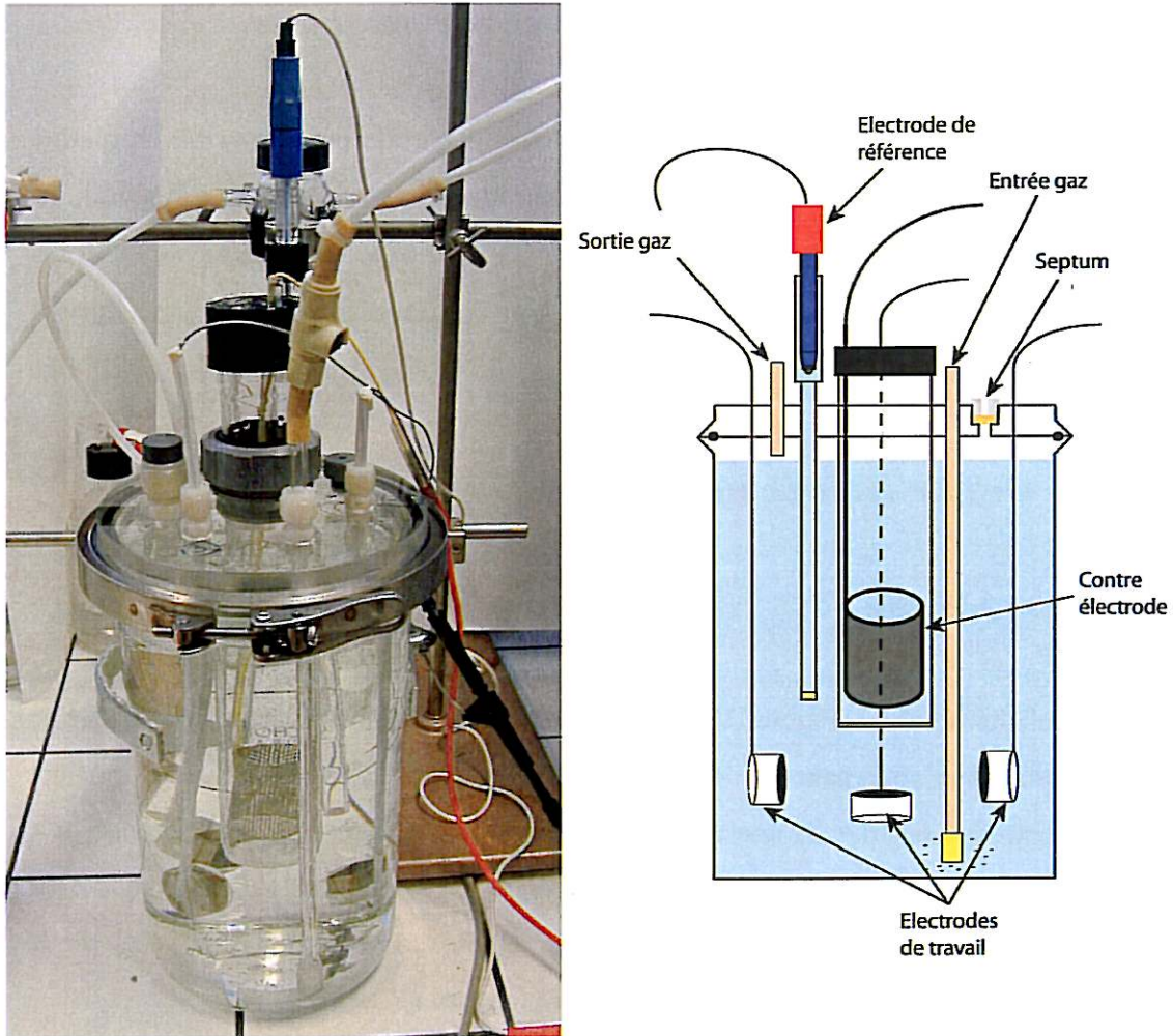
Figure IV.B-1 : Cellule électrochimique classique
