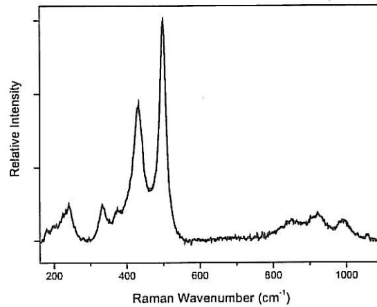
Figure I.A-2 : Spectre Raman in-situ caractéristique de la rouille verte, enregistré après 1 jour sous PC ( -925\text{mV/ECS} ) à la surface de l'acier X70, dans l'eau siliceuse aérée.
