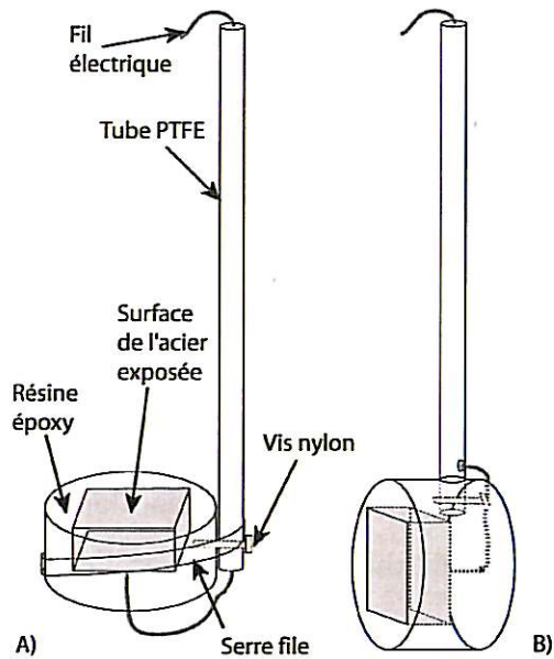
Figure IV.B-3 : Échantillons montés sur les portes-échantillon associés à la cellule électrochimique classique. A) position horizontale, B) position verticale
