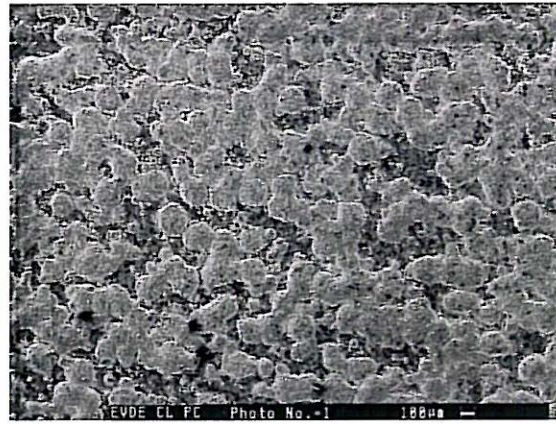
Figure IV.B-5 : Image MEB de la surface de l'acier X70, après 14 jours de CL et 14 jours sous PC (-1125mV/ECS) dans l'eau bi-carbonatée désaérée.
