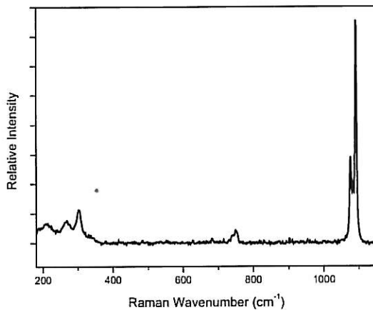
Figure I.A-4 : Spectre Raman in-situ enregistré sur un petit cristal, à la surface de l'acier X70, après 4 heures de CL (-603mV/ECS), dans l'eau bi-carbonatée désaérée saturée en calcite.
