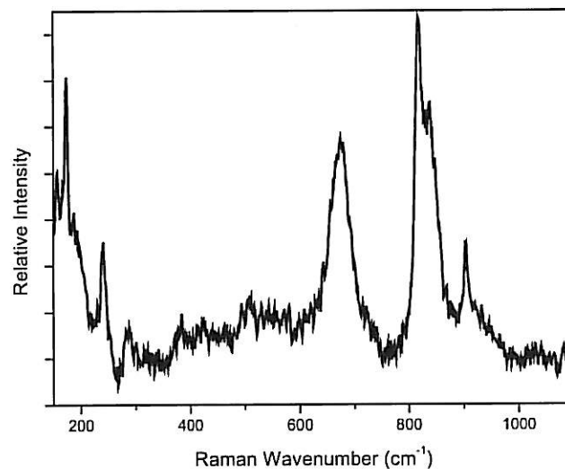
Figure I.C-5 : Spectre Raman in-situ enregistré sur une amorce de piqûre à la surface du fer, après 5 jours sous PC (-1075mV/ECS) dans l'eau siliceuse aérée.
