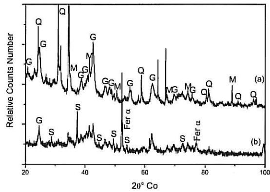
Figure V.B-13 : Diffractogrammes X du défaut lacunaire après un 1 er et un 2 ème grattage. Brech – CL (Q : quartz, G : goethite, M : magnétite, S : sidérite).
