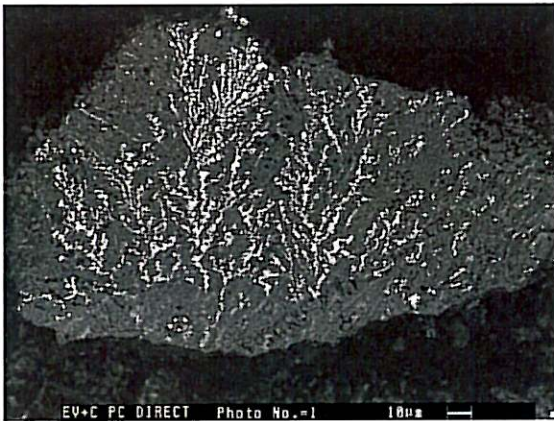
Figure III.B-6 : Image MEB de la face interne de la couche de corrosion formée à la surface de l'acier X70, après 28 jours sous PC (-1125mV/ECS) dans l'eau bi-carbonatée désaérée saturée en calcite.
