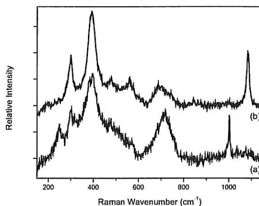
Figure V.B-9 : Spectre Raman ex-situ, enregistré (a) sur la face interne d'une couche grise, (b) sur un cristal noir. Compiègne – PC permanente
