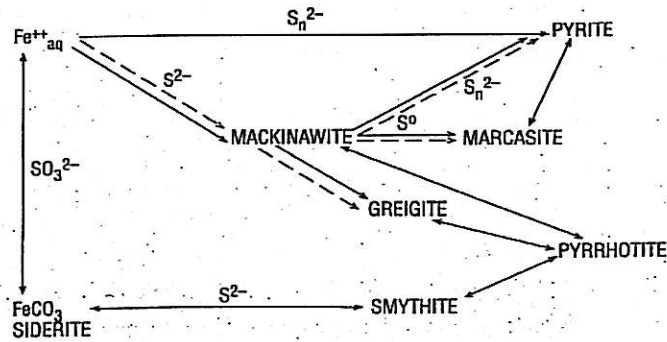
Figure III.D-4 : Transformation des sulfures de fer II formés par corrosion sur les conduites enterrées [42]. Pyrite FeS_2 , Mackinawite FeS , Marcasite FeS_2 , Greigite Fe_3S_4 , Smythite Fe_9S_{11} , Pyrrhotite Fe_{1-x}S .
