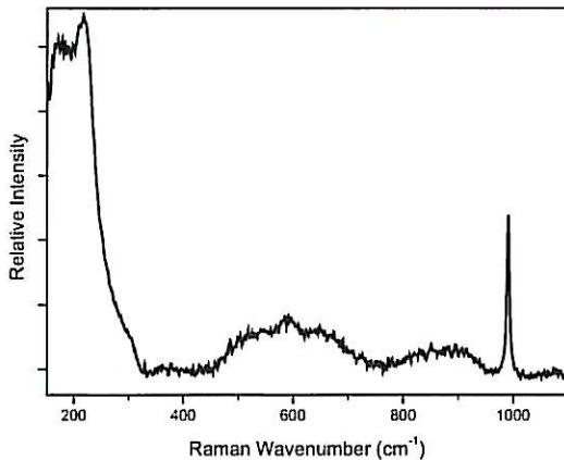
Figure III.A-6 : Spectre Raman ex-situ enregistré sur une zone bleue claire au contact de l'acier X70, après 28 jours de CL dans l'eau bi-carbonatée désaérée saturée en calcite (à travers le flacon hermétique en verre).
