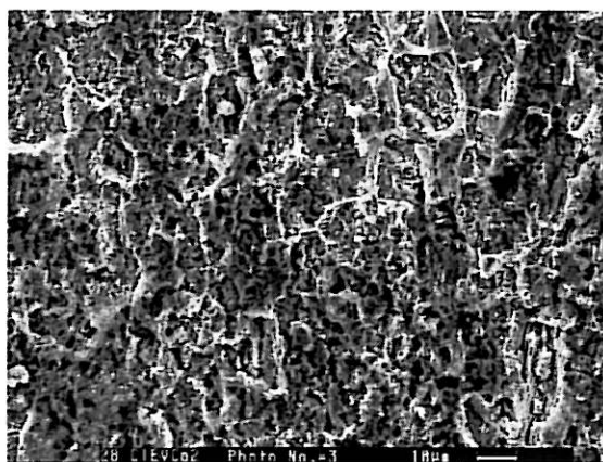
Figure III.A-13 : Image MEB de la surface de l'acier, après 28 jours de CL dans l'eau carbonatée désaérée saturée en calcite.
