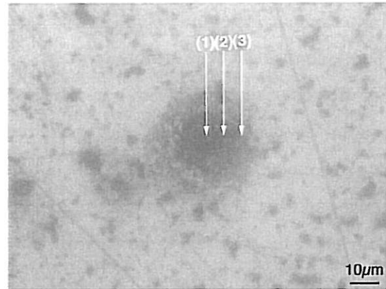
Figure I.C-2 : Photo optique in-situ d'une amorce de corrosion observée sur la surface de l'acier X70 après 3 heures de CL ( -455\text{mV}/\text{ECS} ) dans l'eau siliceuse aérée.
