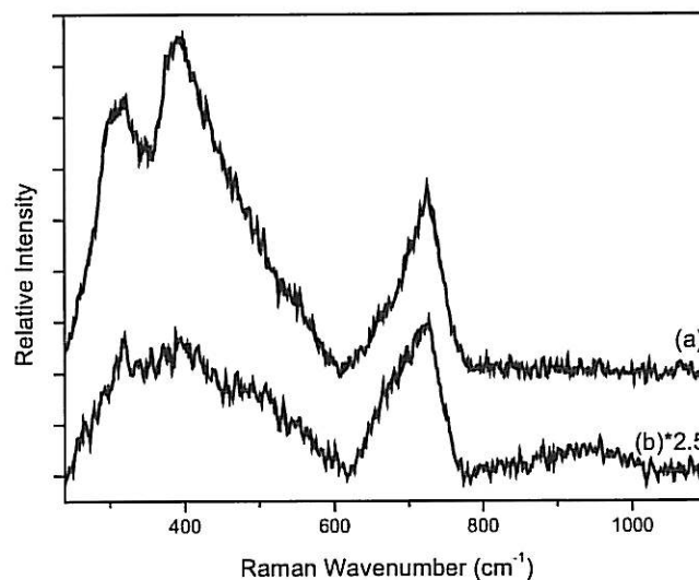
Figure IV.A-3 : Spectres Raman ex situ (a) d'un cristal rectangulaire, (b) de ferrihydrite particulaire noire après 2 jours de CL (-444mV/ECS à -564mV/ECS) et 5 jours sous PC (-1075mV/ECS) dans l'eau siliceuse aérée.
