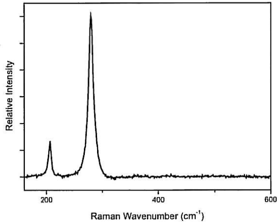
Figure I.C-1 : Spectre Raman in-situ enregistré sur une amorce de piqûre observée à la surface de l'acier X70 après 10 minutes sous PC ( -1075\text{mV}/\text{ECS} ) dans l'eau bicarbonatée désaérée.
