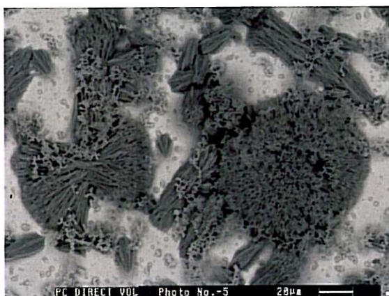
Figure II.B-3 : Image MEB de la surface de l'acier X70, après 16 jours sous PC (-925mV/ECS) dans l'eau siliceuse aérée, dans la cellule spectro-électrochimique.
