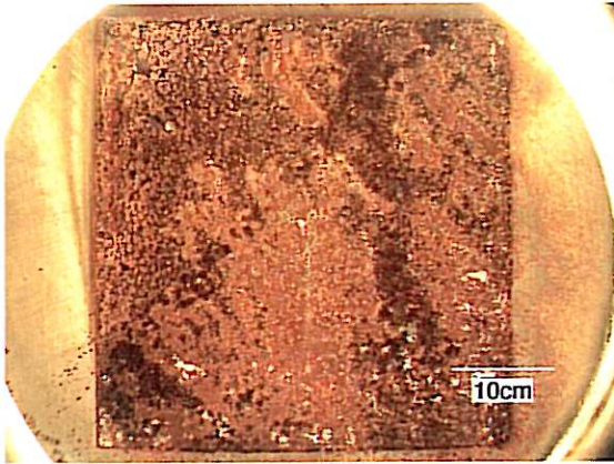
Figure IV.A-4 : Photo optique de la surface de l'acier X70, après 14 jours de CL et 14 jours sous PC ( -1125\text{mV/ECS} ) dans l'eau siliceuse aérée.
