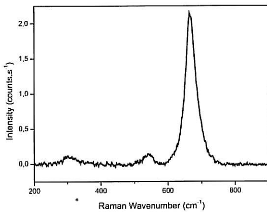
Figure II.A-1 : Spectre Raman de magnétite Fe_3O_4 temps d'acquisition : 250s - puissance du laser : 0,1mW.
