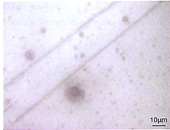
Figure I.B-2 : Photo optique in-situ de la surface de l'acier X70, après 20 heures sous PC (-925mV/ECS), dans l'eau siliceuse aérée.
