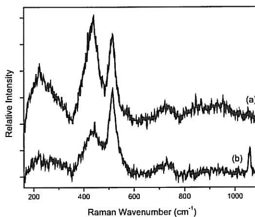
Figure IV.B-2 : Spectres Raman ex-situ enregistrés sur des petits cristaux, formés sur la surface de l'acier X70 après 1 jour de CL, 5 jours sous PC ( -1025\text{mV/ECS} ) et 2 jours de CL, dans l'eau bi-carbonatée désaérée saturée en calcite.
