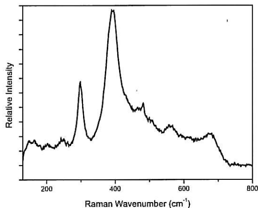
Figure III.A-3 : Spectre Raman in-situ enregistré sur une zone sombre à la surface de l'acier X70, après 26 heures de CL ( \approx -655\text{mV/ECS} ) dans une solution bi-carbonatée désaérée synthétique.
