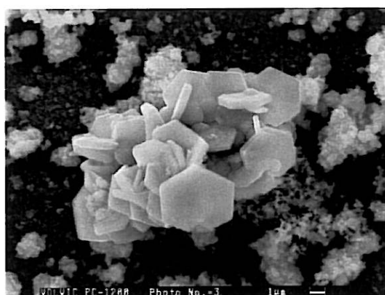
Figure IV.A-2 : Image MEB de produits de corrosion hexagonaux formés à la surface de l'acier X70, après 3 jours de CL ( -455 à -569\text{mV/ECS} ) et 11 jours sous PC ( -783\text{mV/ECS} ) dans l'eau siliceuse aérée.
