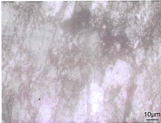
Figure I.B-3 : Photo optique in-situ de la surface de l'acier X70, après 24 heures de CL (-675mV/ECS), dans l'eau bi-carbonatée désaérée saturée en calcite.
