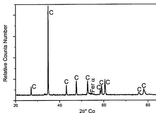
Figure III.B-5 : Diffractogramme X de la couche de corrosion formée à la surface de l'acier X70, après 28 jours sous PC ( -1125\text{mV/ECS} ) dans l'eau bi-carbonatée désaérée (C : calcite).
