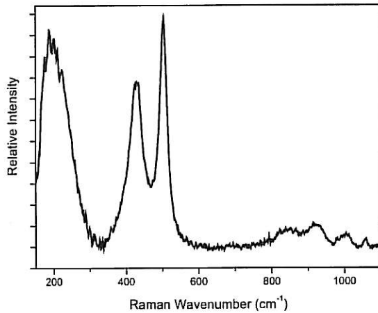
Figure I.A-1 : Spectre Raman in-situ caractéristique de la rouille verte pulvérulente, enregistré après 2 heures en CL ( -463\text{mV/ECS} ) à la surface de l'acier X70, dans l'eau siliceuse aérée.
