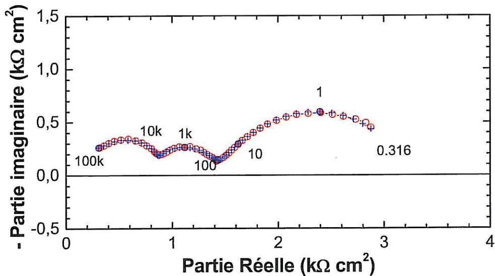
Figure II.B-17 : Diagrammes d'impédances de l'acier X70 polarisé cathodiquement à -1125\text{mV/ECS} , en fonction du temps d'immersion dans l'eau siliceuse aérée, rond : expérimental – croix : modèle électrique
