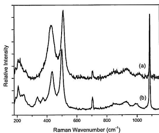
Figure IV.B-1 : Spectres Raman in-situ enregistrés sur la surface de l'acier X70, au cours de la même expérience, après (a) 25 heures de CL ( \approx -575\text{mV/ECS} ), (b) 27 heures de CL et 90 minutes sous PC ( -1025\text{mV/ECS} ), dans l'eau bi-carbonatée désaérée saturée en calcite.
