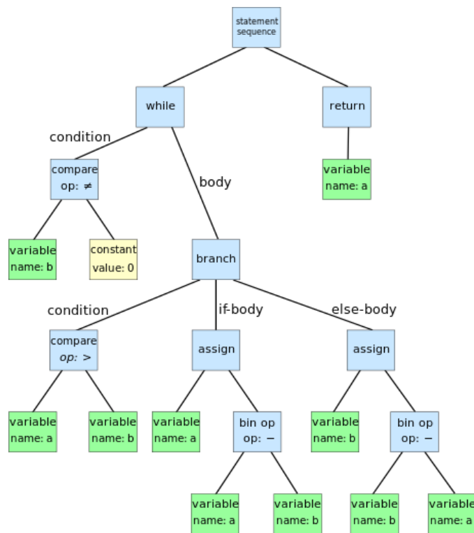
Figure. 12.2 – AST de l'algorithme d'Euclide pour le calcul de PGCD
