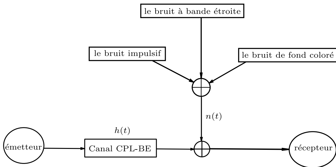
FIGURE 2.4: Bruit sur le canal CPL-BE
