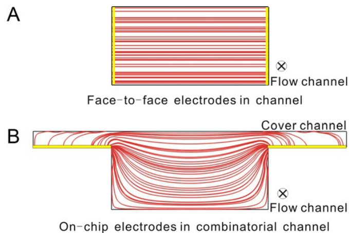
FIGURE 1.16 – Distribution du champ électrique dans un canal fermé (lignes isopotentiellles), pour les deux configurations d'électrodes. (A) Electrodes parallèles. (B) Electrodes intégrées sur le microcanal en PDMS [58].
