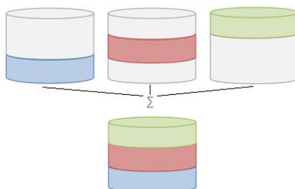
Figure 29 : Clés énumérables
