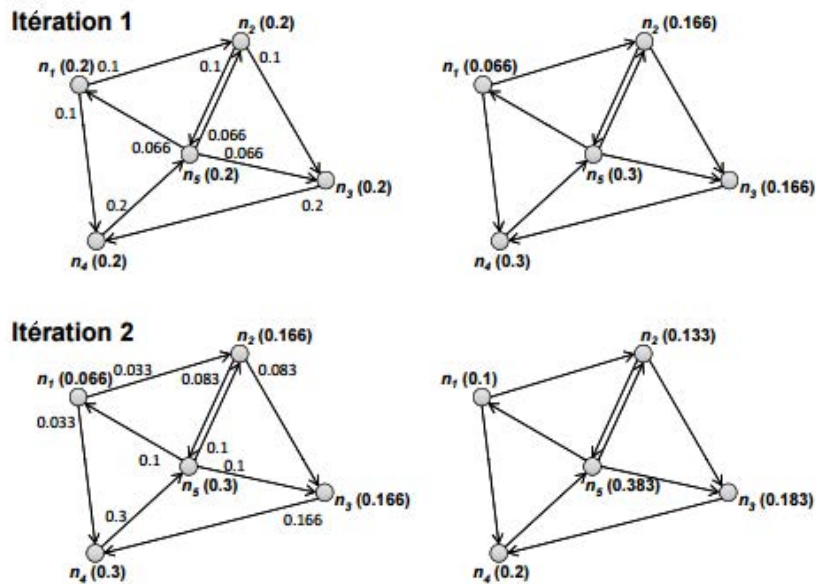
Figure 20 : Algorithme PR
