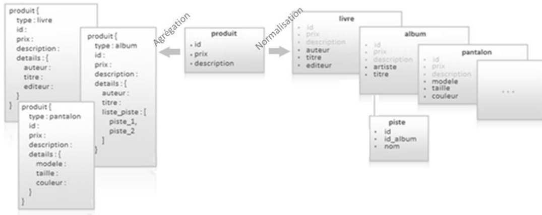
Figure 26 : Agrégation d'entités
