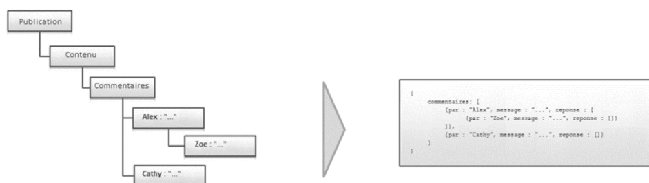
Figure 35 : Agrégation d'arborescence
