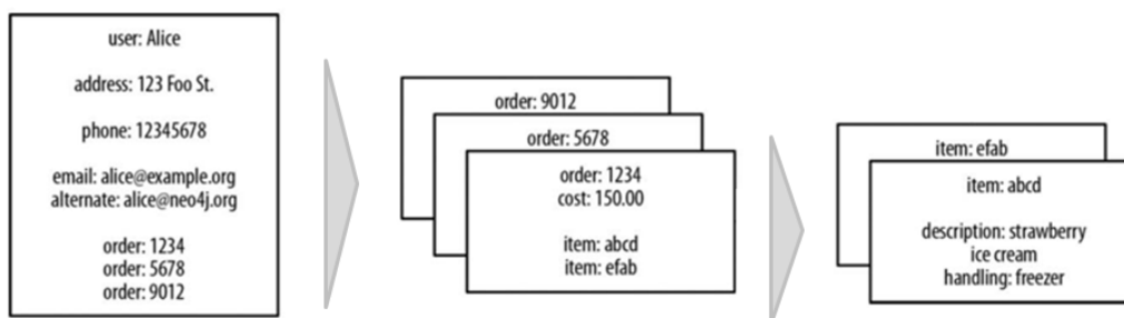
Figure 69 : Références entre documents
