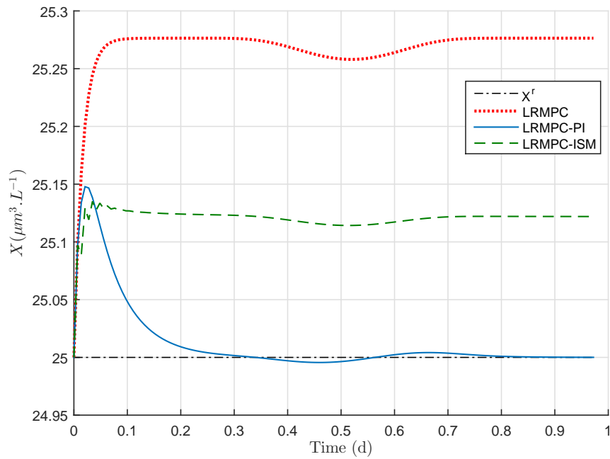
FIGURE 1.11 – Évolution temporelle de la concentration en biomasse.
