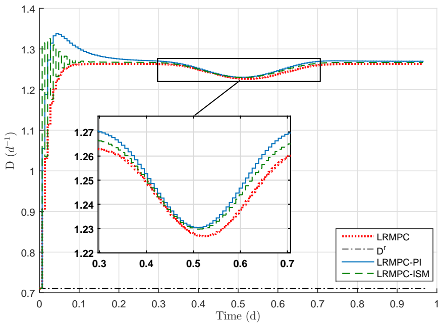
FIGURE 1.12 – Évolution temporelle du taux de dilution.
