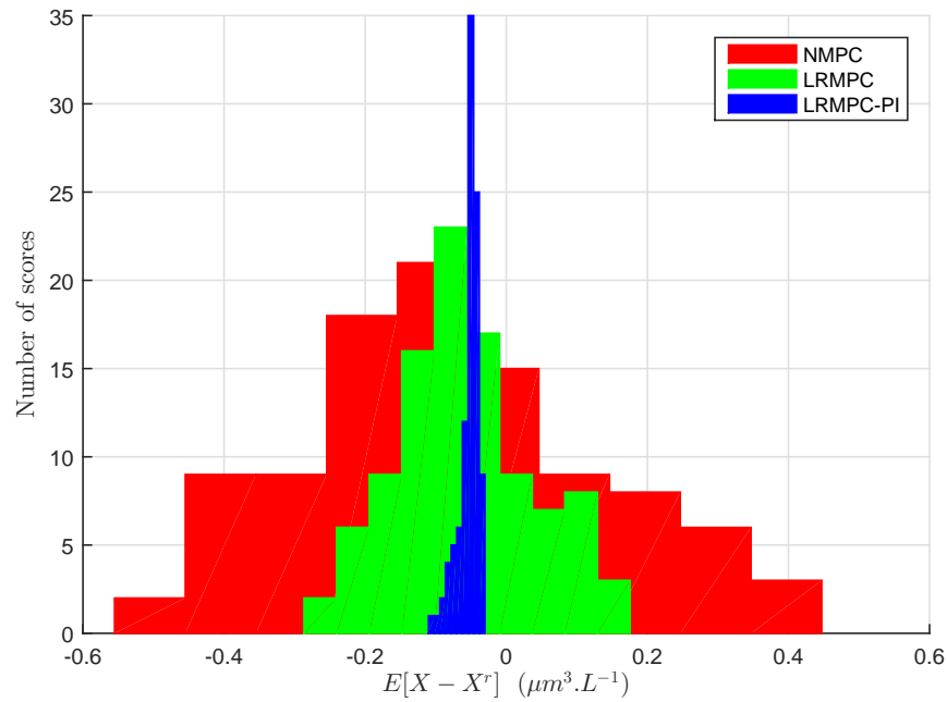
FIGURE 1.10 – Histogramme de la moyenne de l’erreur de poursuite pour une variation aléatoire non-corrélée de tous les paramètres (Monte-Carlo).
