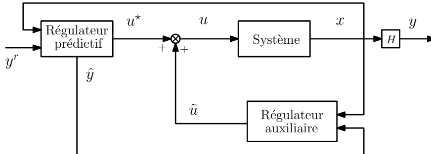
FIGURE 1.6 – Schéma de la stratégie de commande hiérarchisée.
