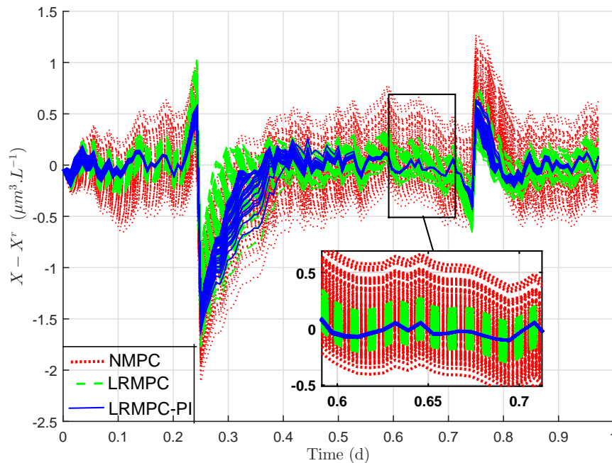
FIGURE 1.9 – Évolution temporelle de l'erreur de poursuite pour une variation aléatoire non-corrélée de tous les paramètres (Monte-Carlo).
