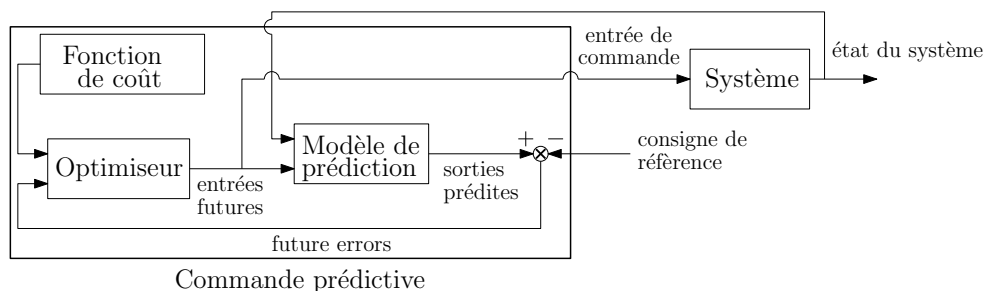
FIGURE 1.1 – Schéma de la structure générale de la commande prédictive.
