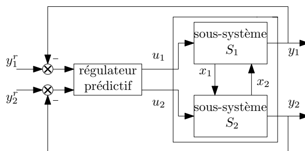
FIGURE 1.2 – Architecture de la commande prédictive centralisée [34].
