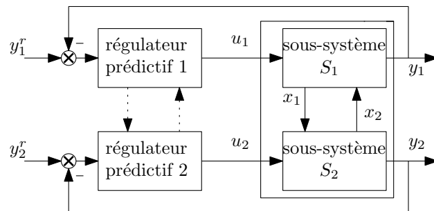
FIGURE 1.4 – Architecture de la commande prédictive distribuée [34].
