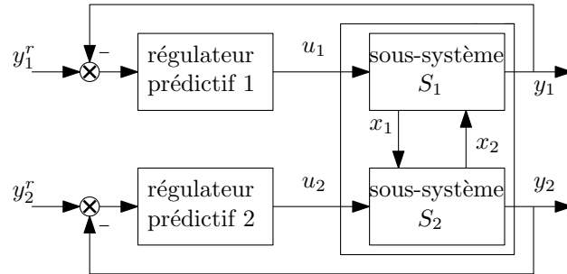
FIGURE 1.3 – Architecture de la commande prédictive décentralisée [34].
