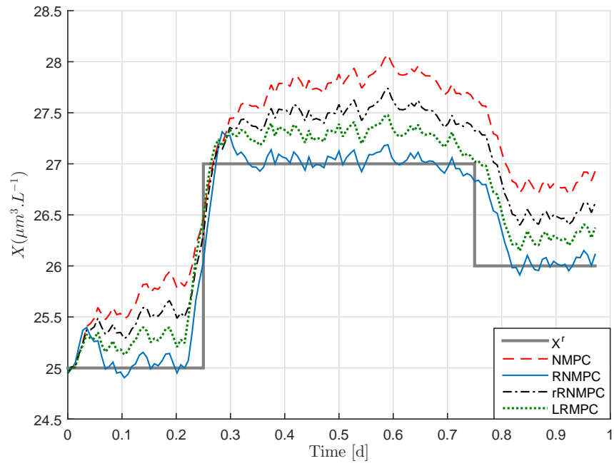
FIGURE 1.7 – Évolution temporelle de la concentration en biomasse.
