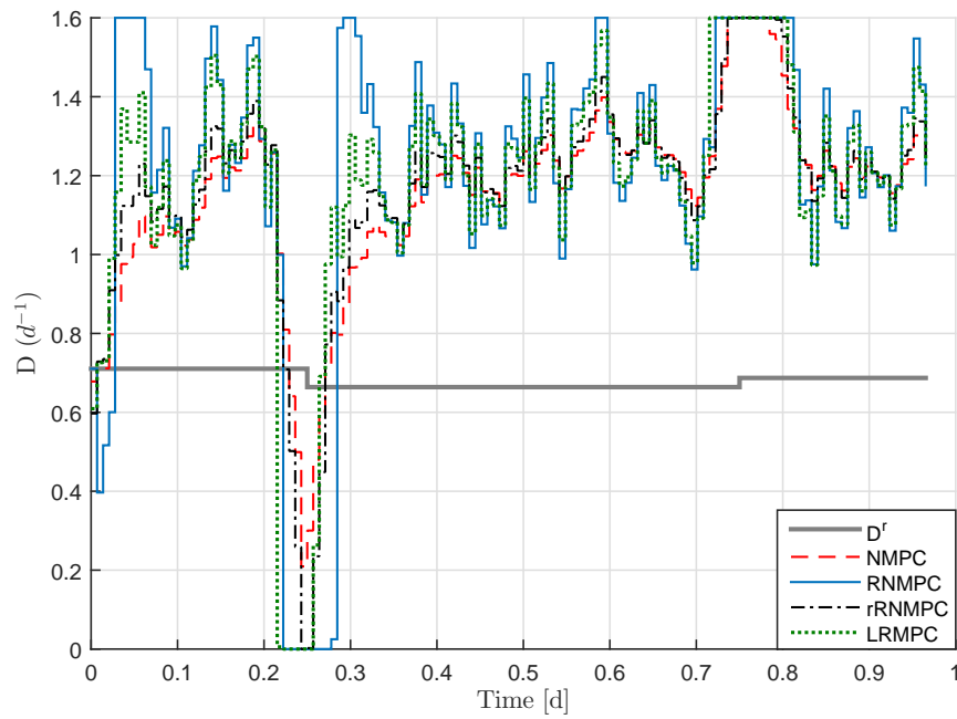
FIGURE 1.8 – Évolution temporelle du taux de dilution.
