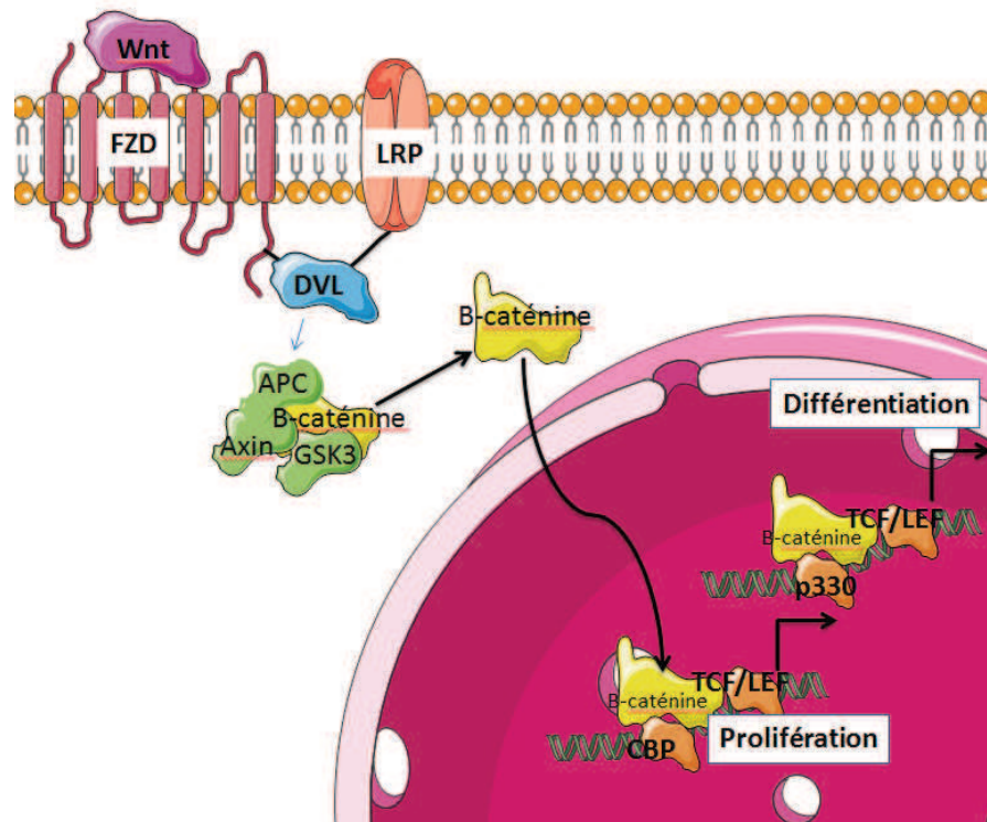
Figure 12 : Schéma simplifié de la voie Wnt/β-caténine
