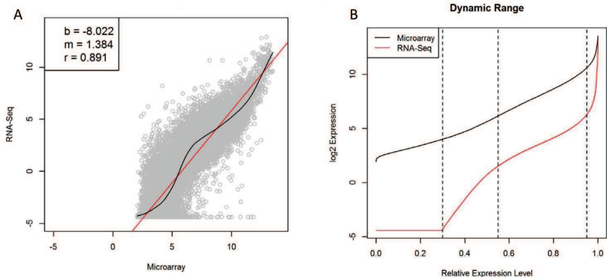
Figure 15 : Comparaison des données de puce et séquençage.
