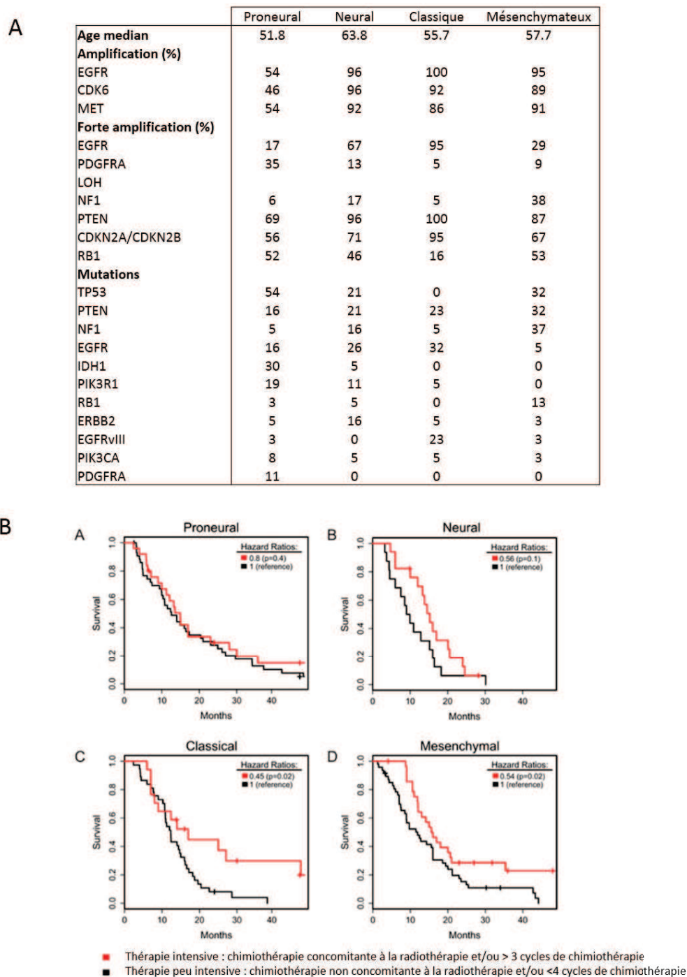
Figure 8 : Classification de Verhaak
