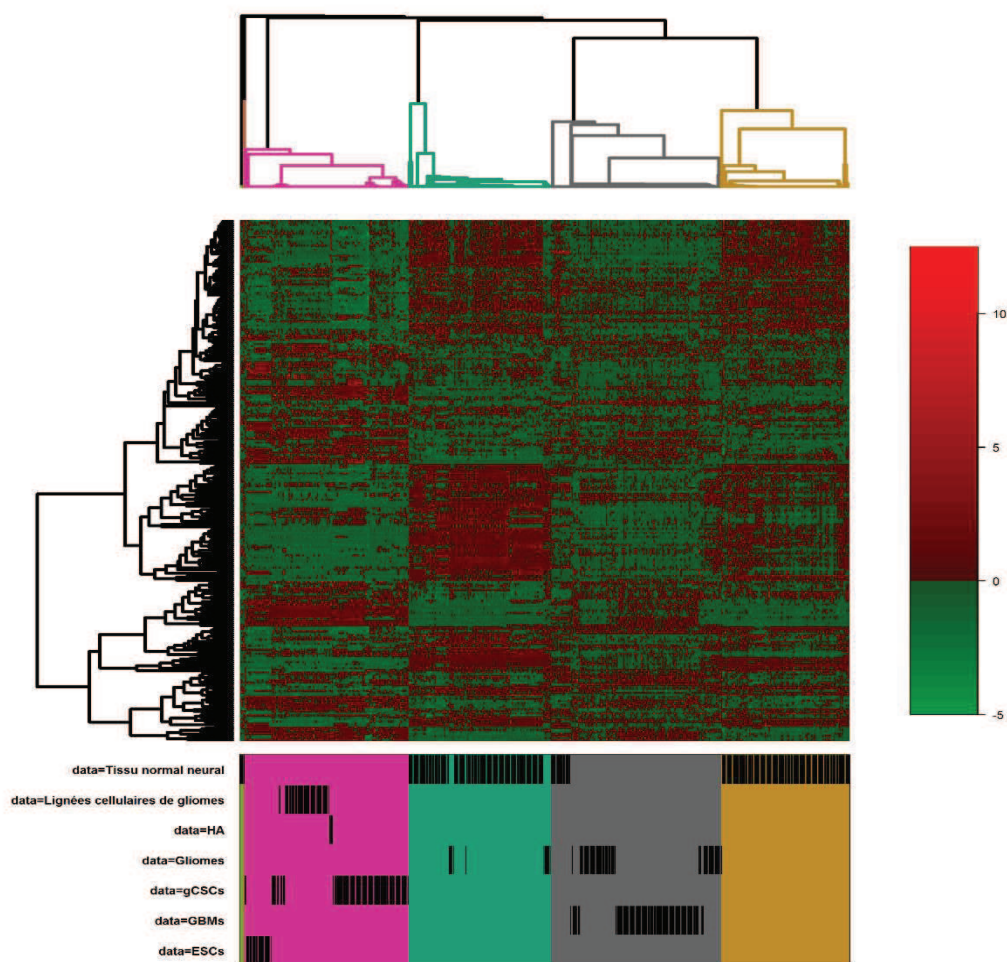
Figure 41 : Classification de l'ensemble des échantillons à partir des gènes de la toolbox calcium filtrés et visualisation sous forme de heatmap avec les annotations.
