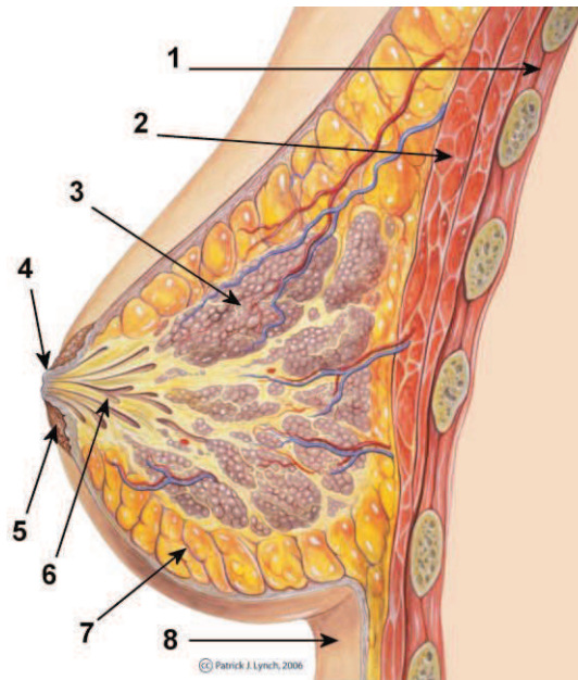
Figure 23 : Schéma anatomique du sein.
