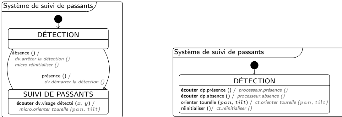
(a) Comportement des fragments du système hébergés sur le processeur (à gauche) et le micro-contrôleur (à droite) avant injection dans les conteneurs
