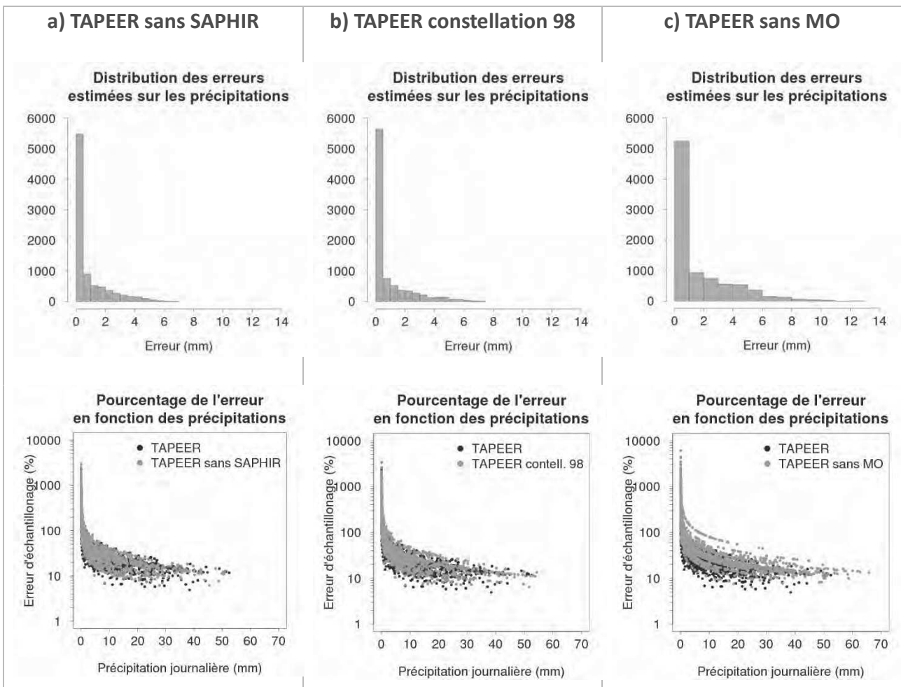
Figure 6. 15 : Distribution des erreurs estimées par TAPEER en mm (panneaux supérieurs) et représentation de l'erreur (en pourcentage des précipitations estimées) en fonction des précipitations (panneaux inférieurs) pour les différentes constellations dégradées.
