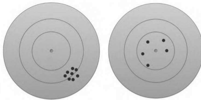
Figure 6. 7 : Illustration des différences entre le biais (a) et l'incertitude (b) d'une estimation, par analogie avec une cible (d'après Chambon 2011). Le centre de la cible en rouge représente la valeur réelle d'une variable et les points noirs ses estimations. Dans le cas de la figure a le biais est plus grand que l'incertitude, la figure b présente le cas contraire.
