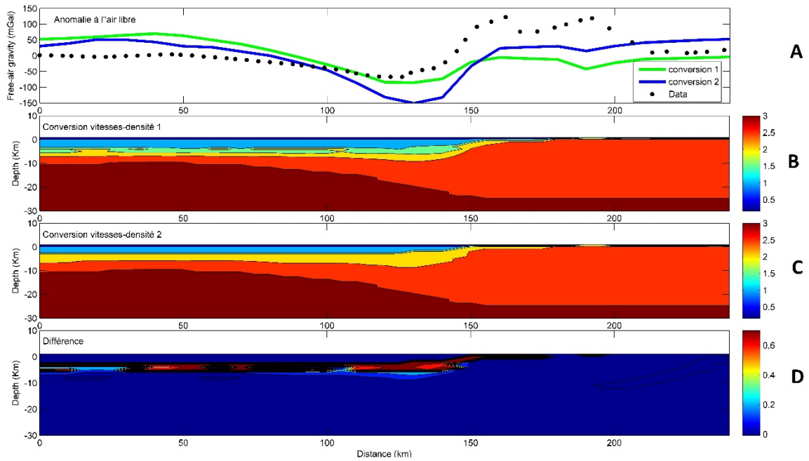
Figure 4-3. Résultats de la conversion vitesse-densité du profil de Kabylie. Modèle 1 : utilisant les lois différentes pour chaque formations (sédiments, croûte et manteau) Hamilton (1978), Carlson & Herrick (1990) et Birch (1961). Modèle 2 : utilisant la loi de Birch (1961). A : anomalie à l'air libre observée et modélisées. B : modèle de densité issu de la conversion 1; C : modèle de densité issu de la conversion 2; D : différences entre les deux modèles de conversion.
