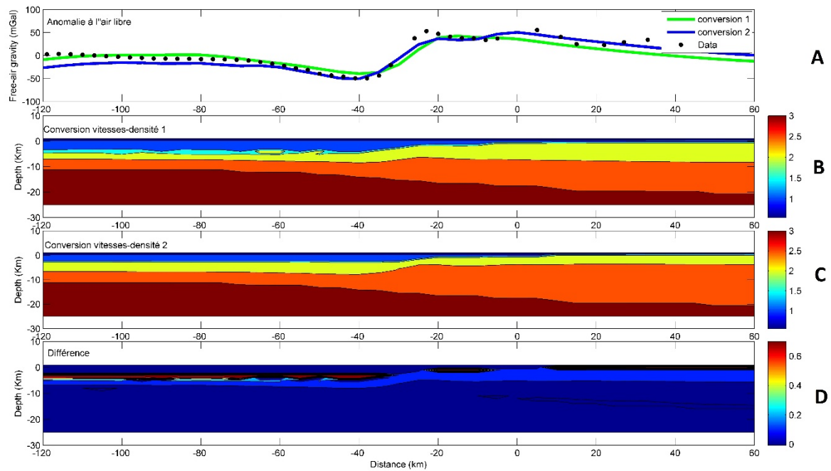
Figure 4-4. Résultats de la conversion vitesse-densité du profil de Tipaza. Modèle 1 : utilisant les lois différentes pour chaque formations (sédiments, croute et manteau) Hamilton (1978), Carlson & Herrick (1990) et Birch (1961). Modèle 2 : utilisant la loi de Birch (1961). A : anomalie à l'air libre observée et modélisées. B : modèle de densité issu de la conversion 1; C : modèle de densité issu de la conversion 2; D : différences entre les deux modèles de conversion.
