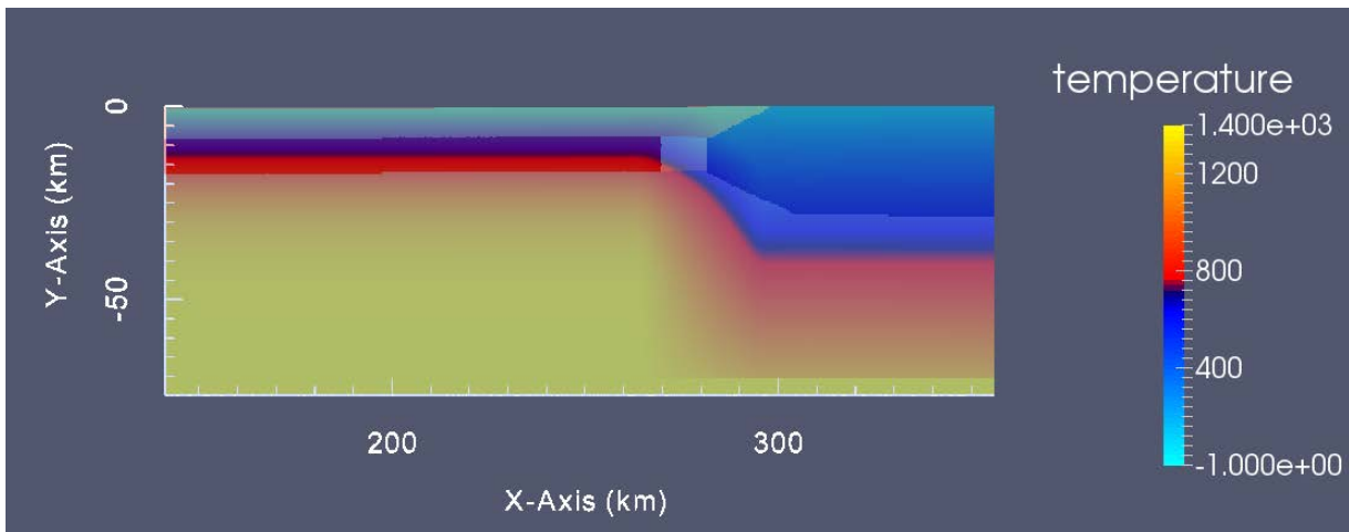
Figure 5-19. Superposition du gradient géothermique avec la géométrie des différentes phases rhéologiques. Contact direct océan-continent (TOC océanique).
