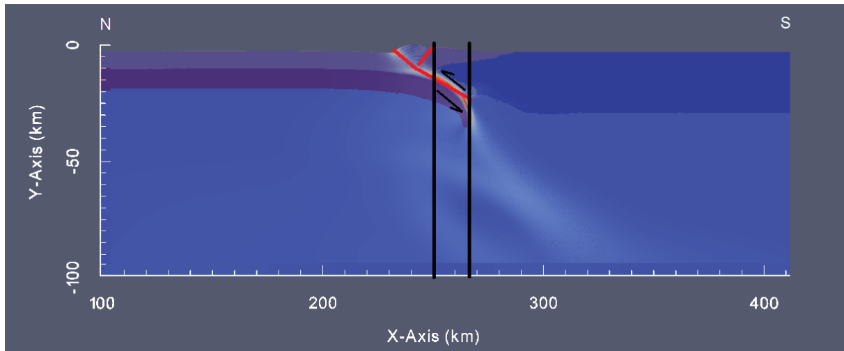
Figure A-4. Taux de déformation du modèle 10 au niveau de la Transition Océan-Continent. Traits noirs : TOC flexurale. Traits rouges : plan de faille supposé. Flèches noirs : sens du cisaillement.
