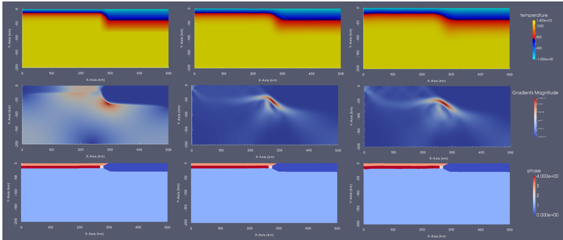
Figure 5-17. Modèle thermomécanique (0-5Ma) avec un gradient géothermique chaud au niveau d'une TOC océanique à contacts verticaux. En haut : gradient géothermique. Au milieu : taux de déformation. En bas : phases rhéologique (rouge : croûte océanique, bleu nuit : croûte continentale, bleu ciel : manteau, blanc : TOC océanique et orange : sédiments). Captures d'image au début (0Ma) au milieu (2,5Ma) et à la fin (5Ma).
