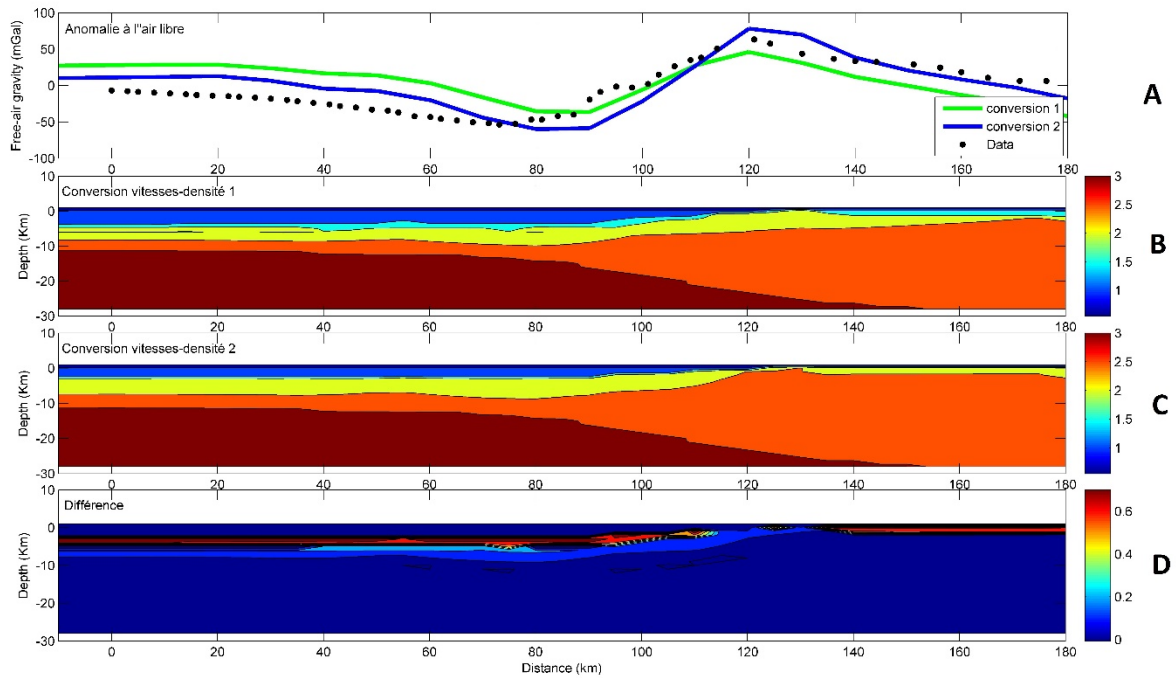
Figure 4-1. Résultats de la conversion vitesse-densité du profil d'Annaba. Modèle 1 : utilisant les lois différentes pour chaque formations (sédiments, croute et manteau) Hamilton (1978), Carlson & Herrick (1990) et Birch (1961). Modèle 2 : utilisant la loi de Birch (1961). A : anomalie à l'air libre observée et modélisées. B : modèle de densité issu de la conversion 1; C : modèle de densité issu de la conversion 2; D : différences entre les deux modèles de conversion.
