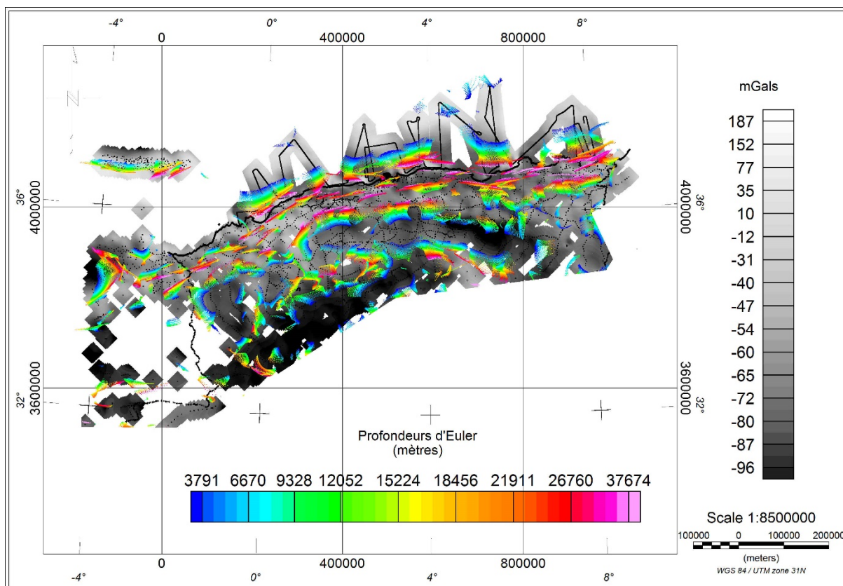
Figure 3-10. Solution d'Euler (fond : carte de la prolongée à 5 km densité 2,67). Structural Index : 0, Windows Size : 10, Tolérance : 5%.
