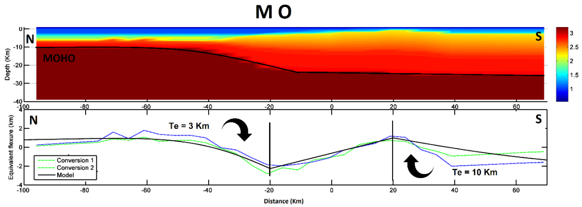
Figure 4-12. Haut : modèle de densité calculé par la conversion des vitesses sismiques en densités avec la loi de Birch (vitesses sismiques d'après Rabia et al. 2014). Bas : modèle de flexion 2-D du profil de Jijel. Les lignes vertes et bleues sont la flexion équivalente calculée à partir des deux différentes conversions vitesse-densité, et la ligne noire est la déflection modélisée. Les deux lignes noires verticales délimitent la zone de transition entre les deux plaques (océanique et continentale) en flexion.
