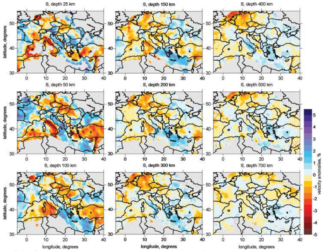
Figure 5-2. Résultats de la tomographie des anomalies de vitesse S dans des sections horizontales (d'après Koullakov et al., 2009).
