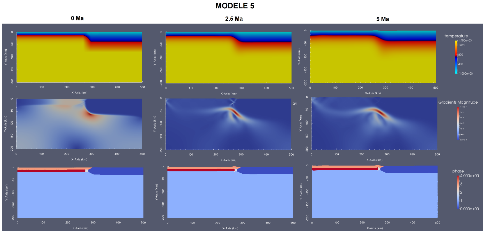
Figure 5-15. Modèle thermomécanique (0-5Ma) avec un gradient géothermique chaud au niveau d'une TOC continentale à contacts verticaux. En haut : gradient géothermique. Au milieu : taux de déformation. En bas : phases rhéologique (rouge : croûte océanique, bleu nuit : croûte continentale, bleu ciel : manteau, blanc : TOC continentale et orange : sédiments). Captures d'image au début (0Ma) au milieu (2,5Ma) et à la fin (5Ma).
