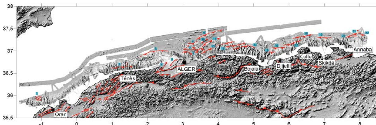
Figure 3-11. Modèle numérique de terrain ombré terre-mer synthétisant les principales structures actives le long de la côte algérienne (d'après Domzig, 2006b).
