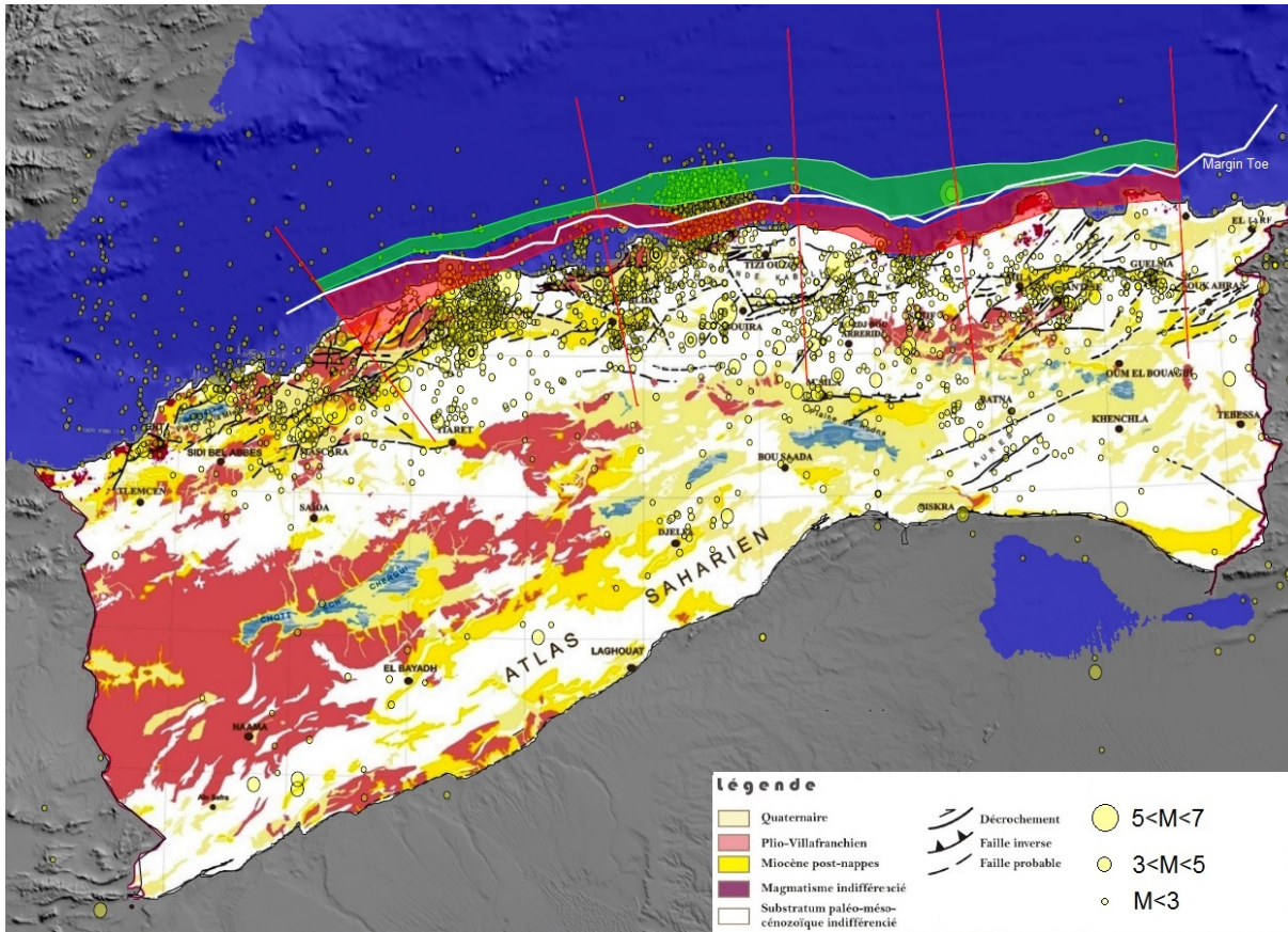
Figure 6-1. Carte sismotectonique du Nord de l'Algérie (CRAAG). En Vert : la TOC d'après les modèles de vitesses. En rouge : la TOC d'après les modèles de flexion. Trait blanc : pied de marge. Traits rouges : profils SPIRAL d'Est en Ouest : Annaba, Jijel, Kabylie, Tipaza et Mostaganem. Source des données sismologique catalogue CRAAG 2013.
