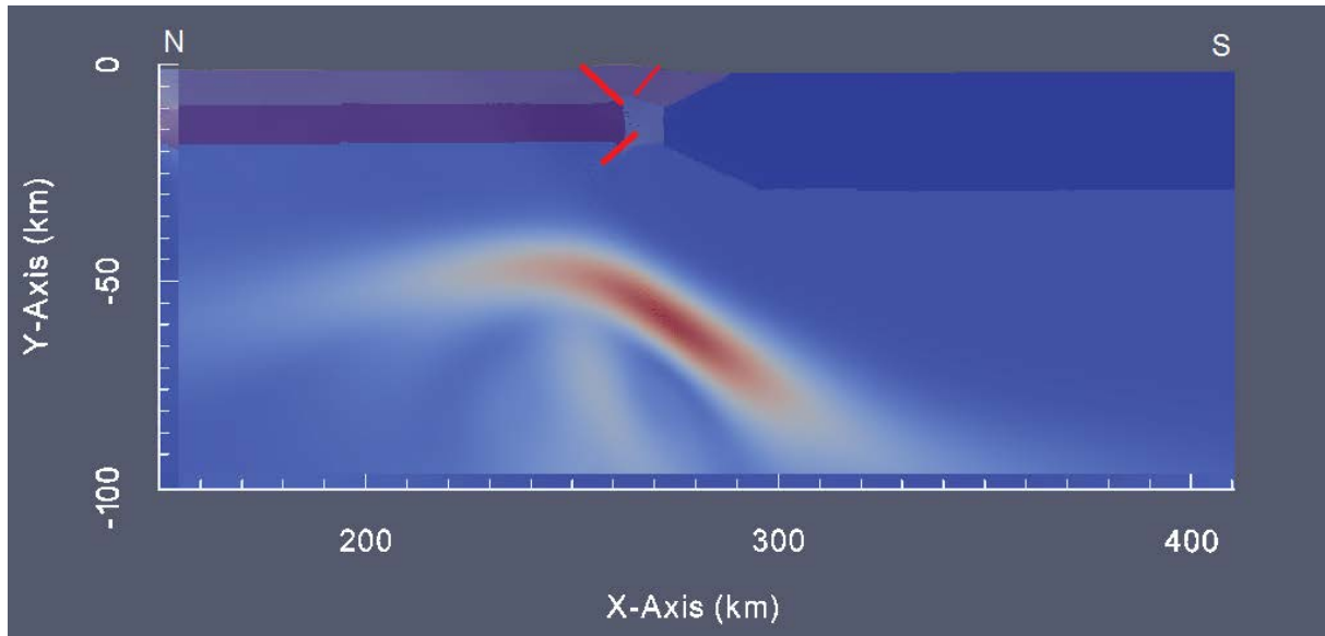
Figure 5-16. Taux de déformation du modèle 5 au niveau de la Transition Océan-Continent. Traits rouges : plans de failles supposés.
