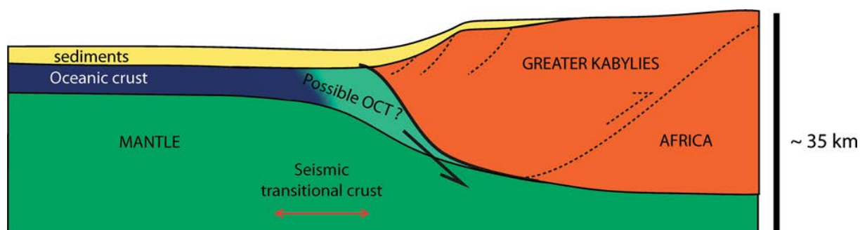
Figure 5-6. Coupe schématique interprétative de la déformation actuelle au niveau de la marge algérienne.
