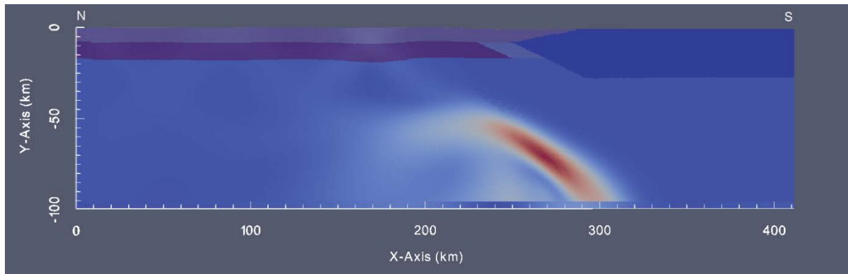
Figure 5-14. Taux de déformation du modèle 4 au niveau de la Transition Océan-Continent.
