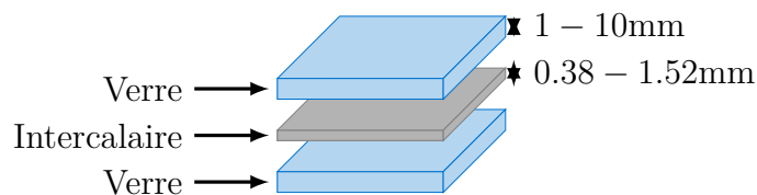
FIGURE 8.1 : Structure d'un verre feuilleté
