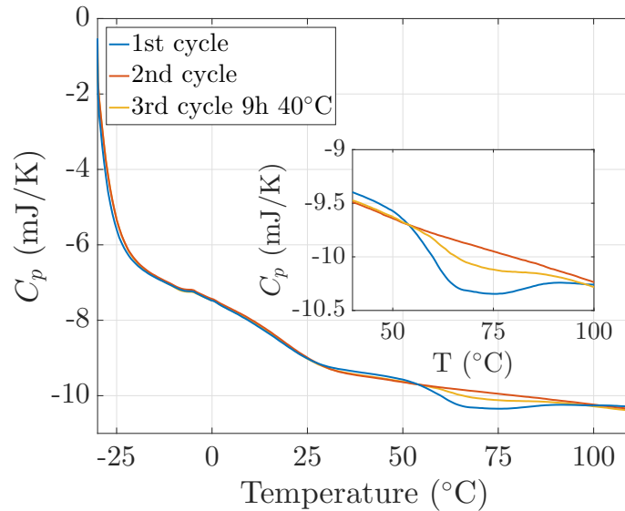
FIGURE 8.5 : La calorimétrie différentielle à balayage permet entre autre de mettre en évidence une transition ordre/désordre autour de 70^{\circ}\text{C} . Cette structure n'est recouverte partiellement qu'après une attente de 9 h à 40^{\circ}\text{C} .
