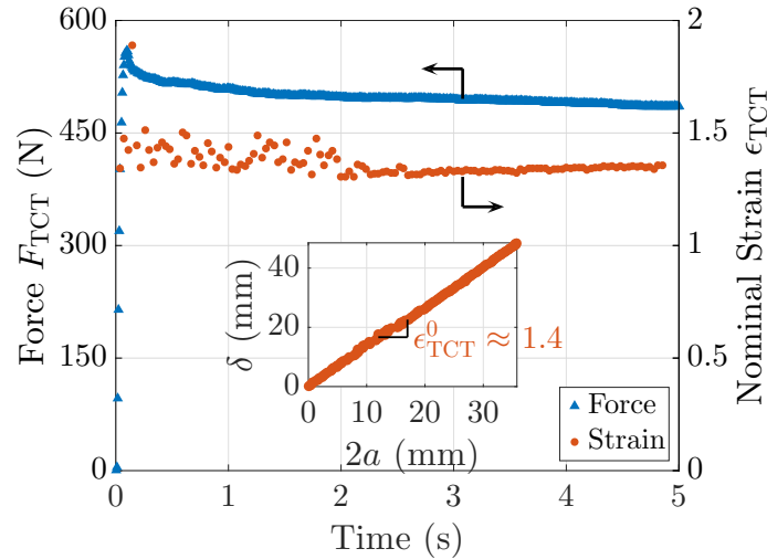
FIGURE 8.8 : Force de délamination et déformation de l'intercalaire sont constants au cours de la délamination stationnaire à 20^\circ\text{C} et 10\text{ mm s}^{-1} .
