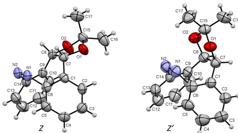
Figure IV-11 : Représentation ORTEP des isomères Z - 121 et Z' - 121 avec numérotation des atomes. Les ellipsoïdes thermiques sont représentés avec une probabilité de 50 % de densité électronique.
