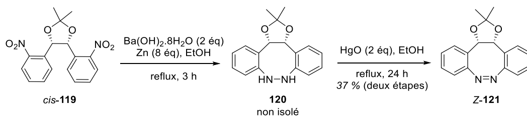
Figure IV-3 : Synth\u00e8se de l'azobenz\u00e8ne Z-121.
