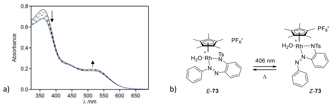
Figure III-11 : a) Spectre d'absorption de 73 dans (\text{CH}_3)_2\text{CO} ( C \sim 10^{-5} M) (courbe noire), évolution au cours de l'irradiation à 406 nm ( P = 9 \text{ mW}\cdot\text{cm}^{-2} , impulsions de 5 s) (courbes pointillées), et état photostationnaire (courbe bleue). b) Processus de photo-isomérisation proposé pour le composé 73 .
