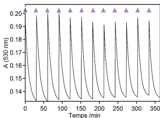
Figure II-22 : Résistance à la fatigue du complexe 37 dans \text{CH}_3\text{CN} ( C = 60 \mu\text{M} ) au cours de cycles d'irradiation à 406 nm et retour thermique dans l'obscurité à 25^\circ\text{C} . Les triangles montrent les impulsions lumineuses.
