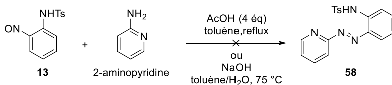
Schéma III-5 : Tentatives de synthèse du composé 58 .
