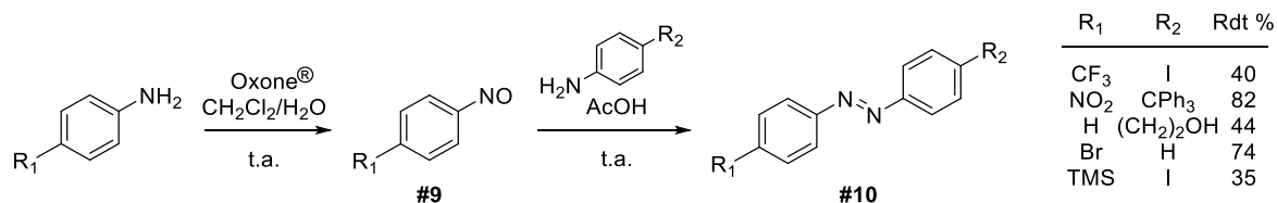
Figure I-7 : Synthèse de nitrosobenzènes et d'azobenzènes par la réaction de Mills.
