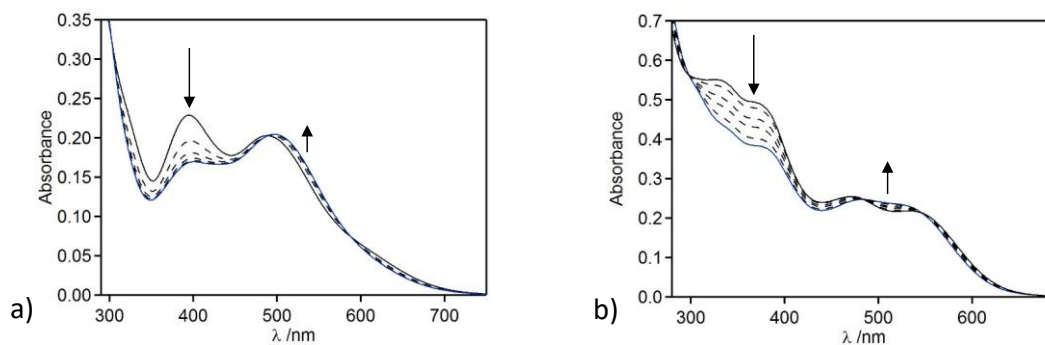
Figure III-5 : Spectres d'absorption dans \text{CH}_3\text{CN} des composés 65 (a) et 69 (b) ( C \sim 10^{-5} M) (courbes noires), évolution au cours de l'irradiation à 406 nm ( P = 9 \text{ mW}\cdot\text{cm}^{-2} , impulsions de 10 s) (courbes pointillées), et état photostationnaire (courbes bleues).
