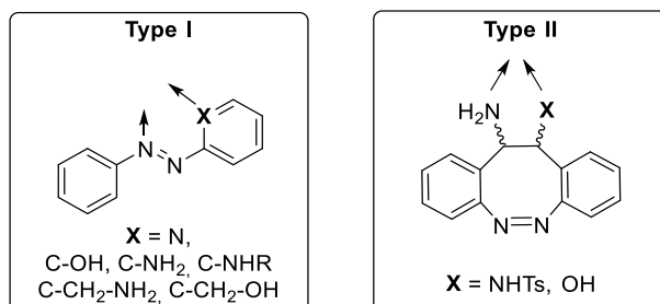
Figure I-13 : Structure des ligands cibles de type I et II.
