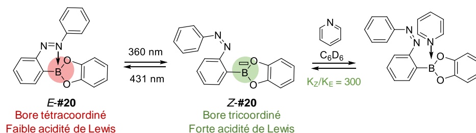
Schéma I-16 : Contrôle du caractère acide de Lewis d'un catecholborane par photo-isomérisation d'un azobenzène.
