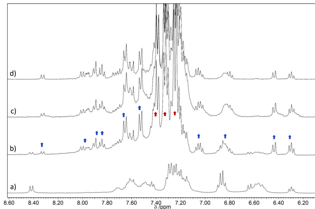
Figure A-5 : Portion du spectre RMN ^1\text{H} de Z-91 dans \text{CD}_3\text{CN} ( C = 4,8 \text{ mM} ) avant irradiation (a) et après irradiation à 406 nm ( P = 20 \text{ mW}/\text{cm}^2 ) pendant 30 min (b), 80 min (c) et 120 min (d). Les flèches montrent les signaux des protons aromatiques du complexe solvaté (bleu) et \text{PPh}_3 (rouge) apparaissant sous irradiation.
