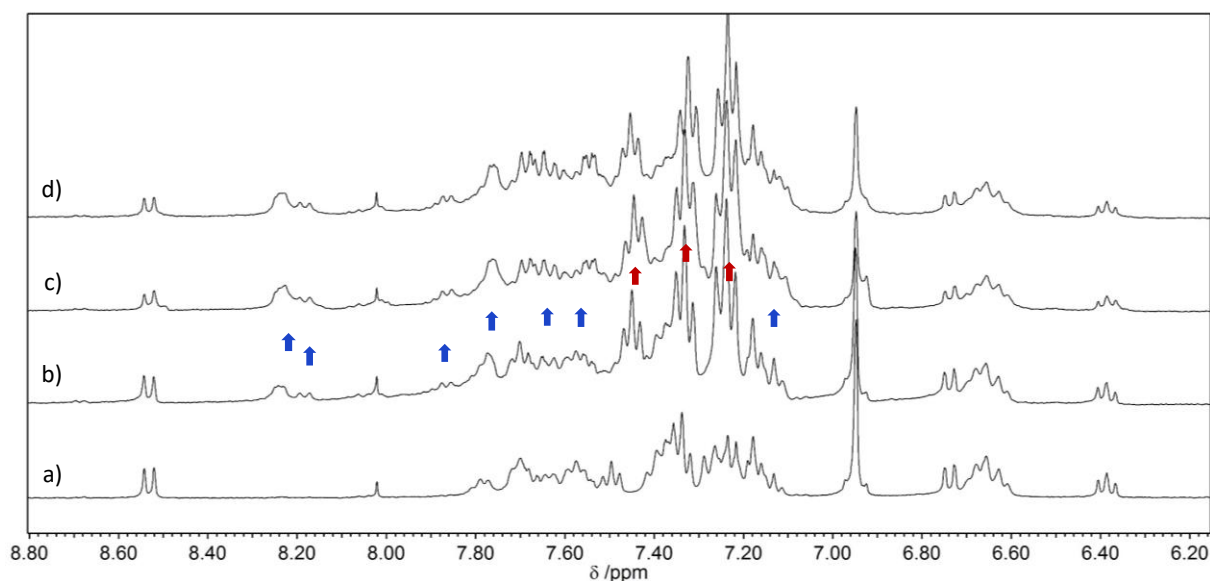
Figure III-17 : Portion du spectre RMN ^1\text{H} de Z-91 dans (\text{CD}_3)_2\text{CO} ( C = 4,8 \text{ mM} ) avant irradiation (a) et après irradiation à 406 \text{ nm} ( P = 20 \text{ mW}\cdot\text{cm}^{-2} ) pendant 30 min (b), 80 min (c) et 120 min (d). Les flèches montrent les signaux des protons aromatiques de 71 (bleu) et \text{PPh}_3 (rouge) apparaissant sous irradiation.
