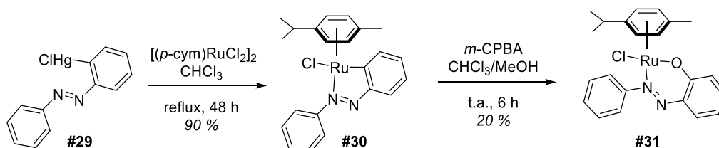
Schéma I-20 : Synthèse des complexes #30 et #31 .
