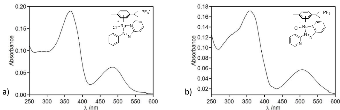
Figure II-5 : Spectres d'absorption dans \text{CH}_3\text{CN} des composés 27 (a) et 28 (b) ( C \sim 10^{-5} M).
