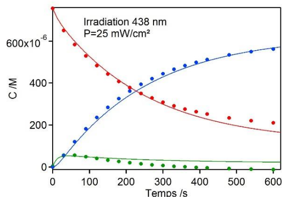
Figure A-7 : Profils temporels de concentrations et courbes d'ajustement pendant l'irradiation à 438 nm d'une solution de Z-121 ( \text{CH}_3\text{CN} , C = 0,76 mM). Z : rouge, Z' : bleu, E : vert.
