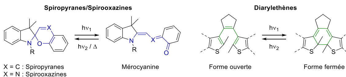
Schéma I-2 : Cyclisation des spiropyranes/spirooxazines et diaryléthènes.
