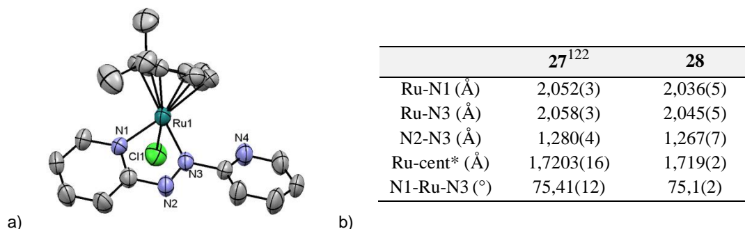
Figure II-3 : a) Représentation ORTEP du composé 28 . Les atomes d'hydrogène et le contre-ion \text{PF}_6^- ont été omis par soucis de clarté. b) Longueurs de liaisons et angles sélectionnés pour le composé 28 en comparaison avec les données de la littérature pour 27 . *cent : centroïde du groupement p -cymène.
