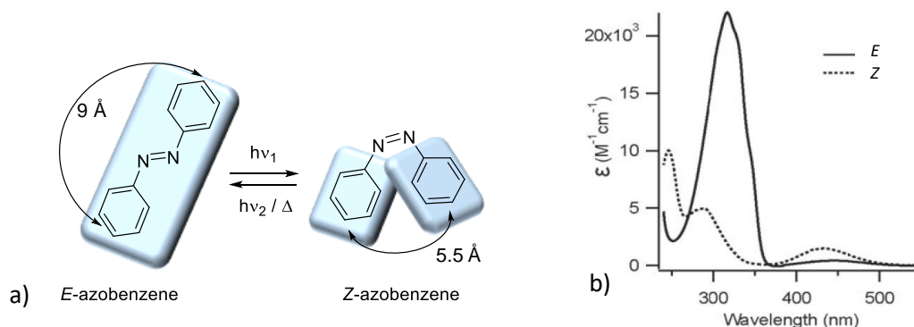
Figure I-3 : a) Photo-isomérisation de l'azobenzène. b) Spectres d'absorption UV-visible des isomères E et Z dans l'éthanol. 14
