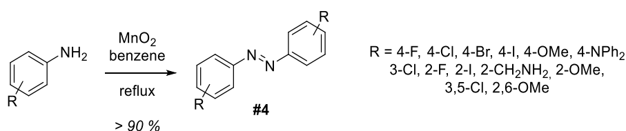
Schéma I-5 : Synthèse d'azobenzènes symétriques par couplage oxydant d'anilines avec MnO_2 .
