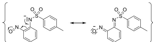
Schéma III-7 : Contribution mésomère possible expliquant la faible électrophilie de l'atome d'azote du composé 13 en milieu basique.
