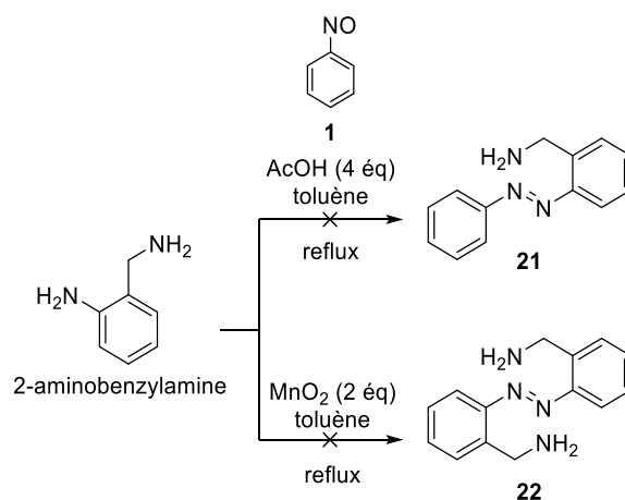
Schéma II-10 : Tentative de synthèse des composés 21 et 22 .
