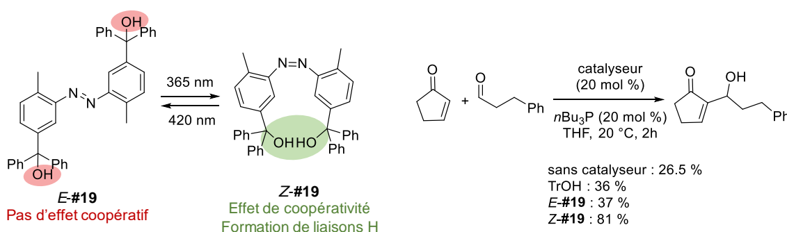
Schéma I-15 : Accélération de la réaction de Morita-Baylis-Hillman par effet de coopération induit par photo-isomérisation.
