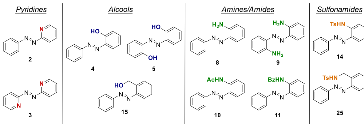
Figure II-2 : Structures des différents azobenzènes synthétisés.
