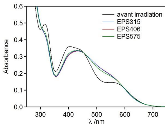
Figure II-21 : Spectre d'absorption du composé 37 dans \text{CH}_3\text{CN} ( C = 50 \mu\text{M} ) avant irradiation (courbe noire) et EPS obtenus après irradiation à 315 nm (courbe bleue), 406 nm (courbe rouge) ou 575 nm (courbe verte).
