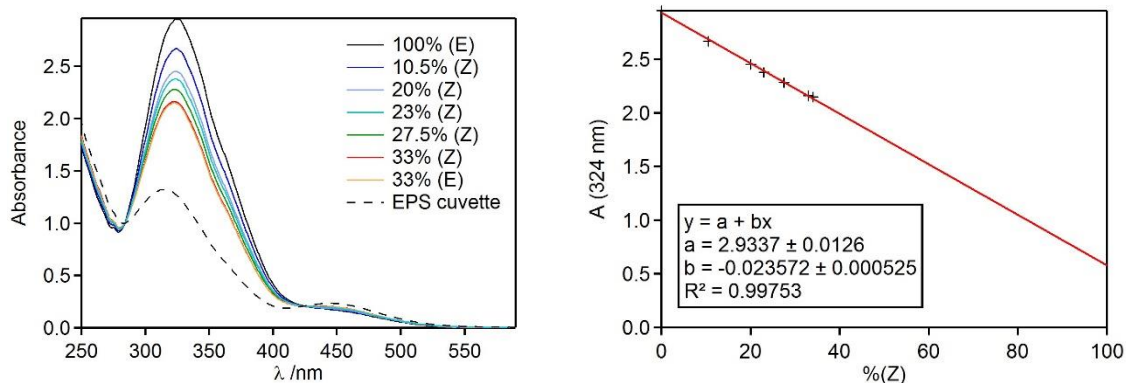
Figure A-2 : Spectre d'absorption de 14 dans \text{CH}_3\text{CN} à différentes proportions de Z. Tracé de l'absorbance à 324 nm en fonction du pourcentage d'isomère Z.
