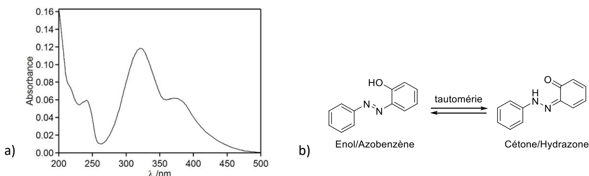
Figure II-12 : a) Spectre d'absorption de 4 dans CH 3 CN ( C \sim 10^{-6} M). b) Tautomérie azo/hydrazone de 4 .
