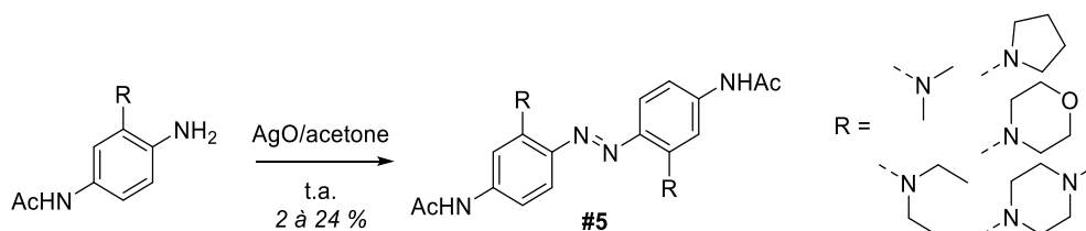
Schéma I-6 : Synthèse d'azobenzènes par couplage oxydant d'anilines avec AgO .
