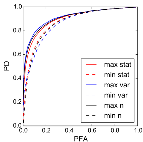
(a) Cas homoscédastique. Le paramètre de la distribution est \lambda = 1 pour \mathbf{x}_{(1)} et \mathbf{x}_{(2)} et les observations de \mathbf{x}_{(2)} sont décalées de 0,5.
