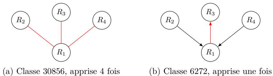
FIGURE 5.27 – CPDAG des principales classes d'équivalence obtenues pour les données électriques avec la méthode GES et le score KL. Les arêtes dont l'orientation diffère par rapport à G_h sont en rouge.
