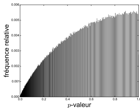
(b) Fonction masse avec n_1 = n_2 = 50 .
