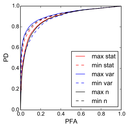
(b) Cas homoscédastique. Le paramètre de la distribution est \lambda = 1 pour \mathbf{x}_{(1)} et \mathbf{x}_{(2)} et les observations de \mathbf{x}_{(2)} sont décalées de -0,5 .
