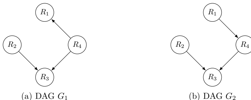
FIGURE 5.4 – Les deux extensions possibles du CPDAG H de la figure 5.3.
