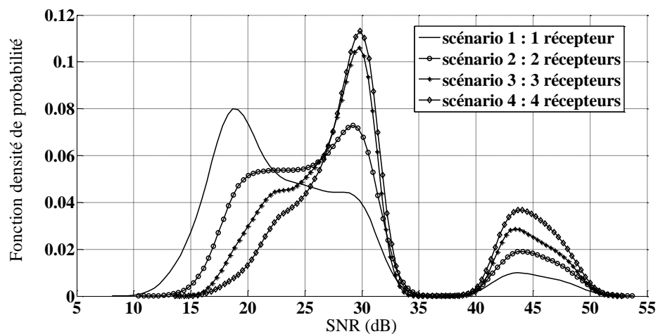
Figure 35 : Densité de probabilité du SNR reçu dans un système SIMO, cas C , \rho=0,8 , P_t = 22 mW, R_b = 5 kbit/s
