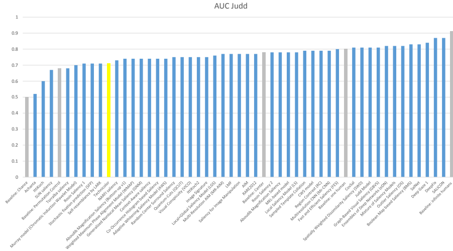
Figure A.2: Benchmark of the Technicolor’s visual attention model on the MIT dataset: AUC Judd metric.
