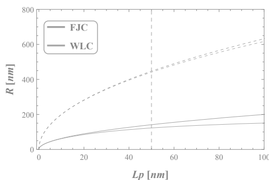
Fig. 2.10 – Comparaison des modèles FJC et WLC . Représentation de l'influence du modèle sur la distance bout-à-bout avec L = 200 nm Fig. 2.11 – Comparaison des modèles FJC et WLC , de l'influence de L sur R . Courbes pleines L = 200 nm, courbes pointillées L = 2000 nm
