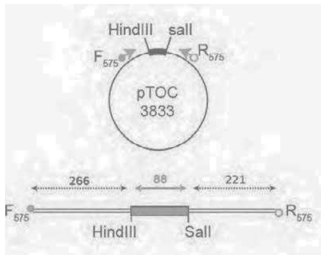
Fig. 6.1 – Schéma du plasmide et de la construction des ADN utilisés
