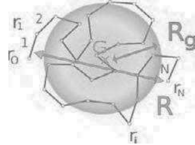
Fig. 2.6 – Rayon de giration, R_g , dans un espace 2D. Nombre de segments N=27
