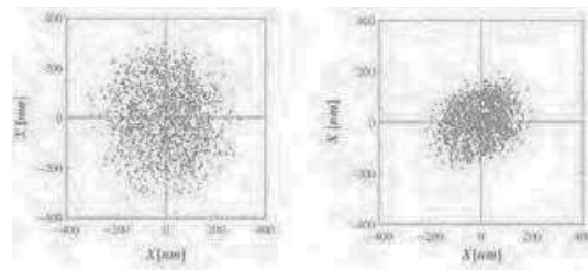
Fig. 3.24 – Illustration de la différence d'asymétrie entre distributions (ADN L_{ADN}=1201 bp, R_{par} = 150 nm)
