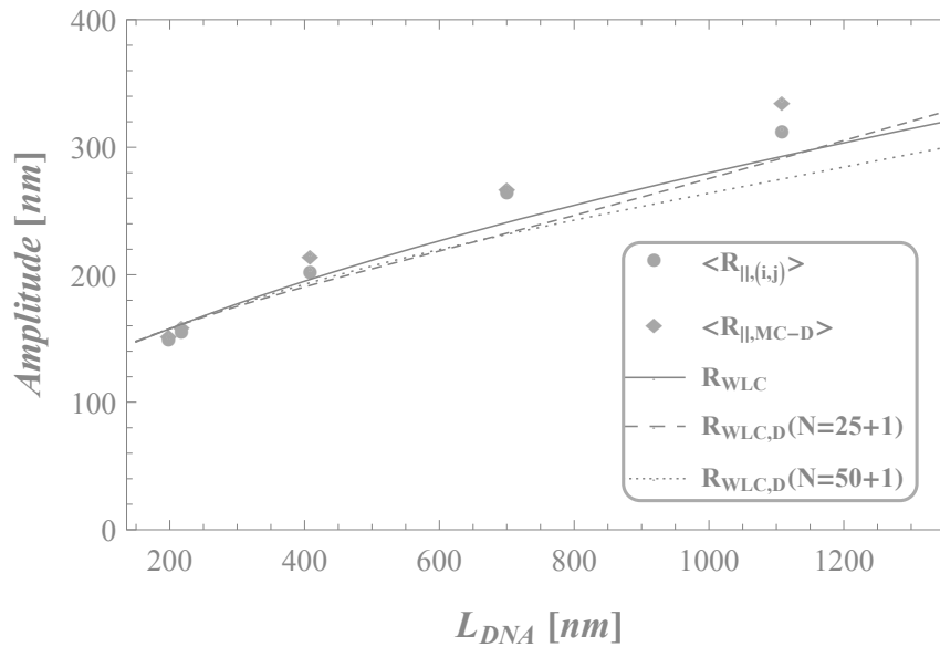
Fig. 4.8 – Courbe de calibration des amplitudes simulées, \langle R_{||,MC-D} \rangle , et expérimentales, \langle R_{||,(i,j)} \rangle . Pour L_{ADN} = 583, 639, 1201 bp, N = 25 + 1 , tandis que pour L_{ADN} = 2060, 3259 bp, N = 50 + 1 ; R_{par} = 150 nm pour toutes les simulations. La courbe continue correspond au modèle WLC , la courbe discontinue correspond au modèle WLC Discret pour N = 25 + 1 tandis que la courbe en pointillés correspond à N = 50 + 1
