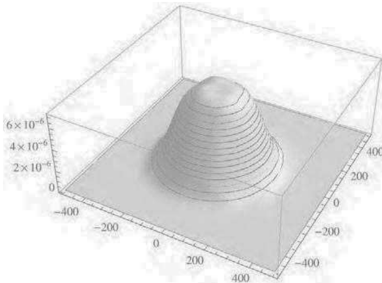
Fig. 3.42 – Distribution de probabilité en 3 dimensions des positions X_{\text{corr},i,j} et Y_{\text{corr},i,j} de l'ensemble des trajectoires conservées ( L_{ADN} = 1201 bp, R_{par} = 150 nm)
