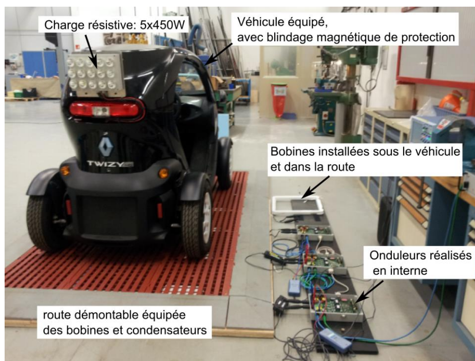
Figure 6-5: photo du prototype Twizy sur 3 mètres de route
