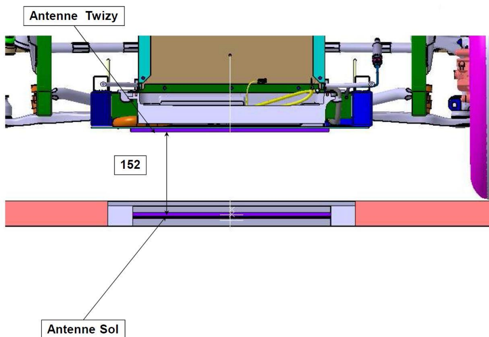
Figure 6-2: vue en coupe de la route et du véhicule équipé
