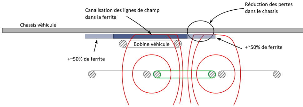
Figure 5-4: Principe du blindage magnétique du véhicule
