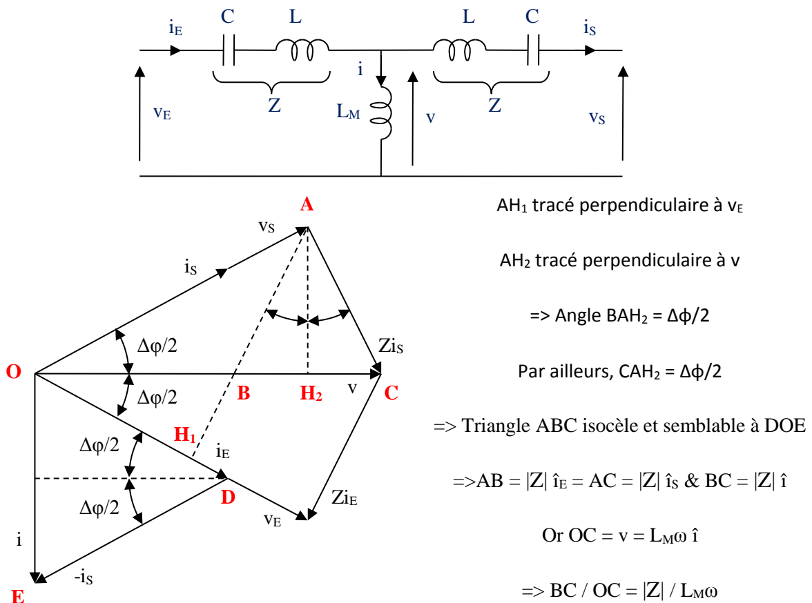
Figure 3-13: Propriétés géométriques du diagramme de Fresnel « idéal »
