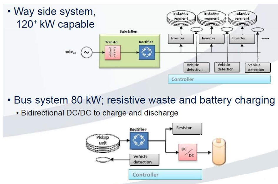
Figure 1-10: Principe de la route électrique Bombardier [40]
