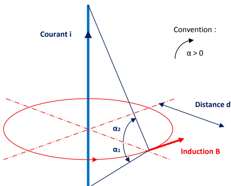
Figure 2-8: Influence d'un courant sur l'environnement magnétique
