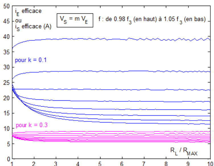
Figure 4-13: Courants efficaces dans le mode 3 particulier
