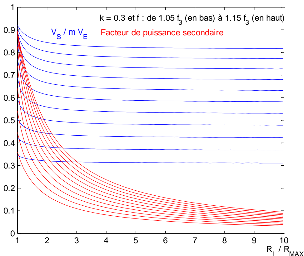
Figure 4-15: Gain en tension et facteur de puissance au secondaire dans le mode 4
