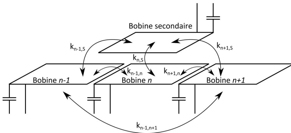
Figure 5-5: représentation d'un circuit multi-primaires
