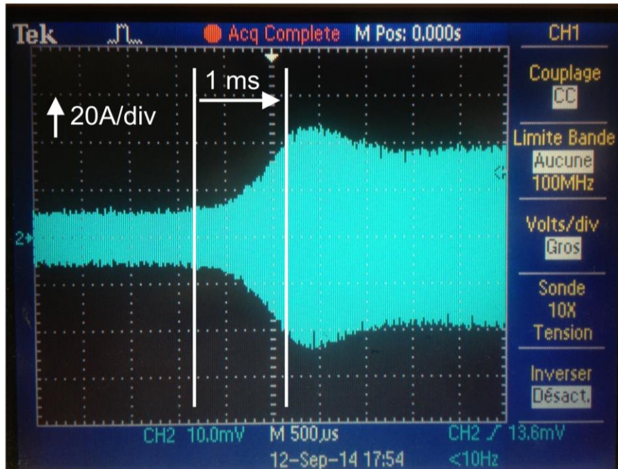
Figure 6-8: courant primaire avec échelon de courant de 30 ampères
