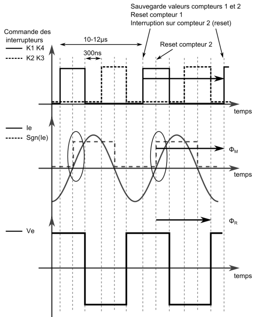
Figure B-1 : Principe de la mesure numérique du déphasage
