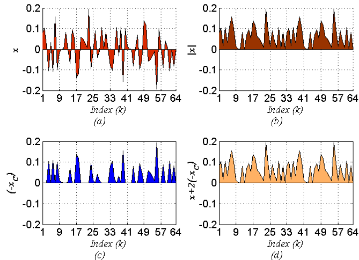
Figure A. 2 : (a) signal x(k) à la sortie de l'IFFT en ACO-OFDM, (b) Module du signal x(k) , (c) signal (-x(k)) clippé, (d) signal résultant de x(k) + 2(-x(k))_C .
