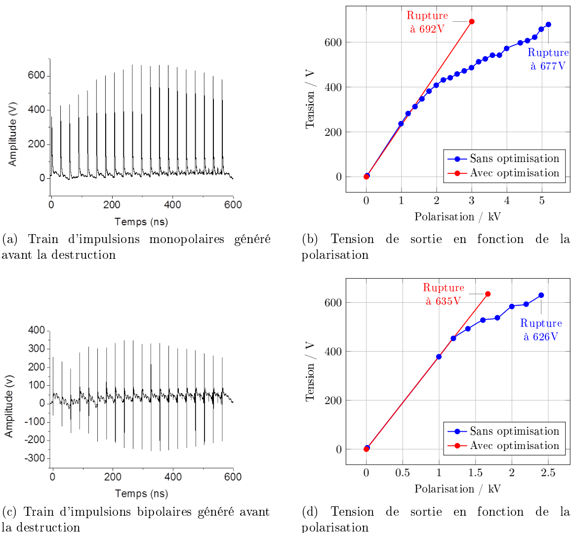
Fig. II.21 – Résultats obtenus pour la génération de train d'impulsions
