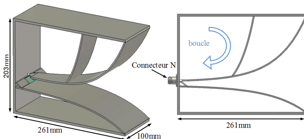
Fig. II.22 – Antenne K d'origine
