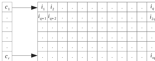
Figure 10.7 – Représentation de la MFU. C'est une table de hachage contenant r clés associées à r tables de hachage P_{c_j} . Chaque table P_{c_j} contient q clés représentant la position des données dans E associées à la position du nœud dans l'arbre où se situe la donnée.
