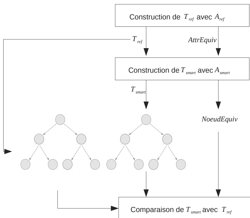
Figure 11.1 – Procédure pour vérifier la stabilité de SMART
