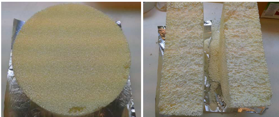
Figure 5 : Homogénéité du dépôt de wash-coat 2,4%CeO 2 /30ppi (synthèse 2 tableau 1).
