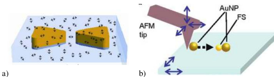
FIGURE 4.2 – a) Antenne noeud papillon couplée à des fluorophores. [77] b) Contrôle de la distance entre une sphere fluorescente et deux particules d'or. [78]
