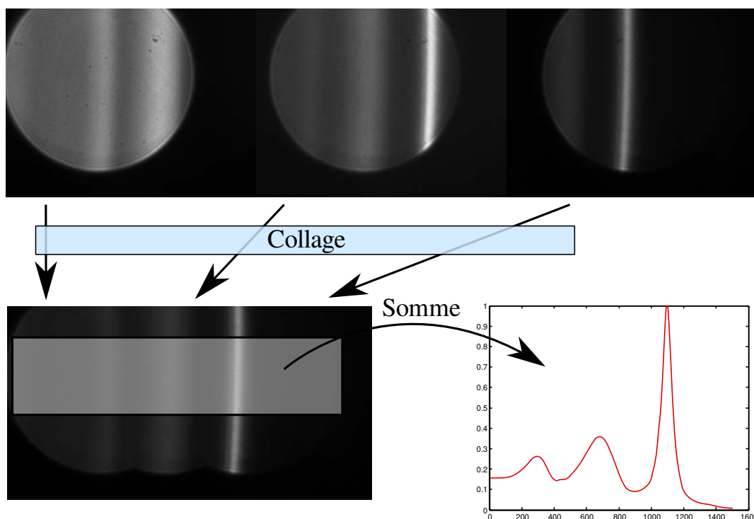
FIGURE 3.11 – Reconstruction informatique de I(\theta) sur plan de Fourier étendu avec correction des contrastes.
