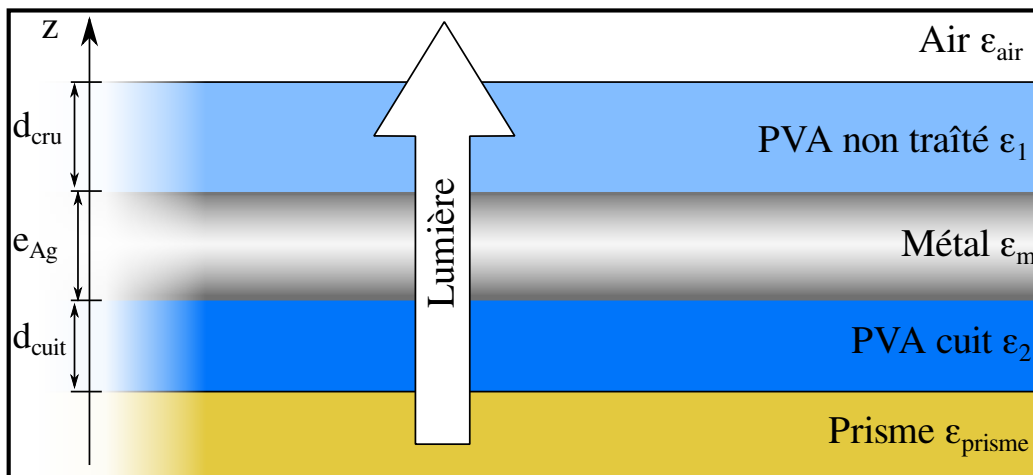
FIGURE 2.9 – Géométrie du système simulé.
