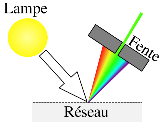
FIGURE 3.2 – Principe d'un monochromateur.
