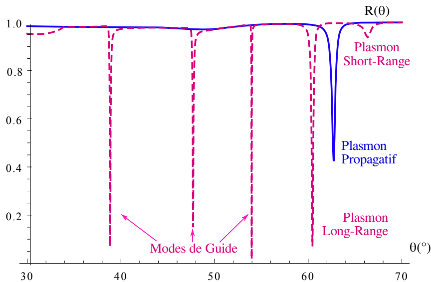
FIGURE 2.10 – Réflectivité calculée d'une géométrie type "plasmon propagatif" comparée à la réflectivité d'une géométrie "plasmon long-range".
