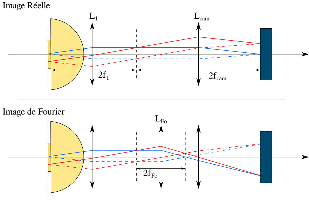
FIGURE 3.8 – Illustration du principe d'observation des espaces réels et de Fourier.
