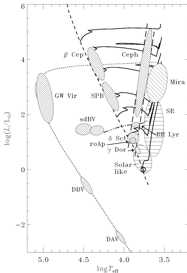
Figure 1.2: Diagramme de Hertzsprung-Russell (HR) représentant la luminosité en fonction de la température. Les lignes noires pleines indiquent le chemin évolutif pour les étoiles de masses (du haut vers le bas) de 20, 12, 7, 4, 3, 2 et 1 M_{\odot} . Chaque cercle hachuré indique une région d'instabilité dans le diagramme HR et le type de hachures correspond à un mécanisme d'excitation. Les pulsateurs de type solaire sont représentés par un cercle avec des hachures horizontales, au niveau du bas de la séquence principale et le haut de la branche des géantes rouges. Crédit : J. Christensen-Dalsgaard
