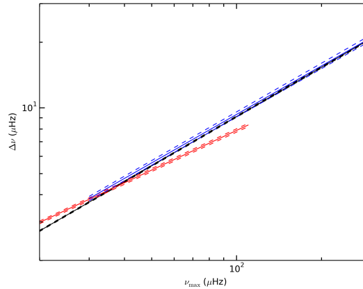
Figure 5.5: Relations d'échelle du paramètre \Delta\nu , avec leurs encadrements, déterminées en utilisant l'ensemble des données Kepler (en noir), uniquement les étoiles du clump (en rouge) et uniquement celles de la RGB (en bleu).
