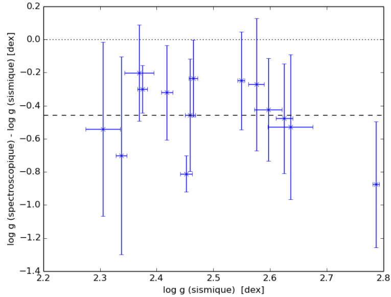
Figure 5.17: Différence des valeurs de la gravité de surface \log g déduits à partir des données spectroscopiques (GES DR1) et astérosismiques (CoRoT) en fonction des valeurs astérosismiques. Les tirets indiquent la moyenne des différences : \langle \log g_{\text{spectroscopique}} - \log g_{\text{sismique}} \rangle = -0,46 \pm 0,21 [dex].
