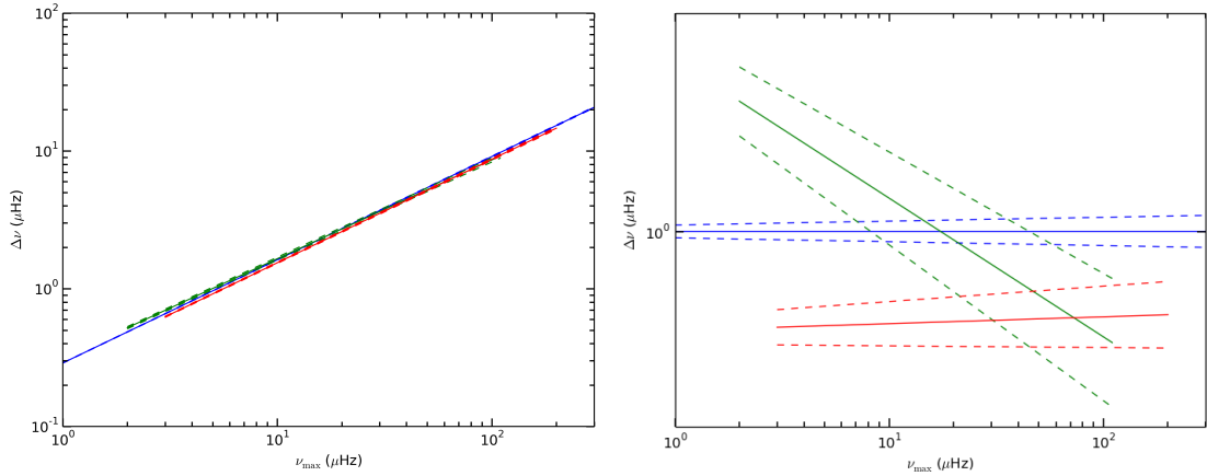
Figure 5.4: Relations d'échelle du paramètre \Delta\nu que nous avons obtenu avec les données CoRoT (en vert) et Kepler (en bleu), ainsi que celle obtenue par Mosser et al. (2012a) (en rouge). Les traits pleins représentent les relations d'échelle déduites de l'ensemble des résultats après un ajustement par moindres carrés en considérant les erreurs internes suivant l'axe des ordonnées. Les tirets représentent les valeurs extrêmes que les relations d'échelle peuvent prendre en considérant les erreurs associées sur le coefficient \alpha et l'exposant \beta .
