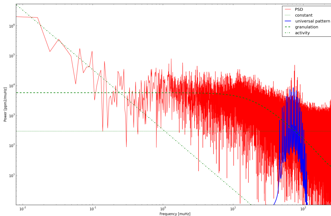
Figure 2.3: En rouge, la densité spectrale de puissance de l'étoile Kepler KIC 11565235 en fonction de la fréquence. En vert, la composante d'activité (en point-tiret), de granulation (en tiret) et de bruit blanc (en pointillée). En bleu, le spectre synthétique d'oscillations.
