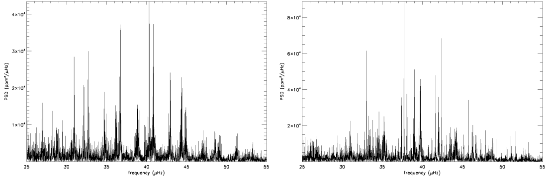
Figure 2.6: Deux spectres de géantes rouges. À gauche, le spectre de l'étoile KIC 1433730 situé en haut de la RGB ( \nu_{\text{max}} = 38,9 \mu\text{Hz} , \Delta\nu = 4,03 \mu\text{Hz} et \Delta\Pi_1 = 60,7 \text{ s} ) ; À droite, celui de l'étoile KIC 1163453 se trouvant dans le clump ( \nu_{\text{max}} = 39,0 \mu\text{Hz} , \Delta\nu = 4,41 \mu\text{Hz} et \Delta\Pi_1 = 271 \text{ s} ).
