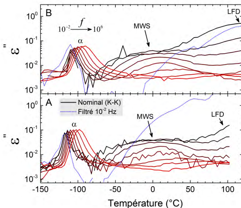
Figure IV.16 – Thermogrammes isofréquences (de 10^{-2} à 10^6 Hz) des pertes diélectriques \epsilon''_{K-K} (transformations de Kramers-Kronig) de l'échantillon nominal vierge (A) et irradié à 9,8 \cdot 10^5 Gy (B). Les pertes à 10^{-2} Hz dans le matériau filtré vierge et irradié à la même dose apparaissent en traits pointillés.
