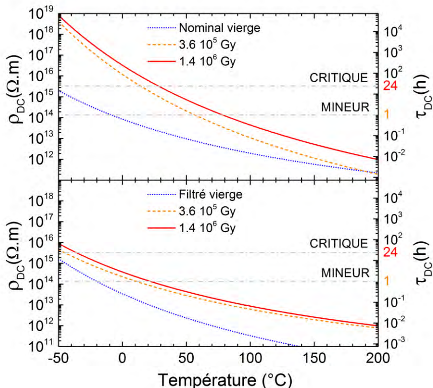
Figure IV.25 – Extrapolation des lois d'Arrhenius de la résistivité obtenues en RPI sur la gamme de températures [-50, 200 \text{ }^\circ\text{C}] , pour les matériaux nominal (haut) et filtré (bas). Les constantes de temps \tau_{DC} de la dissipation des charges accumulées à la surface, et les risques de décharge électrostatique associés, sont également représentés.
