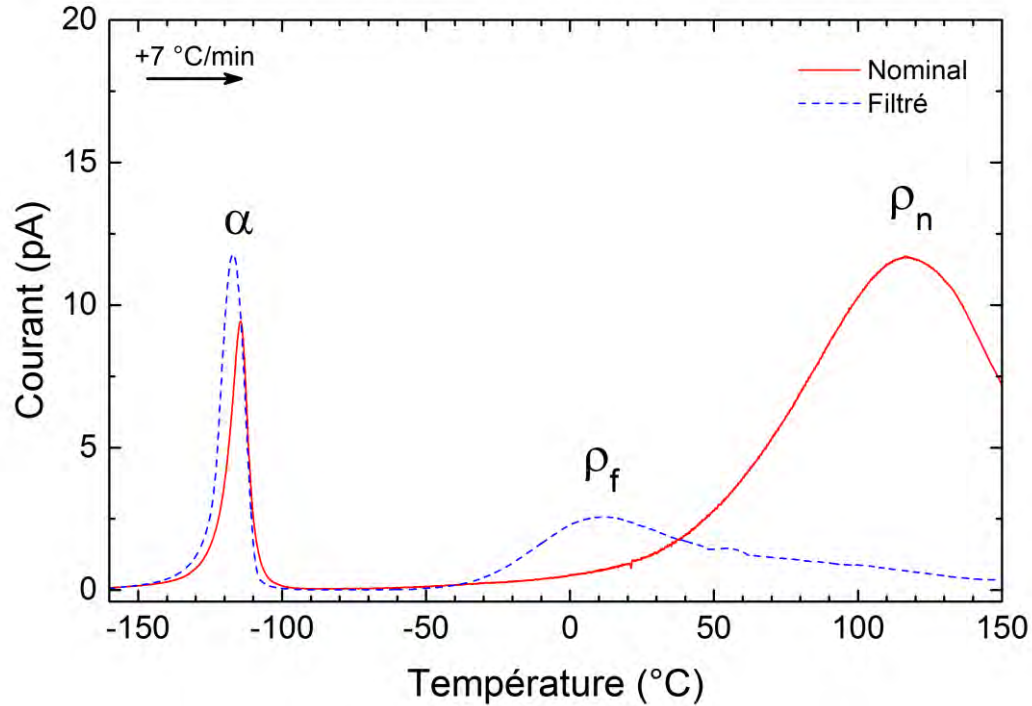
Figure III.14 – Thermogrammes complexes des courants de dépolariation des matériaux nominal et filtré en CTS.
