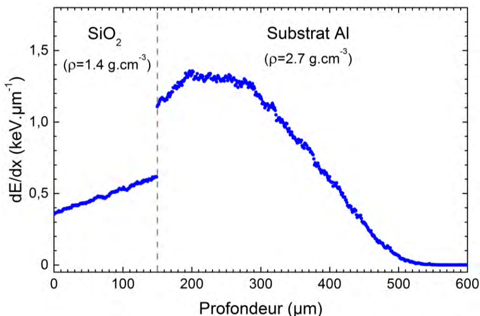
Figure IV.1 – Perte d'énergie d'un électron incident de 400 keV dans la configuration expérimentale ( 10^4 électrons simulés sous Casino).
