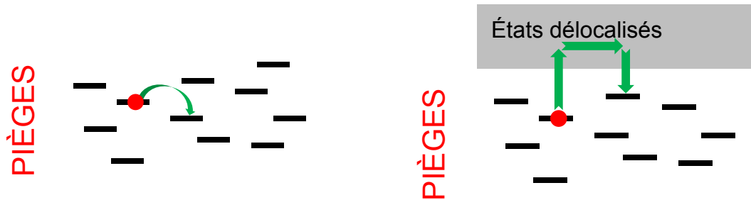
Figure I.12 – Schémas des mécanismes de hopping (gauche) et de multiple-trapping-and-release (droite).
