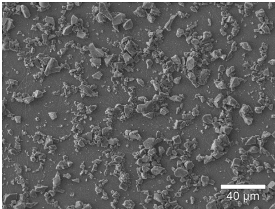
Figure III.1 – Image MEB des particules en mode électrons secondaires ( E_0 = 10 \text{ keV} ).
