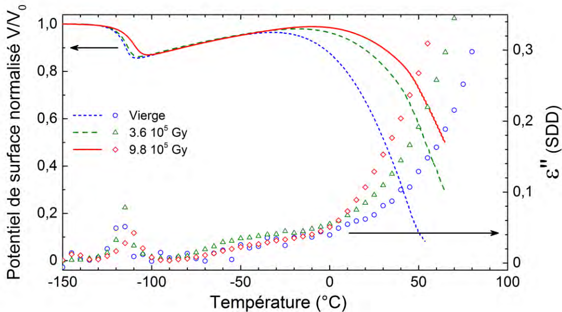
Figure IV.20 – Superposition des thermogrammes en RPTS et en SDD ( \varepsilon'' à 10^{-2} \text{ Hz} ) du matériau nominal vierge et irradié à 3.6 \cdot 10^5 et à 9.8 \cdot 10^5 \text{ Gy} .
