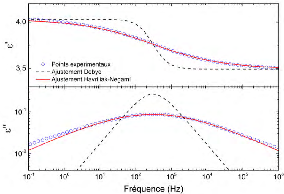
Figure II.4 – Points expérimentaux de \varepsilon' et \varepsilon'' en fonction de la fréquence, à l'isotherme T = -108 °C (mode de relaxation dipolaire \alpha ), sur l'adhésif silicone étudié dans ce manuscrit. Les traits pointillés et plein représentent les ajustements mathématiques de Debye et d'Havriliak-Negami.
