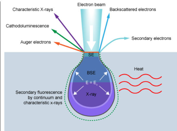
Figure I.17 – Poire d'interaction des électrons avec les différents signaux observables par les techniques de microcaractérisation. Reproduction de Australian Microscopy and Miroanalysis Research Facility (license creative commons).
