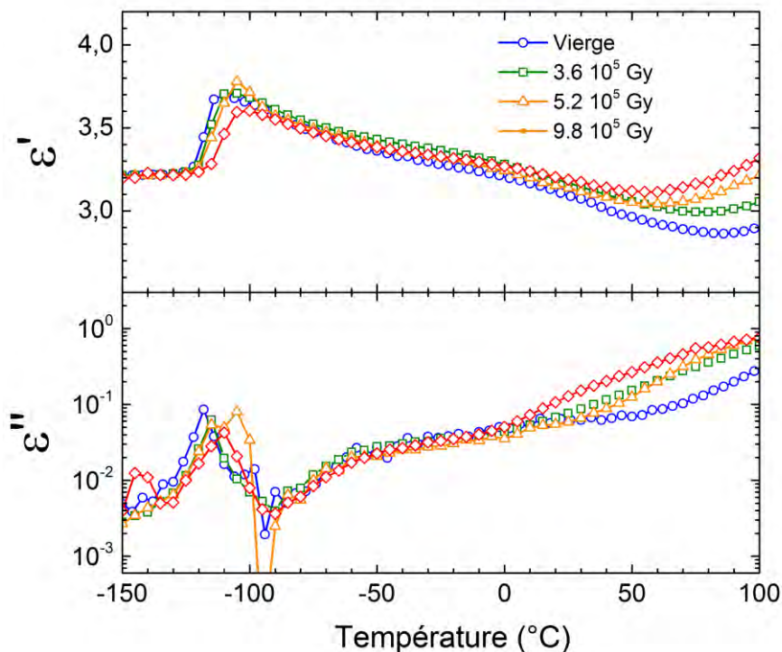
Figure IV.15 – Thermogrammes isofréquences ( 10^{-2} Hz) des parties réelle ( \epsilon' ) et imaginaire ( \epsilon'' ) mesurées en SDD sur le matériau nominal vierge et irradié à différents niveaux de dose.
