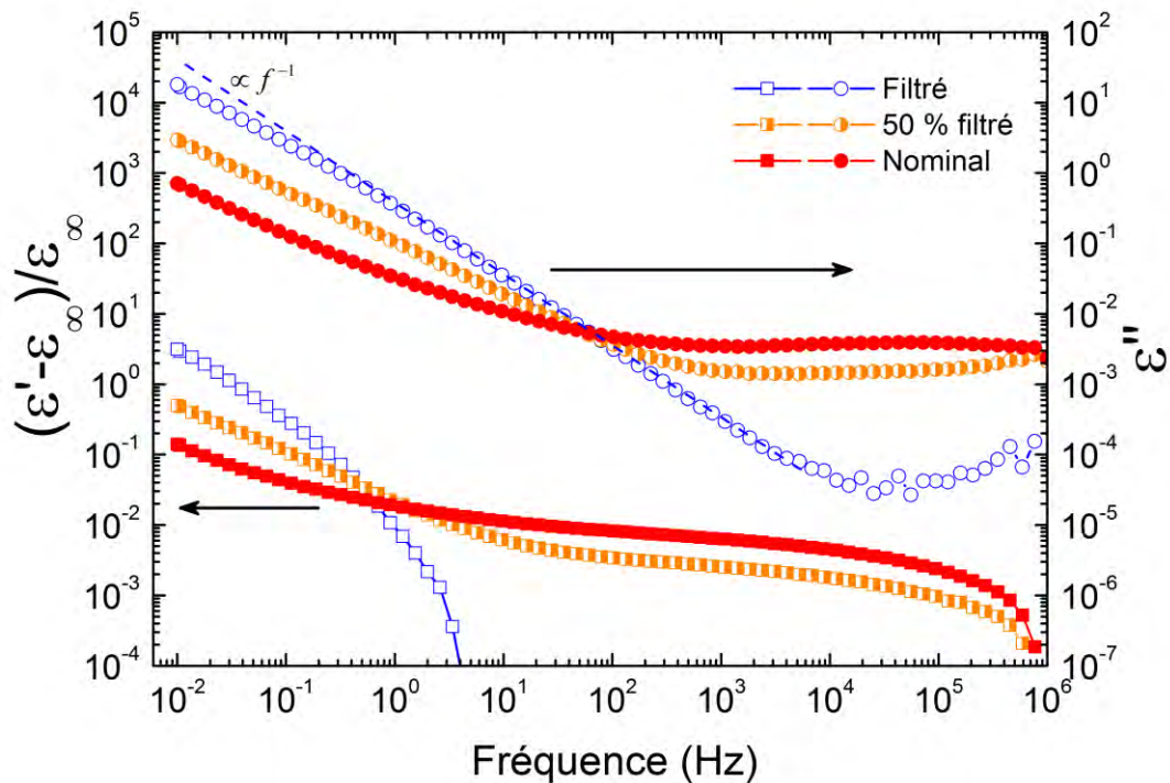
Figure III.22 – Spectres \varepsilon'(f) et \varepsilon''(f) des matériaux nominal et filtré à T = +100\text{ }^\circ\text{C} . Le nombre de décades sur chaque échelle est le même afin de pouvoir comparer les pentes des lois de puissance.
