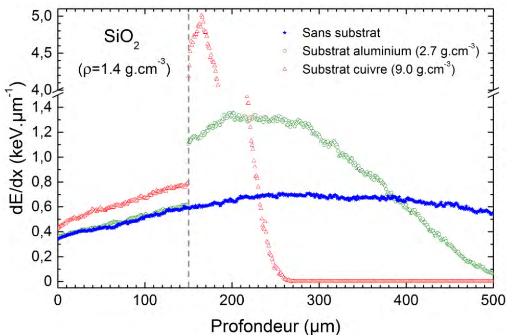
Figure A.1 – Simulation sous Casino de la perte d'énergie d'un électron incident de 400 keV dans trois configurations différentes.
