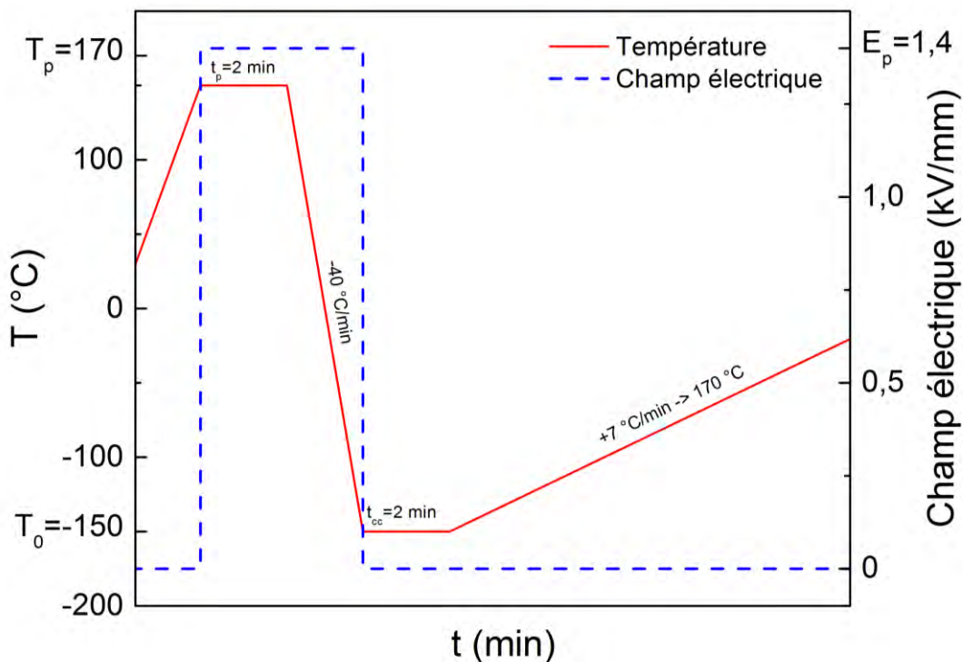
Figure II.6 – Protocole expérimental pour l'obtention d'un thermogramme de dépolariation complexe.
