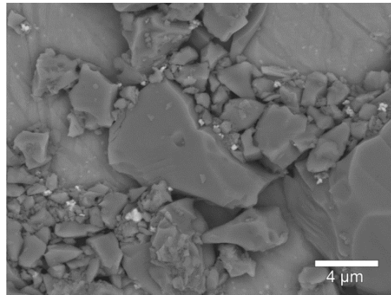
Figure III.2 – Image MEB des particules en mode électrons rétrodiffusés ( E_0 = 10 \text{ keV} ) montrant la présence de 2 types de particules. Les plus volumineuses et nombreuses sont composées d'éléments plus légers que les petits agrégats qui apparaissent plus brillants.
