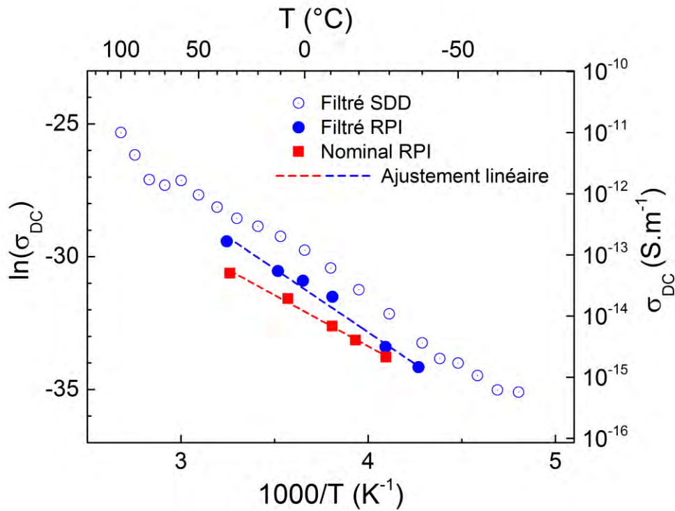
Figure III.29 – Diagramme d'Arrhenius de \sigma_{DC}(1000/T) des matériaux nominal (RPI) et filtré (RPI et SDD).
