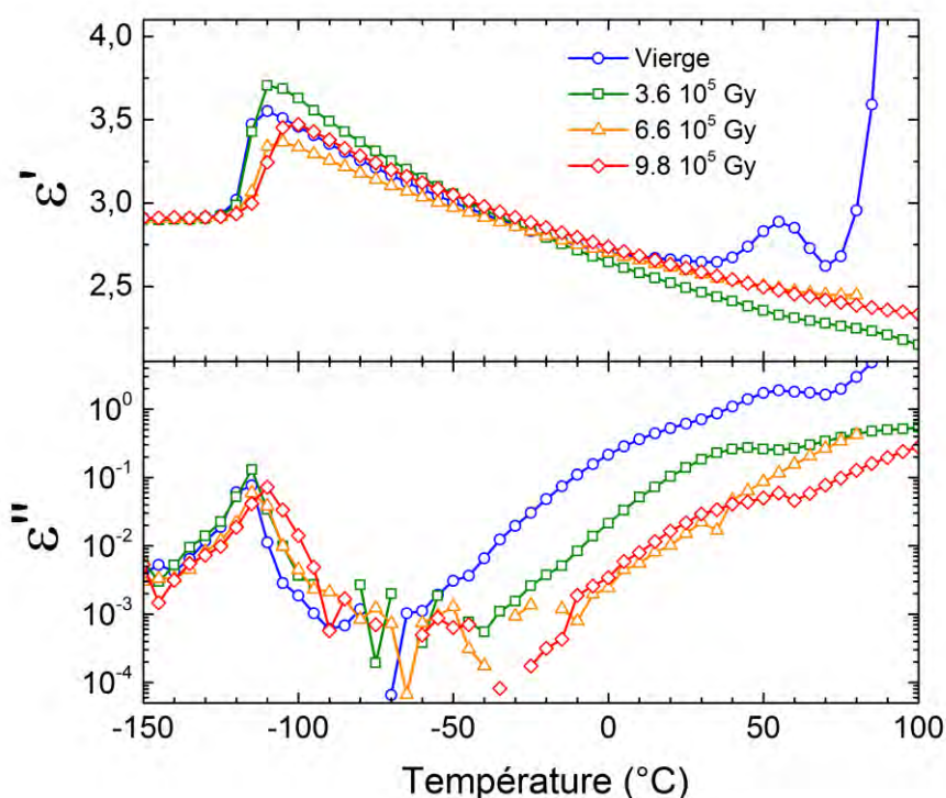
Figure IV.13 – Thermogrammes isofréquences ( 10^{-2}\text{ Hz} ) des parties réelle ( \varepsilon' ) et imaginaire ( \varepsilon'' ) mesurées en SDD sur le matériau filtré vierge et irradié à différents niveaux de dose.
