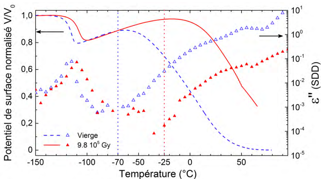
Figure IV.19 – Superposition des thermogrammes en RPTS et en SDD ( \varepsilon'' à 10^{-2} \text{ Hz} ) du matériau filtré vierge et irradié à 9.8 \cdot 10^5 \text{ Gy} .
