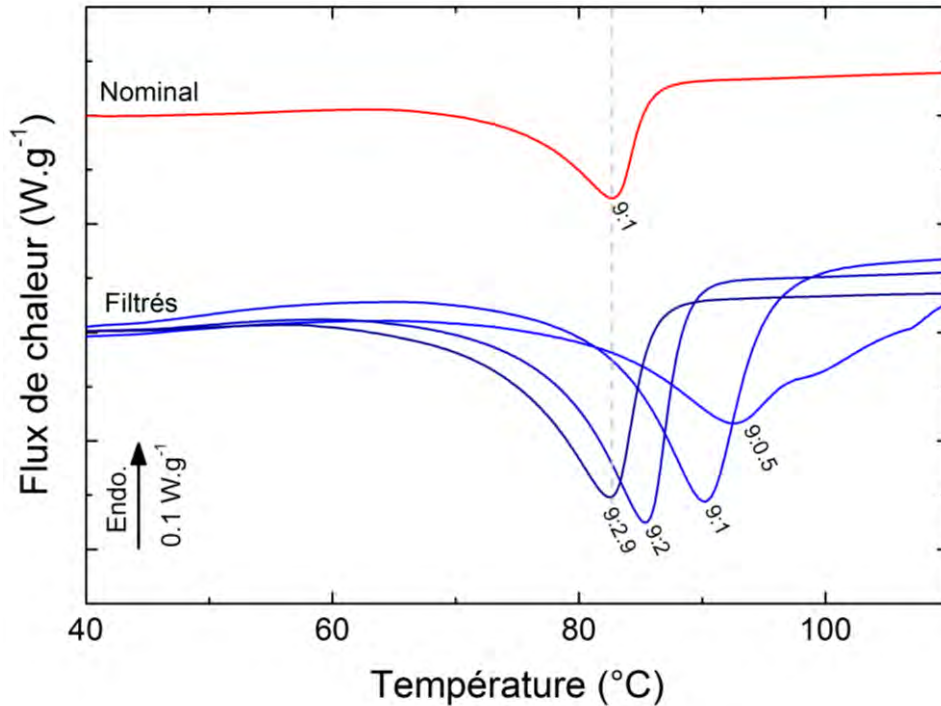
Figure III.7 – Pic de réticulation initial ( t = 9 \text{ min} ) en ACD de différents mélanges de base filtrée avec du durcisseur nominal.
