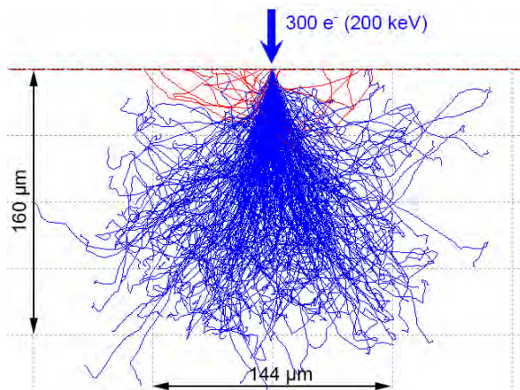
Figure I.16 – Simulation sous le logiciel Casino de la pénétration de 300 électrons d'énergie initiale 200 keV focalisés sur un substrat d'aluminium. Les électrons rétrodiffusés, réémis à la surface de l'échantillon, apparaissent en rouge.
