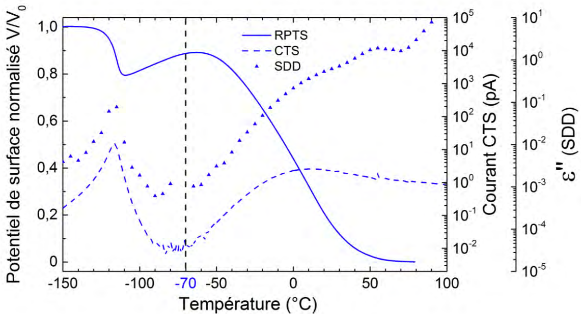
Figure III.34 – Superposition des thermogrammes thermo-stimulés (RPTS et CTS) et isotherme (SDD à 10^{-2} Hz) du matériau filtré.
