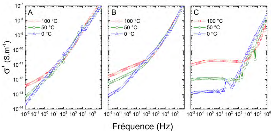
Figure III.21 – Trois spectres de conductivité isothermes (0, +50 et +100 °C) obtenus en SDD pour : (A) un échantillon nominal, (B) un échantillon au taux de particules de ~28 % m , et (C) un échantillon filtré.
