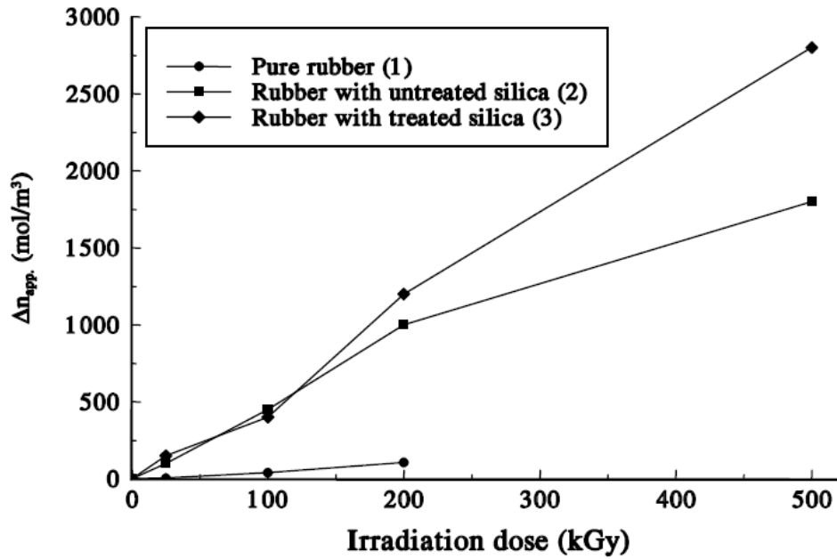
Figure I.23 – Variation de la densité de réticulation apparente avec la dose ionisante pour : (1) un élastomère de PDMS pur, (2) un élastomère de PDMS avec 30 % vol de silice non fonctionnalisée et (3) un élastomère de PDMS avec 30 % vol de silice fonctionnalisée. Reproduction de [153].
