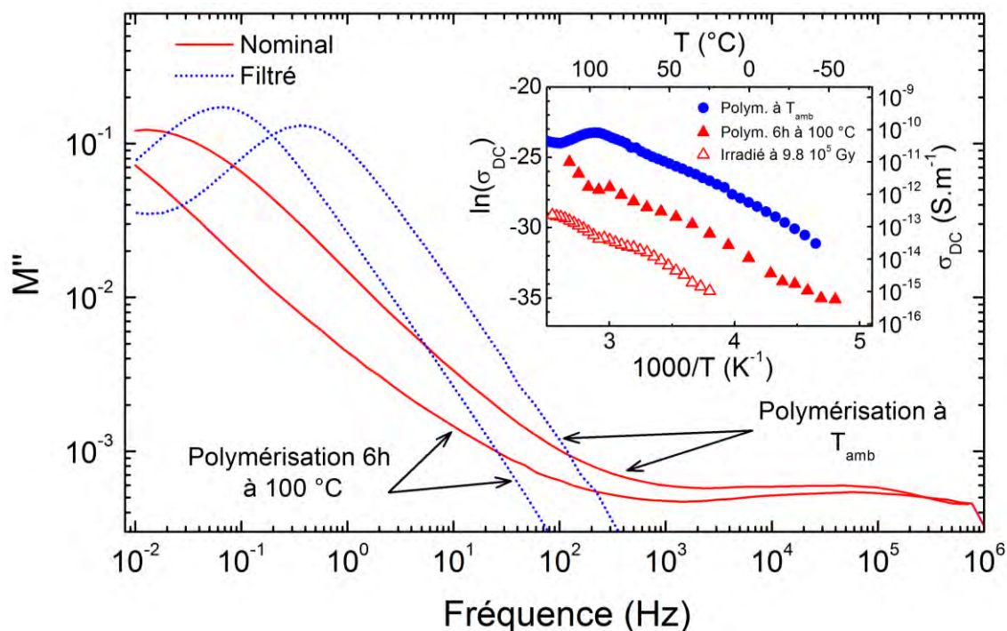
Figure IV.24 – Influence du recuit sur M''(T = 100\text{ °C}) des matériaux nominal et filtré. En encart : diagramme d'Arrhenius de \sigma_{DC} (mesurée sur les plateaux DC de \sigma'(f) ) du matériau filtré polymérisé 7 jours à température ambiante, recuit 6h à 100\text{ °C} et recuit puis irradié à la dose de 9.8 \cdot 10^5\text{ Gy} .
