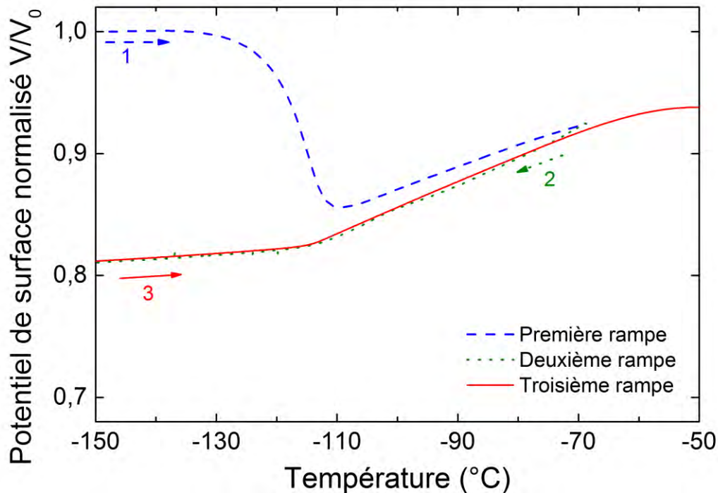
Figure III.17 – Rampes successives en RPTS au voisinage de T_g^{ACD} sur le matériau nominal.
