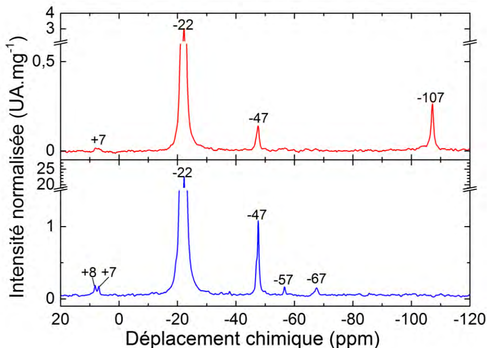
Figure III.9 – Spectres en RMN du 29Si (mode SP-MAS) des matériaux nominal (haut) et filtré (bas).
