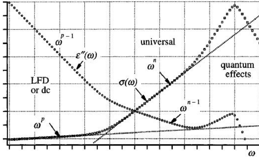
Figure I.15 – Représentation des spectres de conductivité \sigma'(\omega) et de pertes diélectriques \epsilon''(\omega) d'un solide désordonné, faisant apparaître le comportement en loi de puissance fractionnelle. Selon Jonscher [69].
