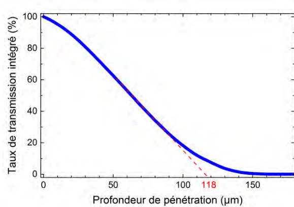
Figure I.19 – Simulation sous Casino du taux de transmission intégré en fonction de la profondeur d'arrêt. La portée pratique est représentée en trait pointillé.
