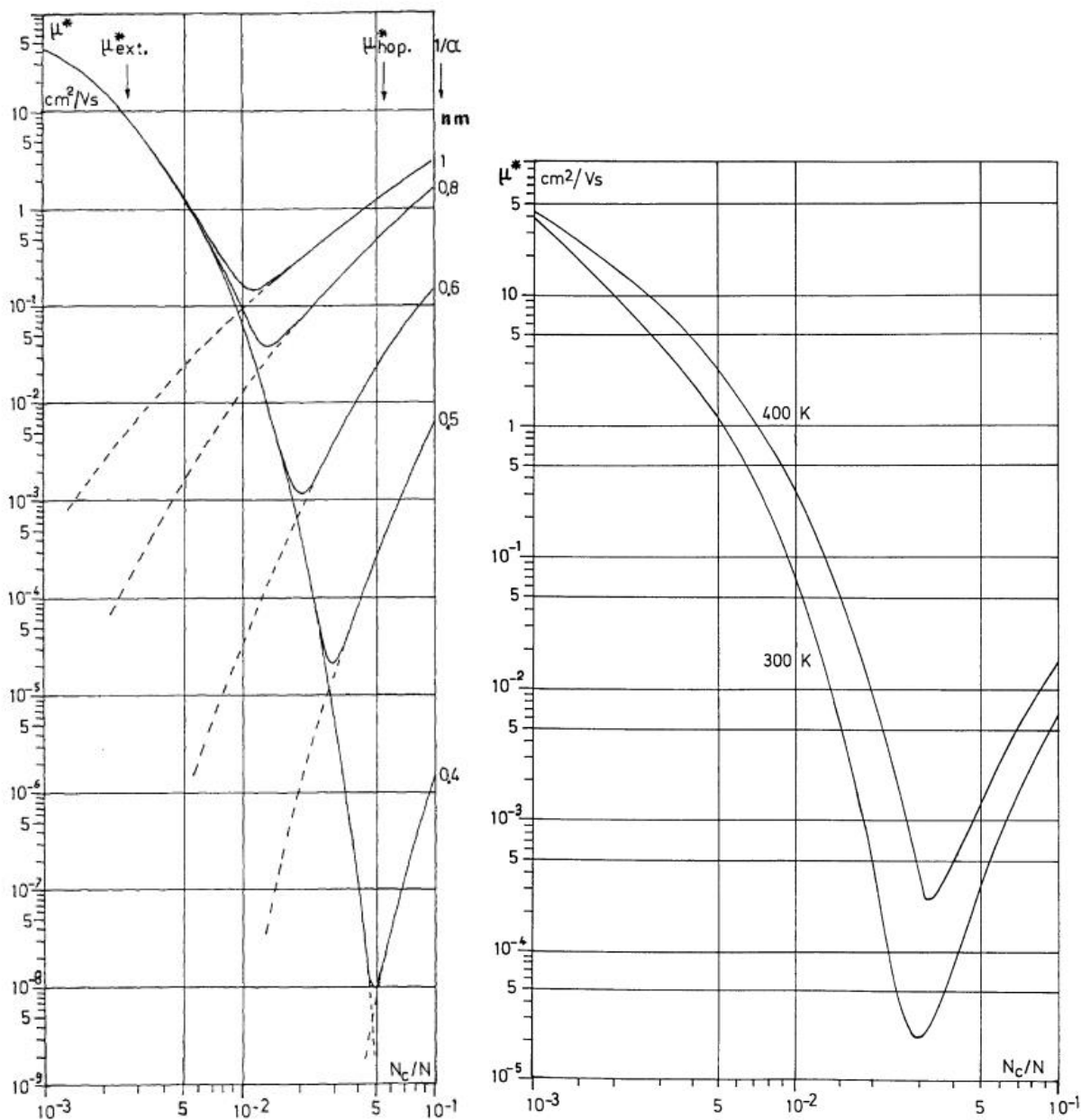
Figure I.13 – Variation de la mobilité dans les états délocalisés \mu_{\text{ext}}^* et de la mobilité de hopping \mu_{\text{hop}}^* avec le désordre, pour différentes longueurs de localisation \frac{1}{\alpha} de l'électron (gauche) et à deux températures différentes (droite). Reproduction de [49].
