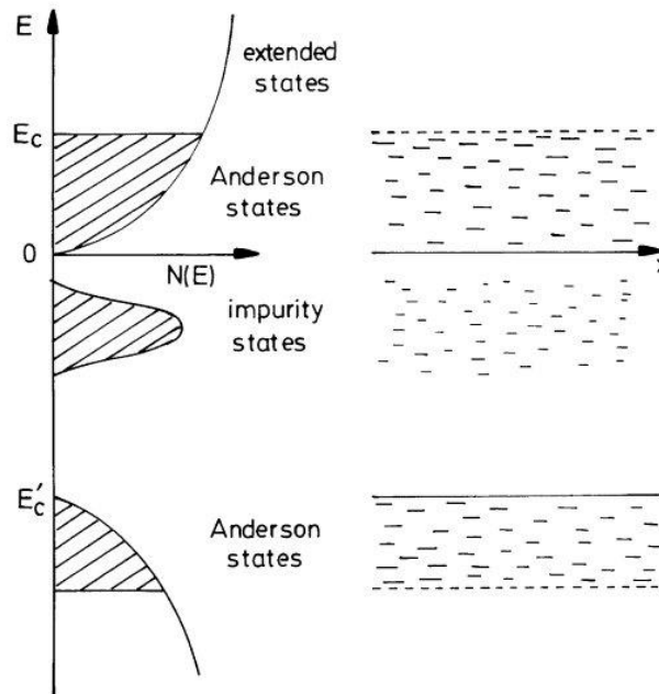
Figure I.10 – Schéma de la densité d'états électroniques localisés dans la bande interdite théorique, dissociant pour des raisons de clarté les pièges physiques (d'Anderson) des pièges chimiques. Reproduction de [49].
