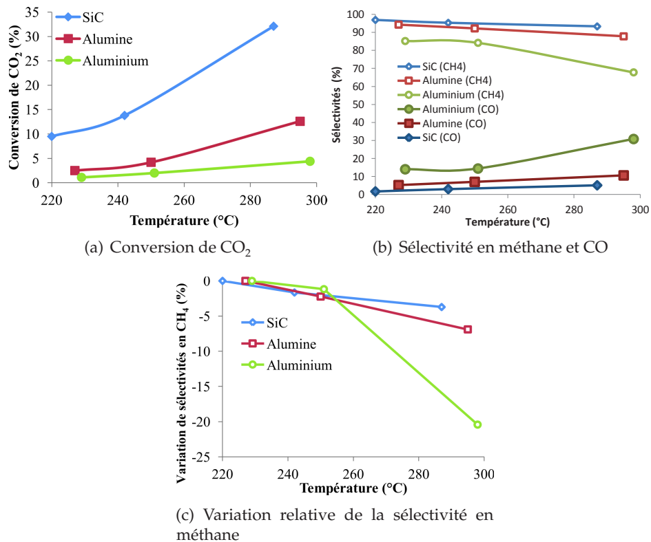
Figure 4.7 Résultat des tests catalytiques réalisés dans le réacteur sans hublot à 2 \text{ L h}^{-1} en fonction du support de catalyseur utilisé (SiC, alumine et aluminium)
