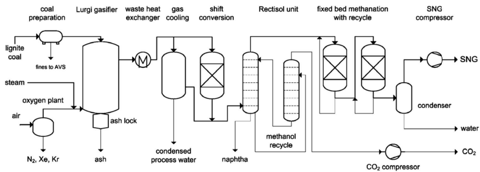
Figure 1.13 Procédé Lurgi 22
