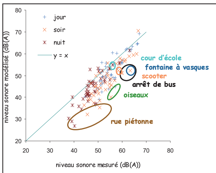
Figure 39 : Distribution des niveaux sonores mesurés et modélisés (dB(A)), pour le jour, le soir et la nuit, pour les 44 logements retenus pour l'étude, et sources sonores identifiées à proximité des logements
