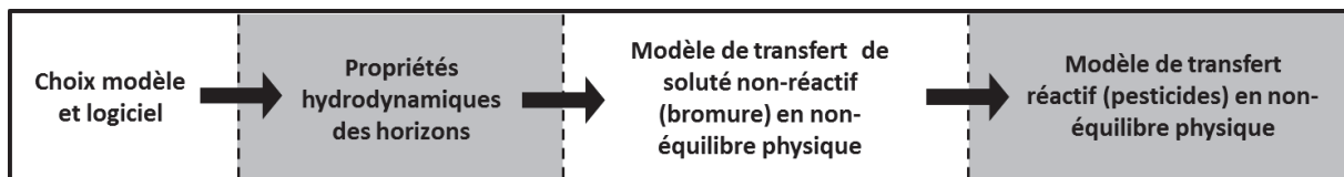
Figure 70 : diagramme de l'approche de modélisation à complexité croissante adoptée
