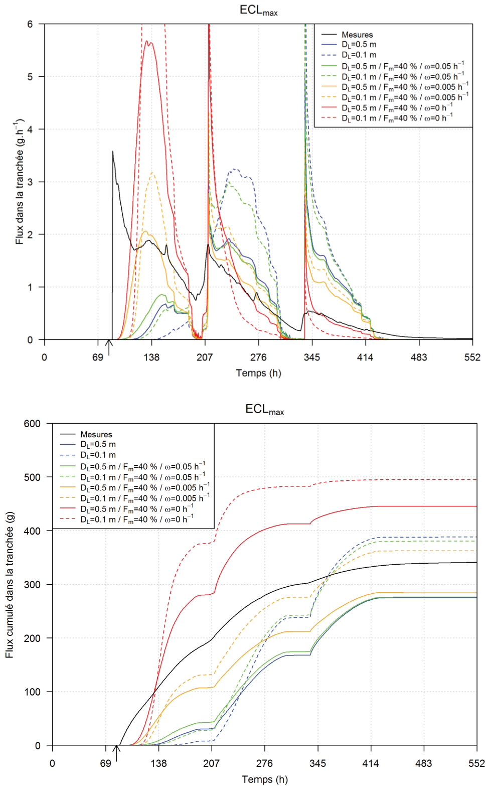
Figure 88 : flux mesuré et flux simulés, cumulés et instantanés, de soluté dans la tranchée pour 1) les scénarios ECL_{max} avec F_m = 40\% , pour l'ensemble des variantes sur \omega et sur la dispersivité, et 2) les scénarios ECL_{max} et F_m = 100\% (en bleu)
