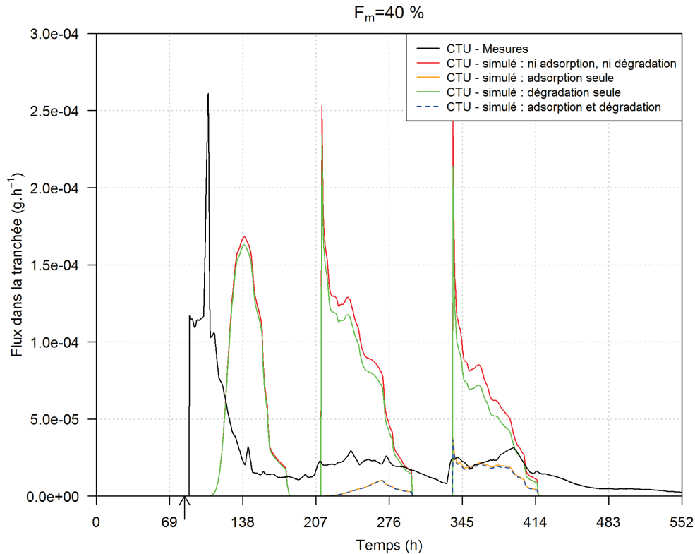
Figure 91 : flux mesurés et simulés pour le chlortoluron, selon les processus pris en compte. Les courbes bleue et orange sont quasiment identiques
