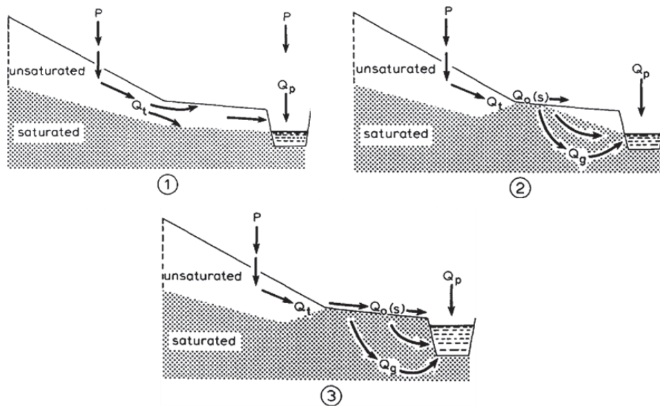
Figure 6 : illustration de la succession des phases d'écoulements, pour un versant très perméable qui subit un événement pluvieux, par Ward (1984)
