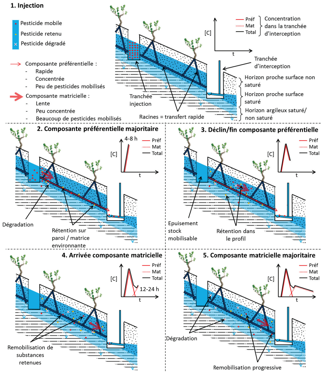
Figure 95 : modèle conceptuel du transfert lors du traçage, mettant en jeu les deux composantes de l'écoulement identifiées
