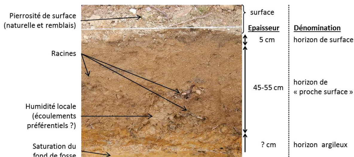
Figure 27 : fosse pédologique montrant le profil du sol en aval de la parcelle, quelques caractéristiques et éléments remarquables. Photographie prise le lendemain de l'ouverture de la fosse, après un événement pluvieux : au fond de la fosse, dans l'horizon argileux, subsiste une flaque d'eau provoquée par les écoulements latéraux
