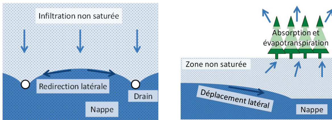
Figure 9 : à gauche, illustration de l'écoulement latéral se produisant entre deux drains ; à droite, illustration de l'écoulement latéral provoqué par une évapotranspiration marquée
