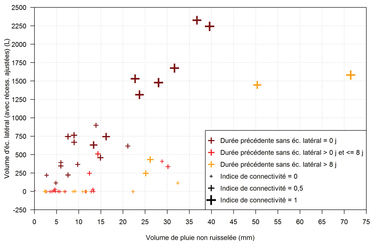
Figure 53 : volume évènementiel d'écoulement latéral selon le volume de pluie, la durée précédente sans écoulement latéral, et l'indice de connectivité. La taille des croix des évènements est variable et représente la valeur exacte de leur indice de connectivité (il ne s'agit pas de classes)
