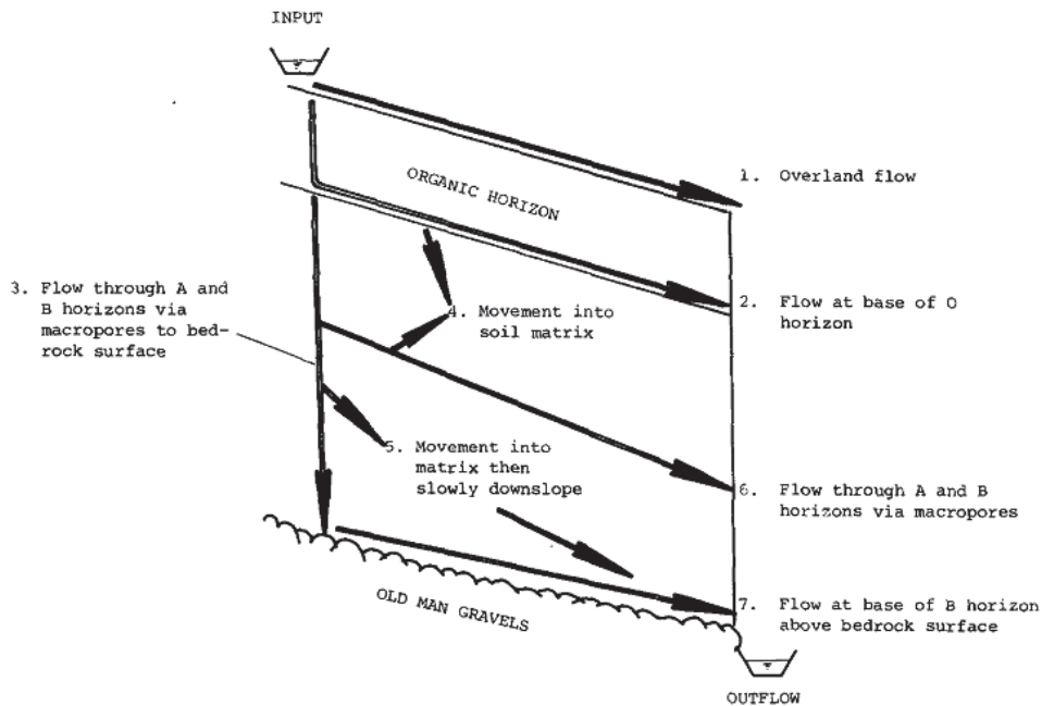
Figure 7 : vue schématique des chemins empruntés par l'eau dans le sol (dans et d'après Mosley (1982))
