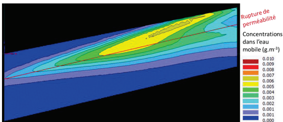
Figure 92 : champ des concentrations final (après 23 j) en chlortoluron dans l'eau mobile
