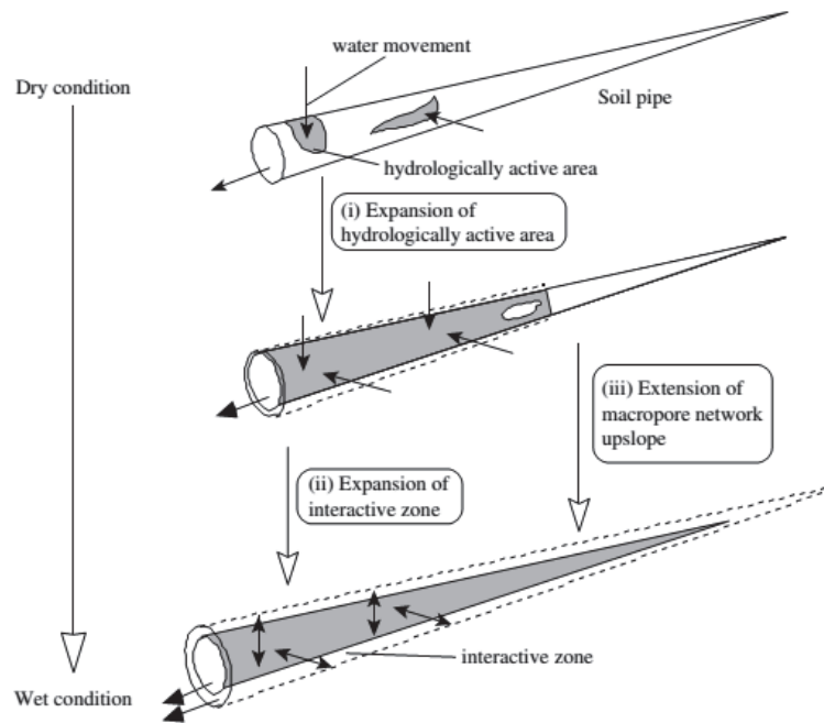
Figure 12 : modèle d'extension de l'activité hydrique d'un conduit tubulaire selon son état d'humidité, tiré de Uchida et al. (2001)
