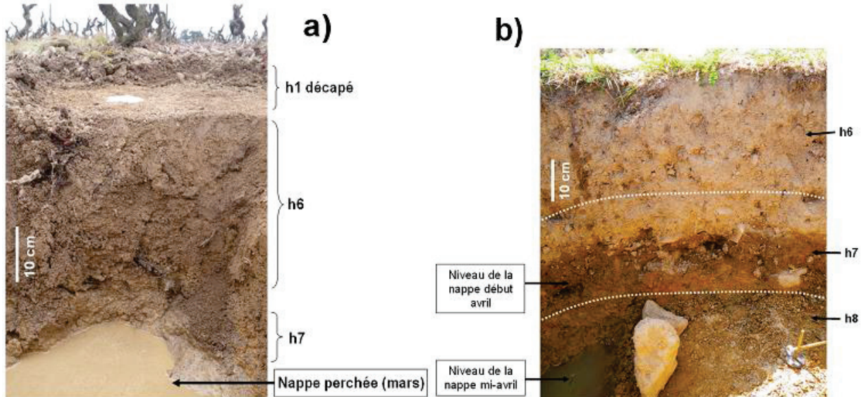
Figure 102 : a) Nappe perchée dans une fosse (mars). b) Nappe perchée dans une fosse (avril)
