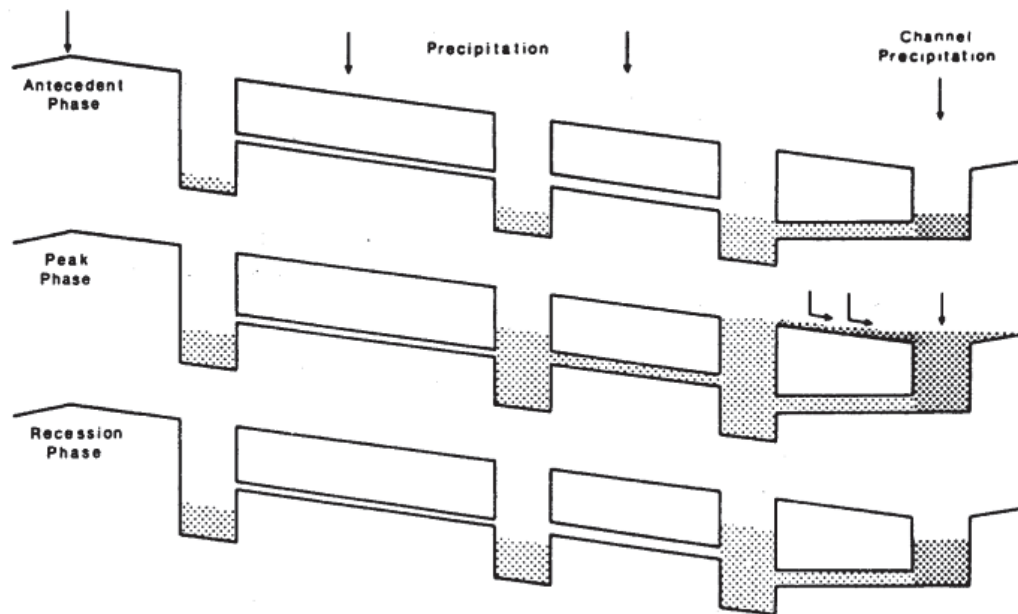
Figure 5 : illustration de la variabilité de la surface contributive amont pour l'écoulement latéral. D'après Hewlett et Nutter (1970)
