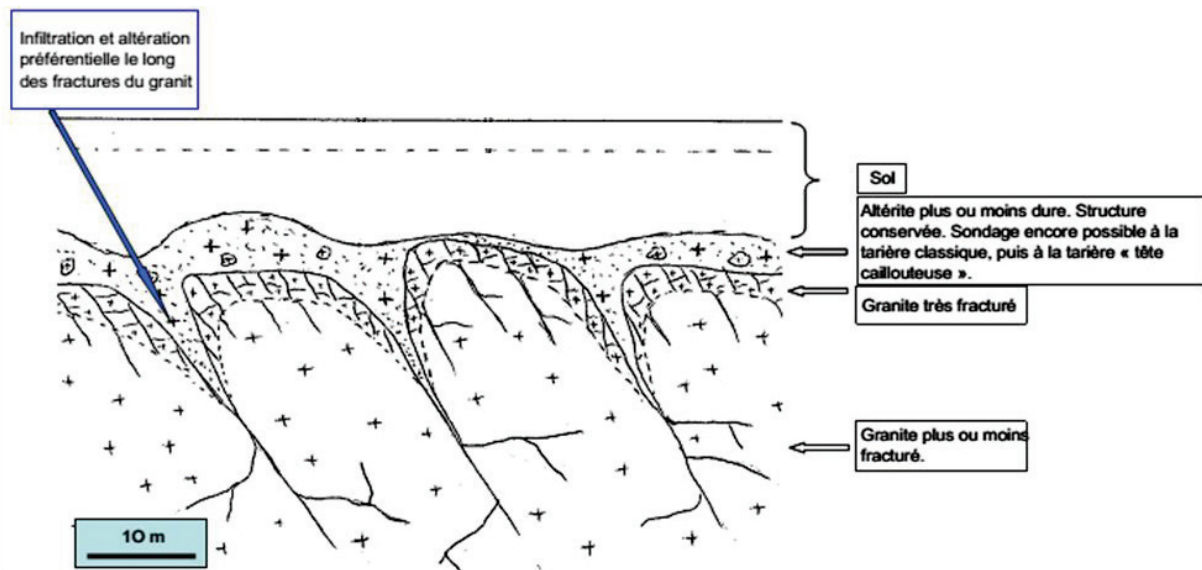
Figure 21 : schéma interprétatif de la morphologie de l'altérite en relation avec le processus d'altération préférentielle du granite. Tiré de Van den Bogaert (2011)
