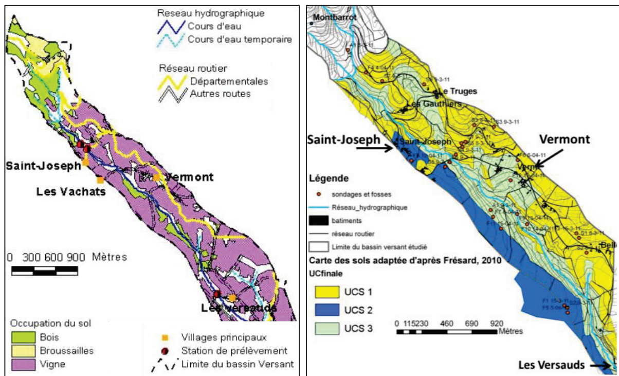
Figure 19 : à gauche, carte d'occupation des sols, source IGN, issue de Escot (2005). À droite, unités cartographiques de sols, d'après Van den Bogaert (2011)
