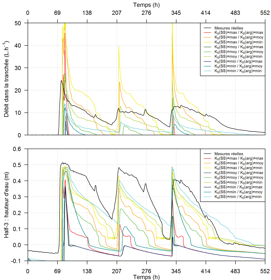
Figure 85 : débit dans la tranchée et hauteur d'eau dans le piézomètre Half-3, pour les scénarios portant sur les propriétés hydrodynamiques des horizons. Dans la légende, « SS » fait référence à l'horizon de proche surface, et « arg » à l'horizon argileux
