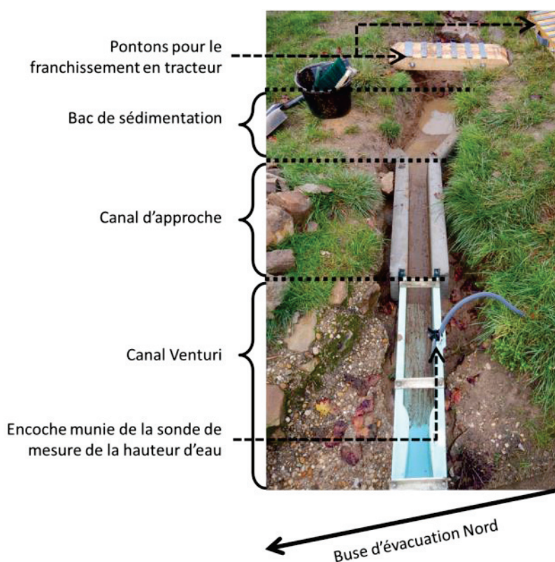
Figure 35 : photographie illustrée de l'installation pour la mesure du ruissellement
