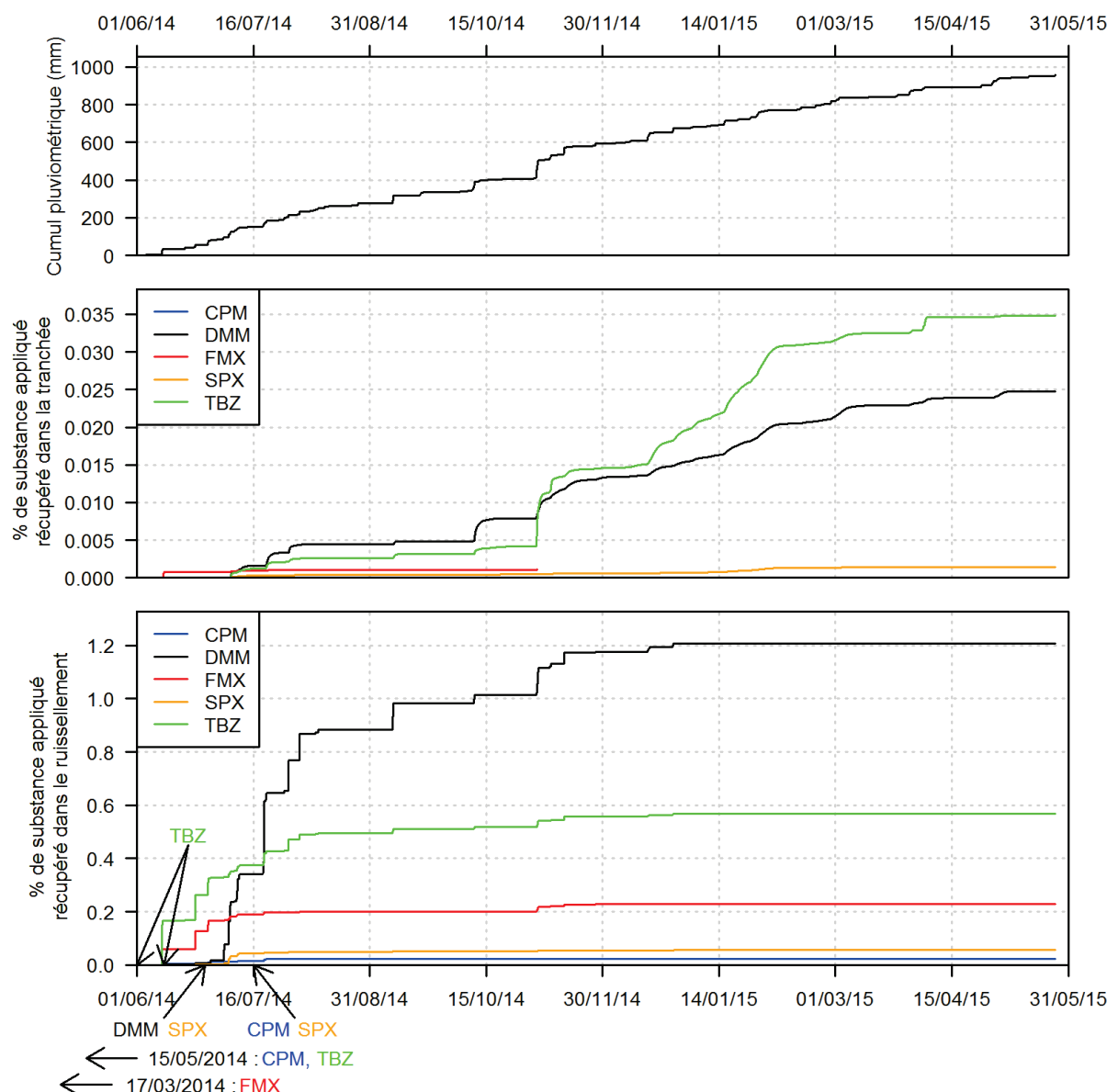
Figure 63 : pluviométrie et pourcentages de récupération des pesticides appliqués pour l'écoulement latéral et le ruissellement, pour chacune des substances étudiées à l'échelle du suivi de l'année culturale 2014. Pour l'écoulement latéral, les données exposées ici correspondent à l'hypothèse d'une surface contributive élevée (3 m × 70 m). Pour l'hypothèse d'une surface contributive faible (3 m × 35 m), les pourcentages de récupération sont à multiplier par deux
