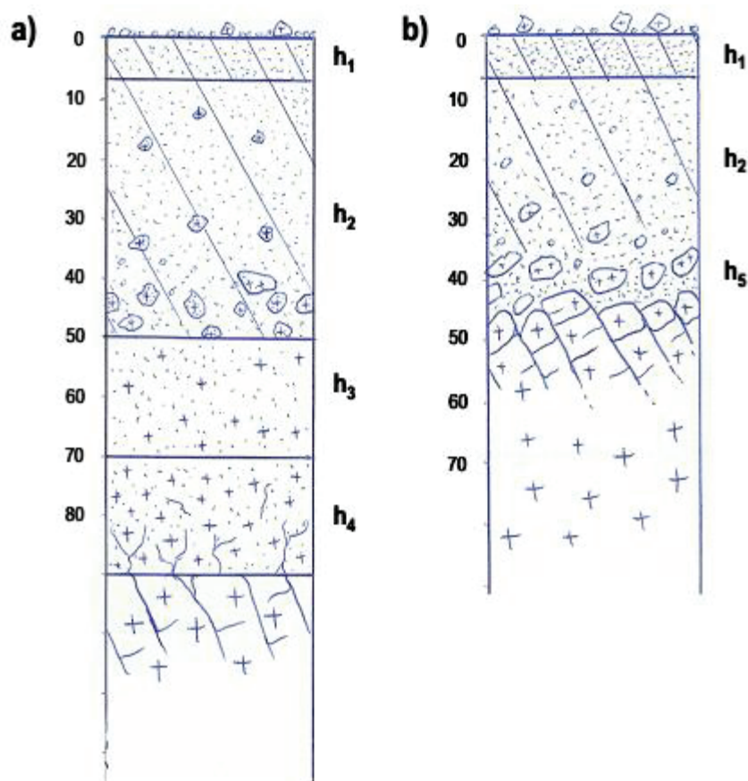
Figure 97 : a) Organisation type des sols sableux sur altérite (UTS 1) ; b) Organisation type des sols sableux sur granite fracturé (UTS 2)
