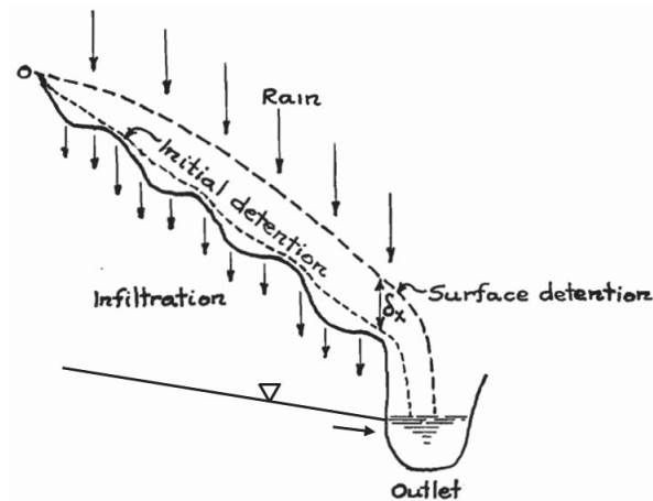
Figure 2 : demi-section d'un petit bassin versant illustrant la théorie de l'infiltration (l'échelle verticale est exagérée). Adapté de Horton (1945)
