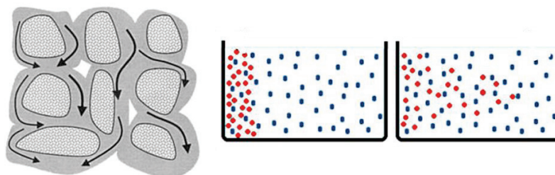
Figure 1 : à gauche, illustration de la dispersion hydrodynamique dans le sol. Au centre et à droite, illustration de la diffusion moléculaire
