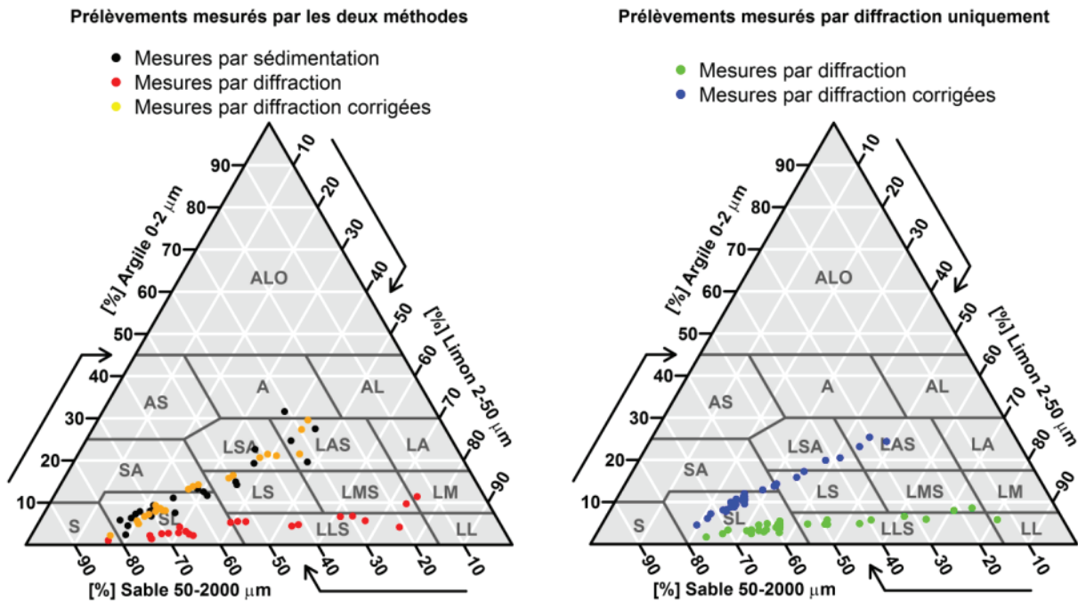
Figure 24 : triangles des textures de l'Aisne. À gauche, comparaison des mesures par sédimentation, par diffraction, et les résultats des mesures corrigées, pour les prélèvements analysés selon les deux méthodes. À droite, comparaison des mesures par diffraction et les résultats des mesures corrigées pour les prélèvements uniquement analysés par diffraction
