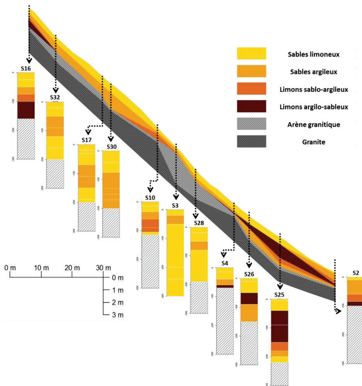
Figure 26 : toposéquence du versant, au niveau de la partie Nord, sur toute la longueur de la parcelle.
