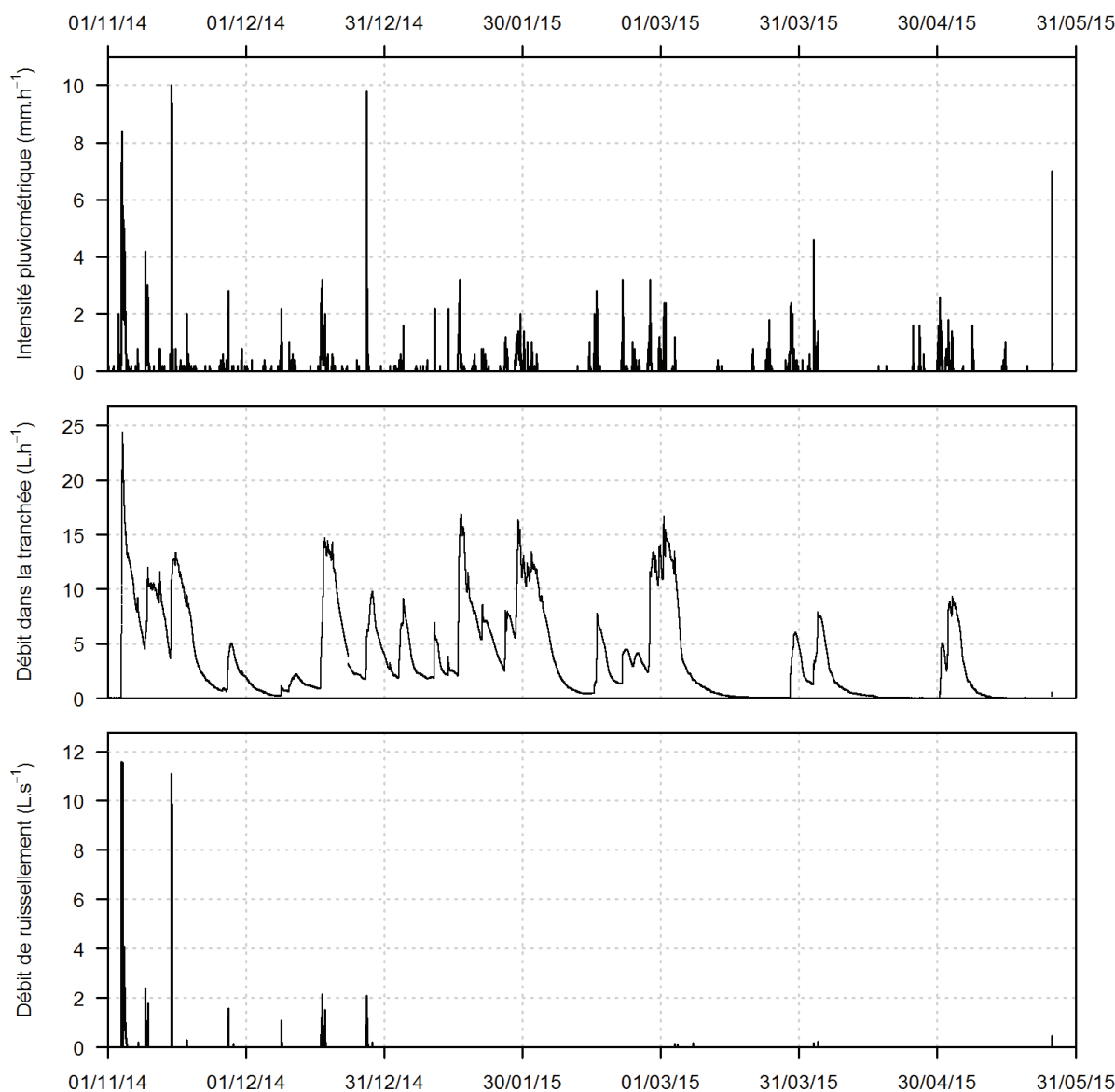
Figure 42 : pluviométrie horaire, débit d'écoulement latéral mesuré dans la tranchée, et débit de ruissellement mesuré dans le canal Venturi, pour la période allant du 1 er novembre 2014 au 31 mai 2015
