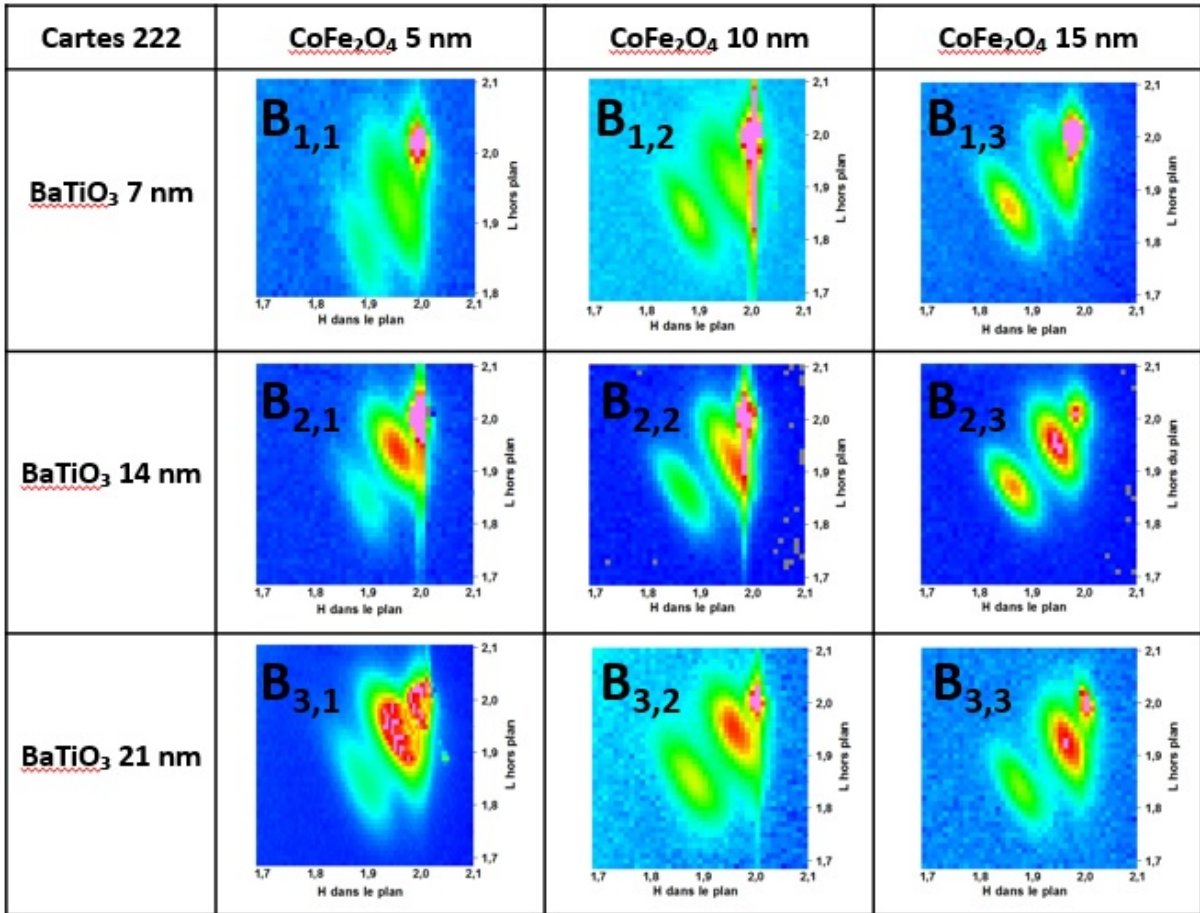
Figure 35: Cartes HKL autour du pic asymétrique 222 dans l'espace réciproque pour les échantillons de la série B. L'abscisse H indexe le paramètre dans le plan, et l'ordonnée L le paramètre hors du plan. H et L sont donnés en unités du réseau réciproque du substrat SrTiO 3 (001). Les coordonnées des cartes sont indexées entre 1.7 et 2.1 dans les deux directions, avec la coordonnée (H=K ; L) = (2.0 ; 2.0) correspondant au pic de Bragg du substrat SrTiO 3 .
