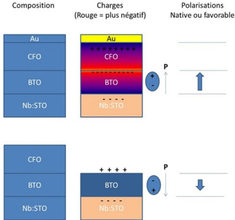
Figure 56: Représentation schématique de la polarisation électrique intrinsèque au sein de la couche de BaTiO 3 dans la configuration CoFe 2 O 4 / BaTiO 3 / SrTiO 3 et BaTiO 3 / SrTiO 3 .
