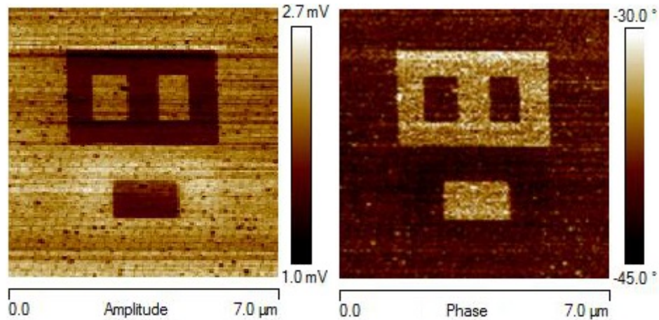
Figure 58: Images PFM de phase (gauche) et d'amplitude (droite) d'un échantillon de 5 nm de \text{CoFe}_2\text{O}_4 sur 14 nm de \text{BaTiO}_3 sur substrat \text{Nb}:\text{SrTiO}_3(001) . Images obtenues le lendemain de l'écriture à \pm 8\text{V} du motif de type smiley.
