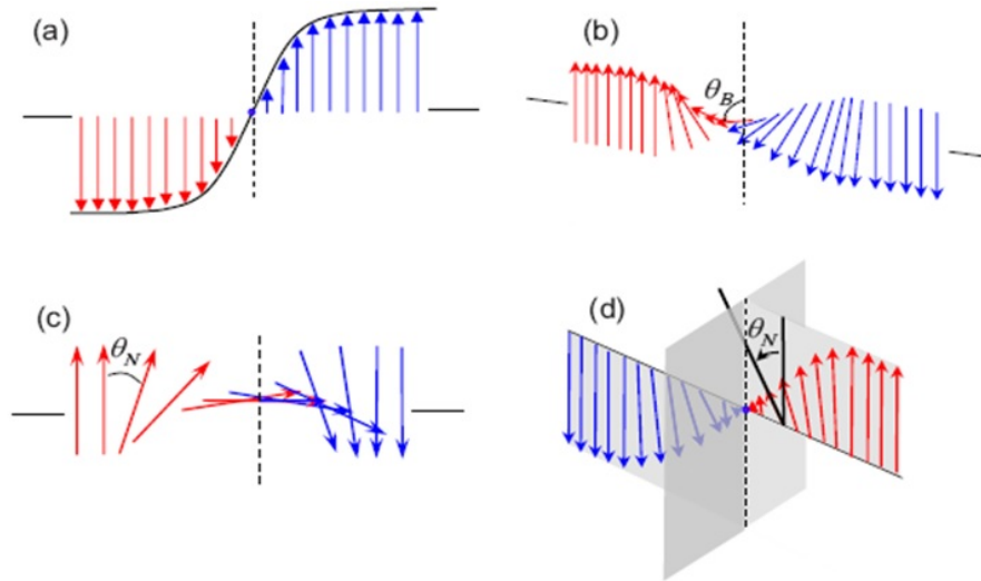
Figure 3: Différents types de parois de domaines. (a) Ising (b) Bloch (c) Néel (d) Mélange Ising-Néel. D'après [3].
