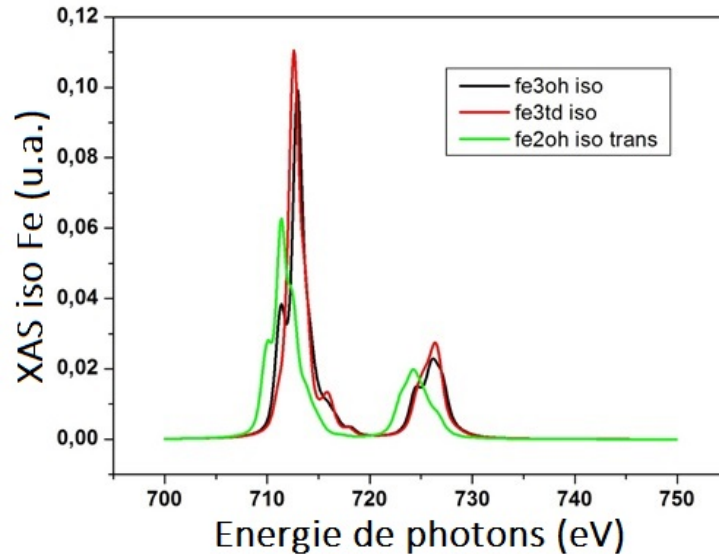
Figure 87: Courbes XAS théoriques calculées par P. Saintavrit pour les ions \text{Fe}^{3+} et \text{Fe}^{2+} en sites octaédriques et tétraédriques.
