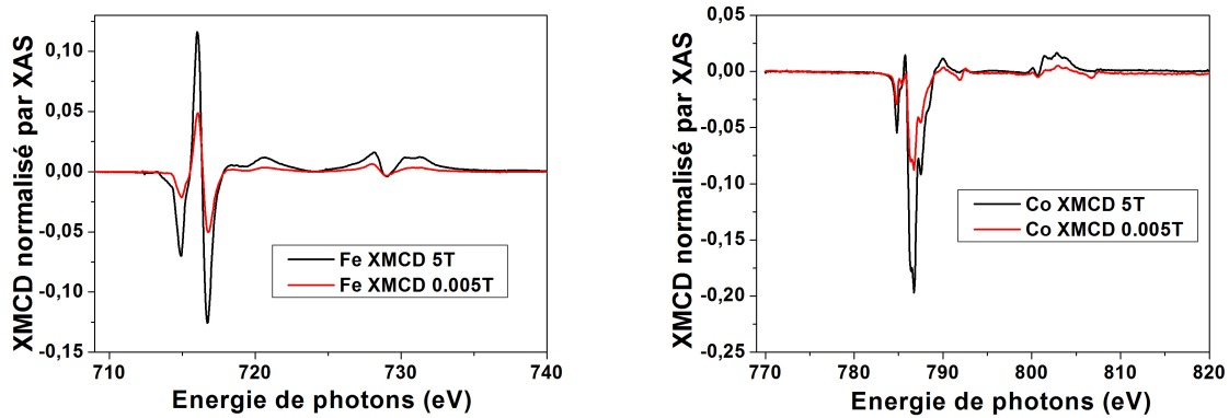
Figure 47: Echantillon A 1,3 de 6.6 nm de CoFe 2 O 4 sur 7 nm de BaTiO 3 . Signal XMCD réalisé à 4K sous un champ saturant de 5T et à 0.005T à rémanence des pics L 2,3 du Fe (gauche) et L 2,3 du Co (droite).
