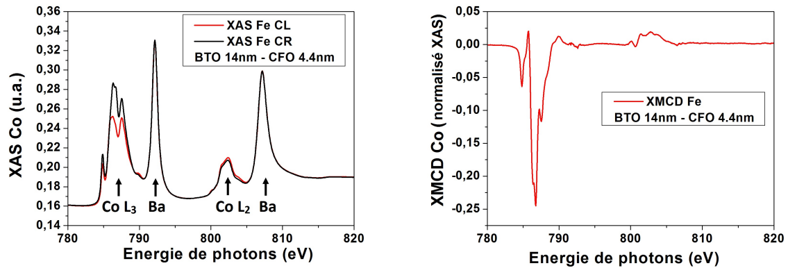
Figure 46: Exemple de spectres d'absorption réalisés à 4K sous un champ saturant de 5T et de dichroïsme circulaire pour un échantillon de 4.4 nm de \text{CoFe}_2\text{O}_4 sur 14 nm de \text{BaTiO}_3 ( A_{2,2} ). A gauche : spectres de spectroscopie d'absorption XAS montrant les seuils L_{2,3} du Co, pour les polarisations circulaire gauche (CL) et circulaire droite (CR). A droite : spectre XMCD associé normalisé au XAS.
