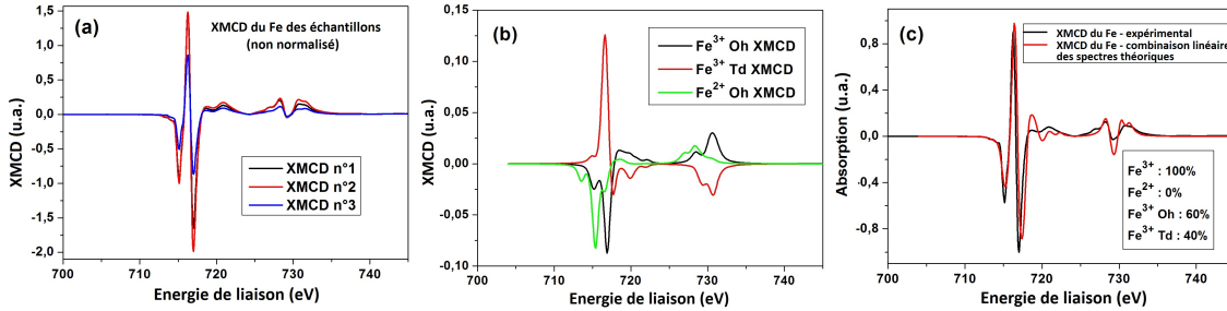
Figure 29: (a) Spectres XMCD expérimentaux autour des seuils L_{2,3} du Fe dans les échantillons décrits dans le tableau 2 (b) Spectres XMCD théoriques pour Fe^{3+} Oh , Fe^{3+} Td et Fe^{2+} Oh (c) Spectre XMCD expérimental d'un des échantillons approché par méthode des moindres carrés à partir des spectres théoriques
