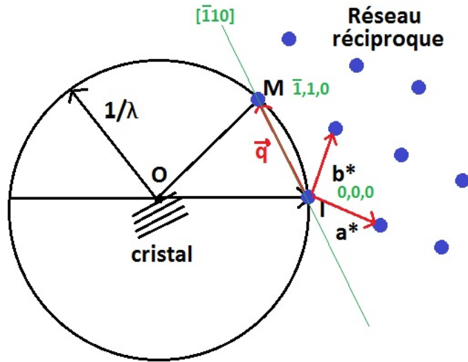
Figure 16: Sphère d'Ewald
