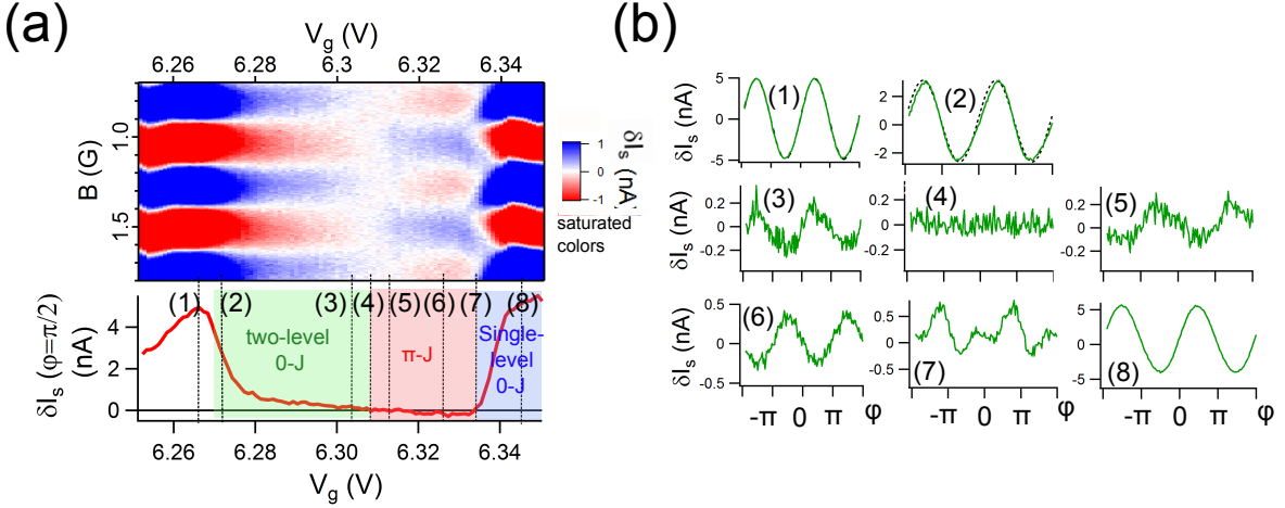
FIGURE 3 – (a) Modulation du courant de switching du SQUID en fonction du champ magnétique, quantité proportionnelle à la relation courant phase, en fonction de la tension de grille V_g dans le diamant de Coulomb correspondant à une occupation N=3 . Le supercourant à la transition étant très petit, l'échelle de couleur est saturée. En dessous est tracé le supercourant à une phase de \varphi = \pi/2 fixée en fonction de V_g . (b) Relation courant phase aux tensions de grilles indiquées sur le graphe 2D. On peut remarquer qu'à la transition (4), le courant critique s'annule, et pas à la transition (7).
