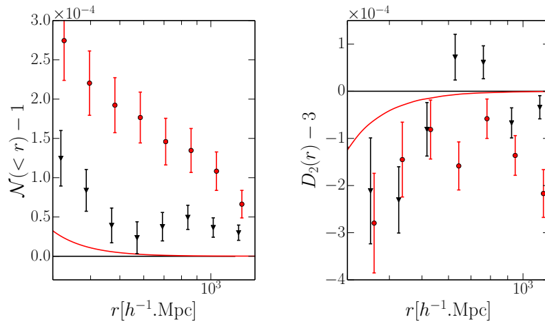
FIGURE 4.17 Mesures de \widehat{\mathcal{N}}^{\text{LS}}(<r) et \widehat{D}_2^{\text{LS}}(r) pour la matière pour le NGC d'eBOSS (en noir) et le SGC d'eBOSS (en rouge).
