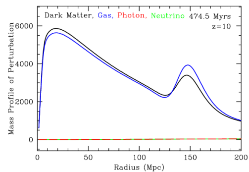
(F) Les profils de densité de matière noire et de matière baryonique sont équilibrés.
