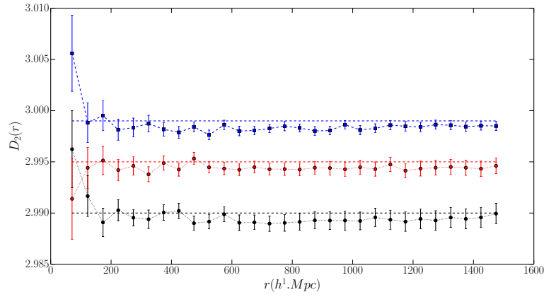
FIGURE 4.10 Valeurs de D_2(r) moyennes obtenues pour les simulations brutes (c'est-à-dire, sans appliquer la géométrie du relevé.), pour D_2 = 2,99, 2,995, \text{ et } 2,999 (soit p = 0,9931, 0,9965, \text{ et } 0,9993 ). L'erreur correspond à l'écart type entre les 200 simulations.
