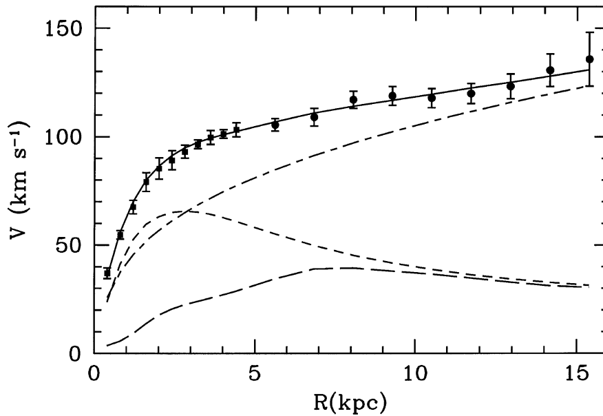
FIGURE 1.4 Courbe de rotation de la galaxie M33, obtenue à partir de la mesure de la raie 21-cm de l'hydrogène (points noirs) [13]. La ligne en pointillés courts représente la vitesse attendue si la galaxie n'était composée que d'étoiles, la courbe en pointillés longs représente la contribution du gaz et la courbe en pointillés courts et longs la contribution du Halo. La courbe noire représente la somme de toutes les contributions.
