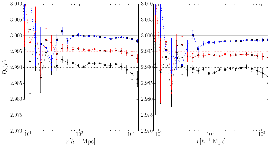
FIGURE 4.12 Valeur moyenne de D_2 reconstruite avec l'estimateur \widehat{D}_2^{\text{PH}}(r) (à gauche) et \widehat{D}_2^{\text{LS}}(r) (à droite) pour 200 simulations après analyse. Les erreurs sont obtenues à partir de la déviation standard des 200 simulations. Les courbes pointillées correspondent à la valeur de D_2 initialement simulée.
