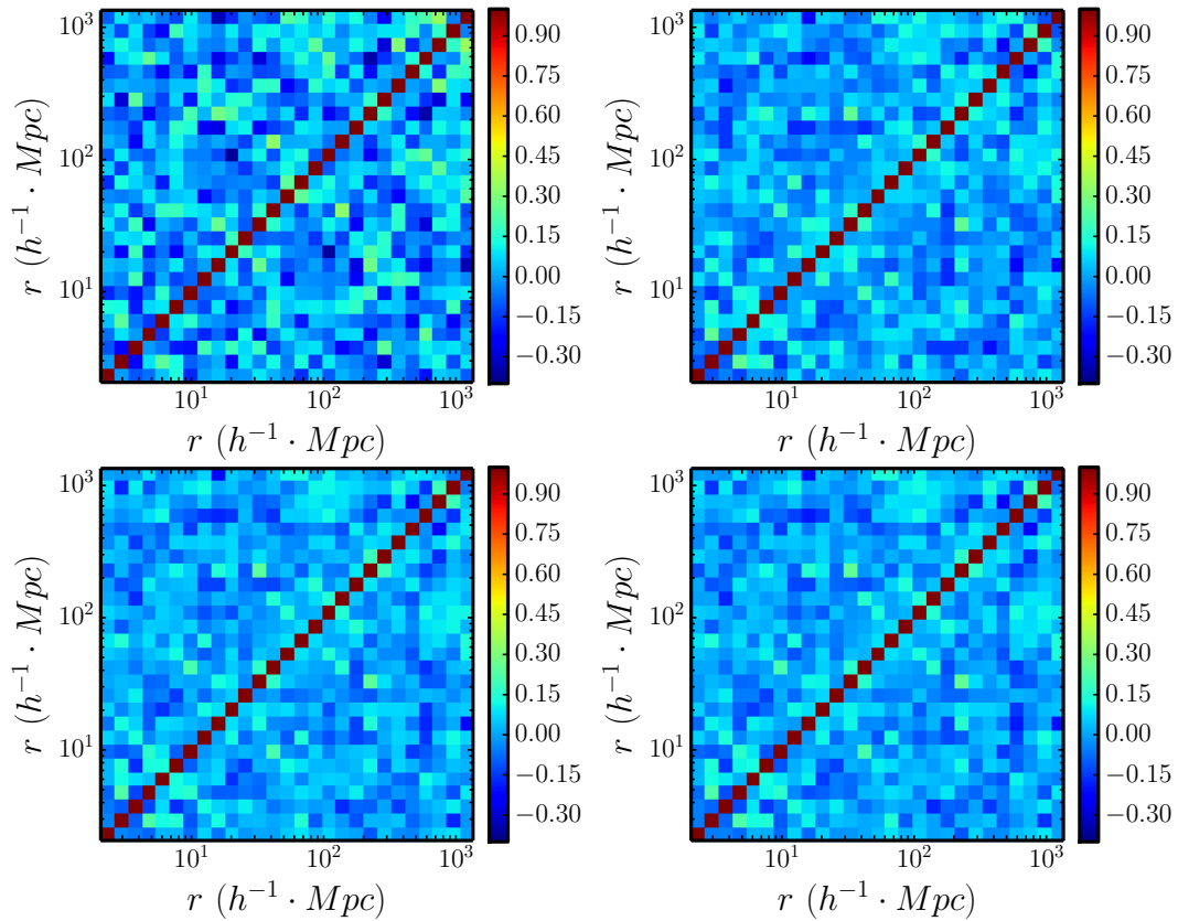
FIGURE 3.10 De gauche à droite et de haut en bas : matrice de corrélation du relevé BOSS (après traitement des effets systématiques) avec 100, 1000, 10^4 et 10^5 réalisations de bootstraps (avec 201 cellules).
