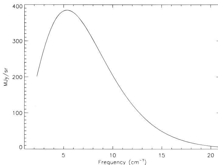
FIGURE 1.3 Spectre de corps noir mesuré par l'instrument FIRAS de l'expérience COBE [8]. Les incertitudes sont si petites qu'elles ne dépassent pas l'épaisseur de la courbe, ajustée aux données, d'un spectre de corps noir.
