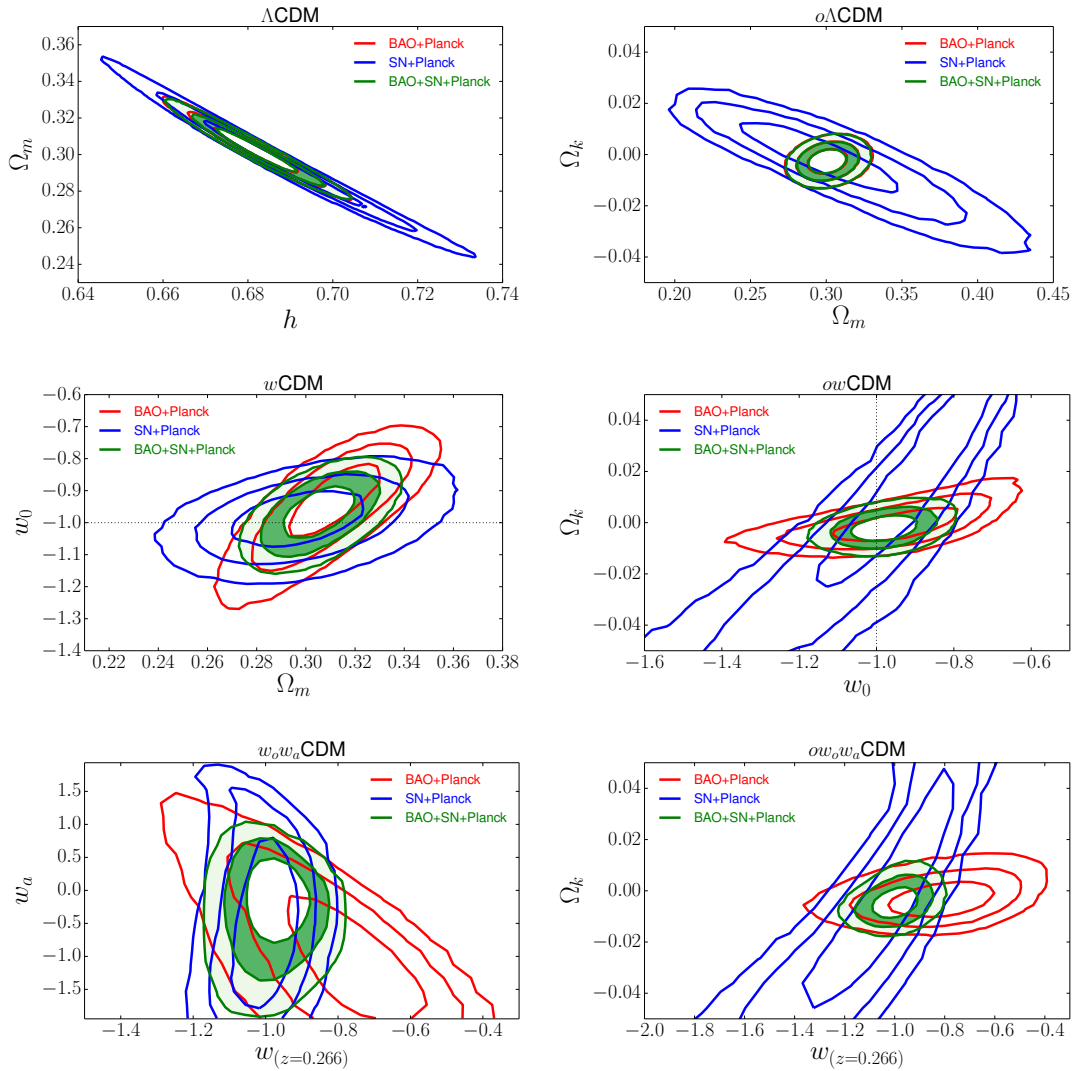
FIGURE 5.4 Contraintes cosmologiques pour différents modèles d'énergie noire, obtenues à l'aide des données BAO, Planck et des supernovæ. Les différents contours correspondent aux contours de confiance à 68 %, 95 % et 99,7 %. On note que les mesures de supernovæ et de BAO sont très complémentaires pour contraindre les paramètres cosmologiques des différents modèles d'énergie noire, tout particulièrement quand la courbure de l'univers est laissée libre [119].
