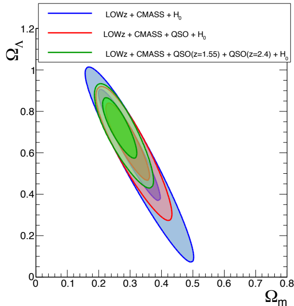
FIGURE 5.10 Contraintes pour le modèle \Lambda CDM dans le plan \Omega_m - \Omega_\Lambda obtenues en combinant la mesure de \alpha_{iso} , les mesures de distances des galaxies LOWZ, CMASS BOSS et de eBOSS, et la mesure locale de H_0 .
