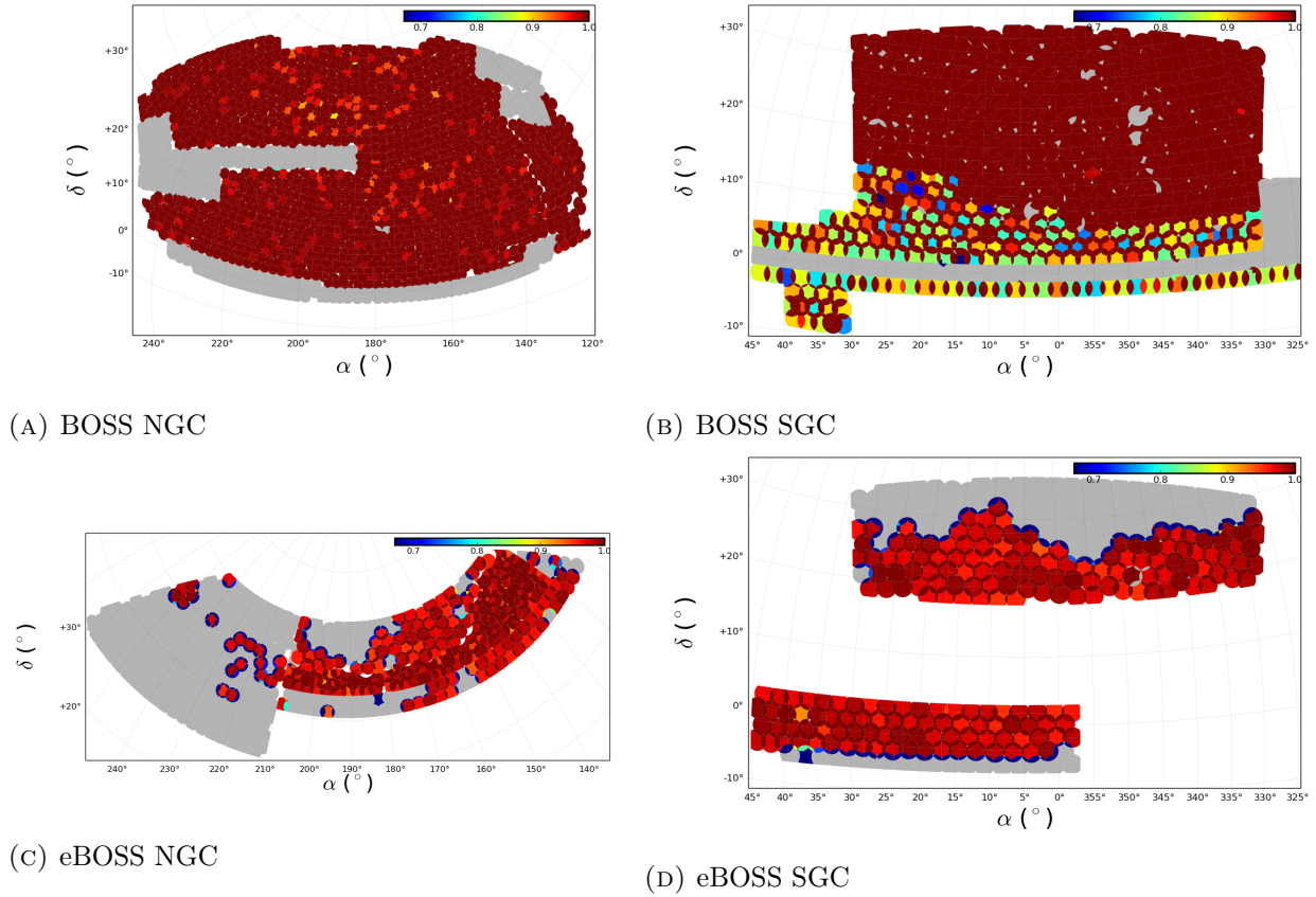
FIGURE 3.1 Complétude du relevé BOSS et eBOSS. Les zones dans le SGC de BOSS avec une complétude plus faible aux centres de plaques correspond aux chunks 12 et 13 dans lesquels les cibles galaxies ont la priorité sur les cibles quasars en cas de collisions. Pour le NGC d’eBOSS, on voit clairement se détacher une zone où la complétude est plus élevée : cette zone correspond au relevé SEQUELS, dont les plaques étaient plus proches que pour le reste du relevé eBOSS. La probabilité qu’une cible quasar soit située sur plus d’une plaque est plus élevée, d’où la complétude plus importante du relevé SEQUELS.
