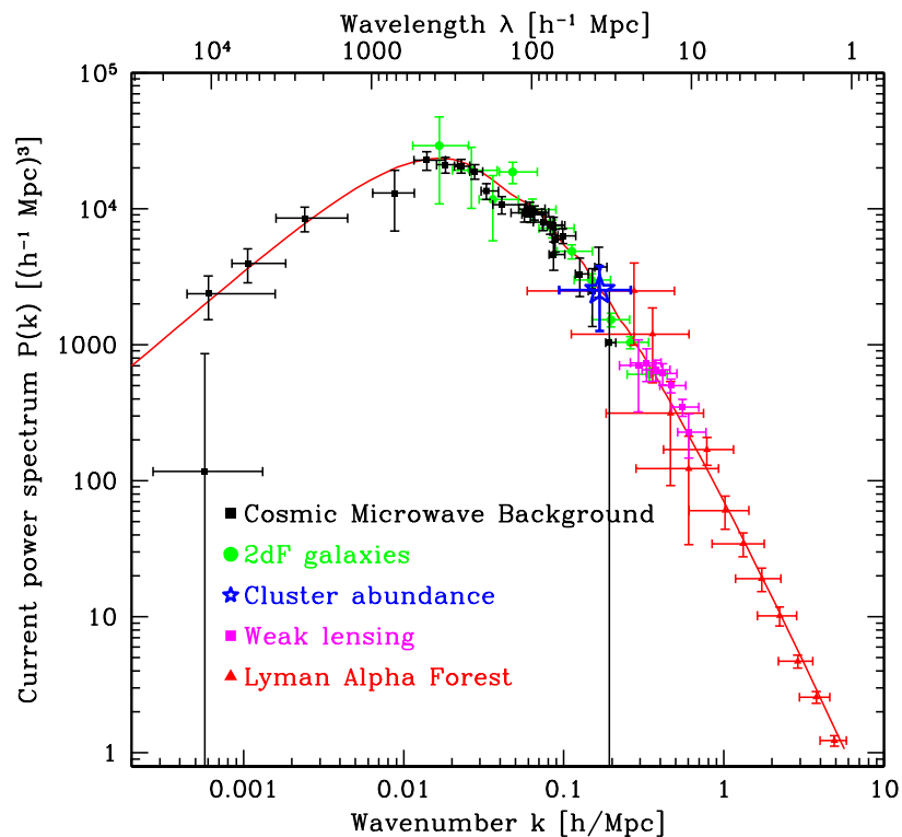
FIGURE 1.9 Combinaison de différentes sondes pour la mesure du spectre de puissance de la matière [20]. La courbe rouge provient d'un ajustement d'un spectre de puissance linéaire sur l'ensemble des données.
