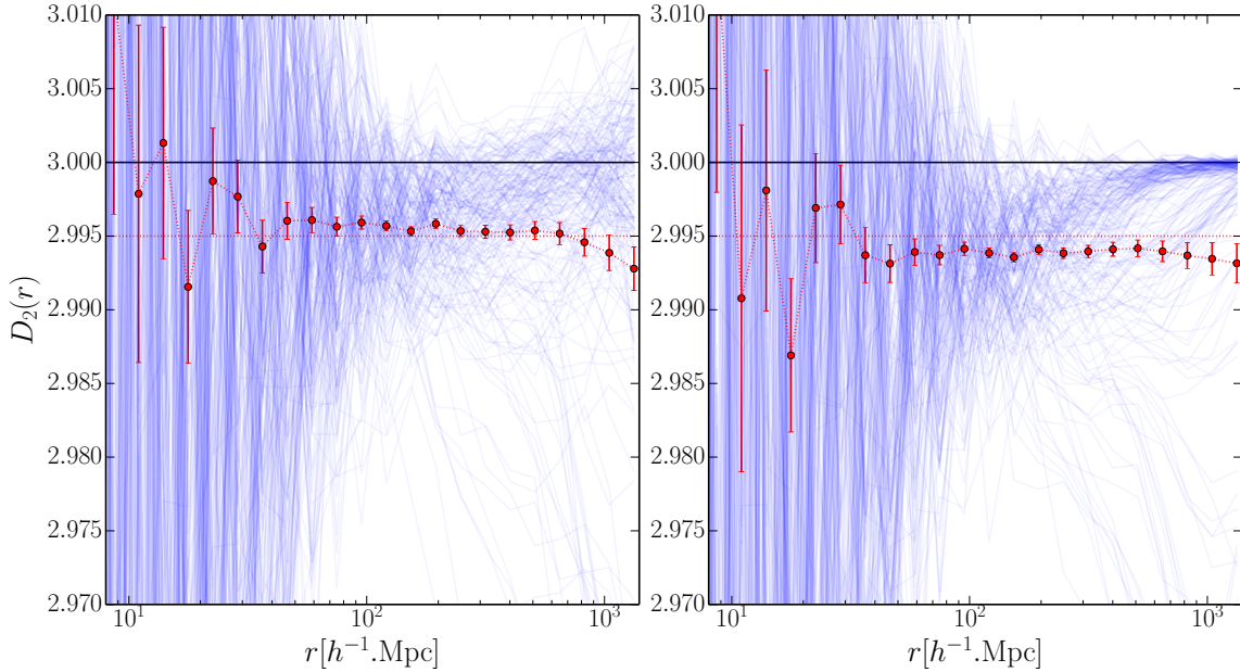
FIGURE 4.13 Ensemble des mesures de \widehat{D}_2^{\text{PH}}(r) et \widehat{D}_2^{\text{LS}}(r) pour chacune des 200 simulations, toutes simulées avec D_2 = 2,995 .
