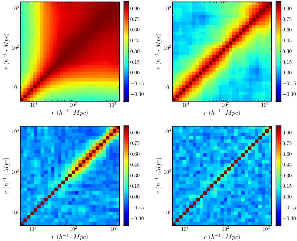
FIGURE 4.7 Matrices de corrélation pour \widehat{\mathcal{N}}^{\text{PH}}(< r) et \widehat{D}_2^{\text{PH}}(r) (en haut), et pour \widehat{\mathcal{N}}^{\text{LS}}(< r) et \widehat{D}_2^{\text{LS}}(r) (en bas) pour le relevé eBOSS (NGC + SGC), après correction des effets systématiques.
