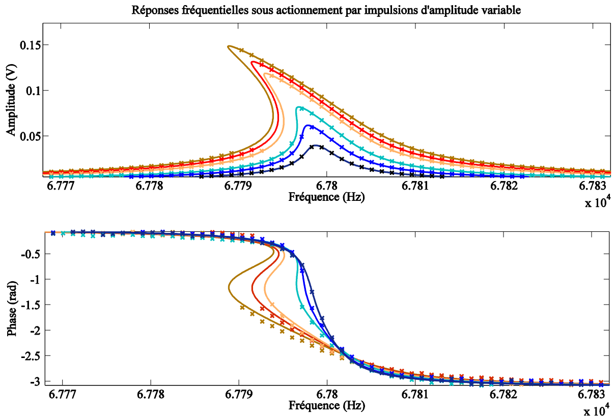
Fig. 53 Résultats expérimentaux sur 5 séries de mesures de réponses fréquentielles pour des tensions d'actionnement croissantes (de bleu à brun).
