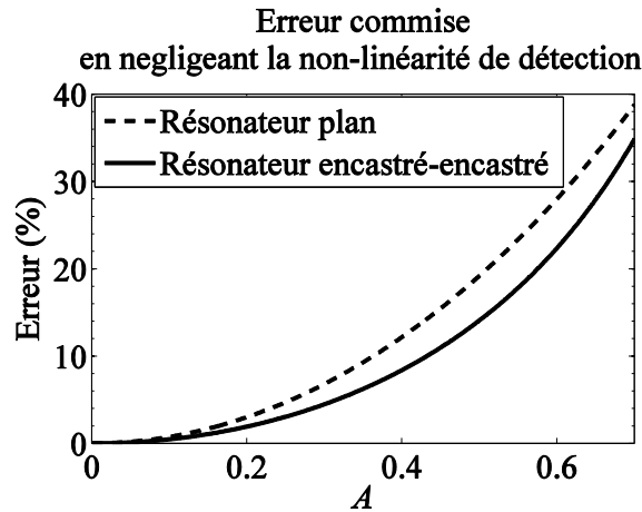
Fig. 80 Erreur commise en approximant la détection par une détection linéaire pour un pont vibrant et comparaison avec un résonateur plan.
