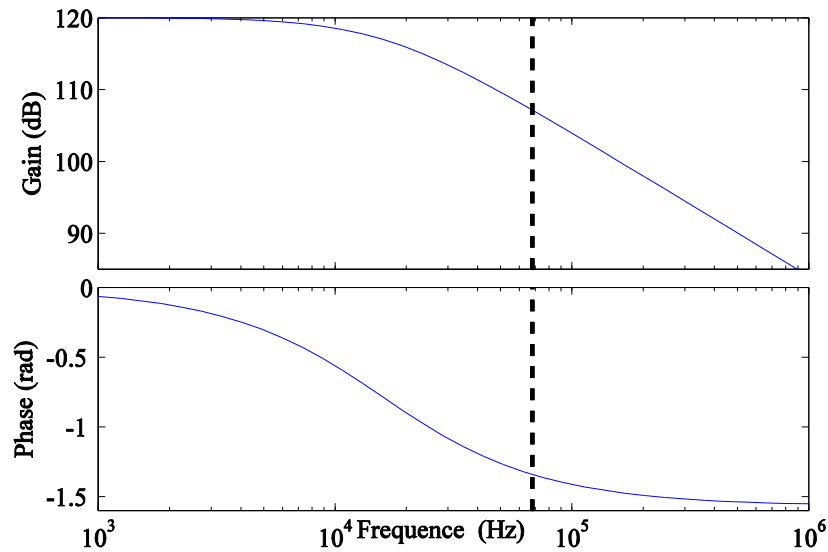
Fig. 12 Diagramme de bode de l'amplificateur de charge utilisé pour la détection. La fréquence de travail est représentée par le trait pointillé.
