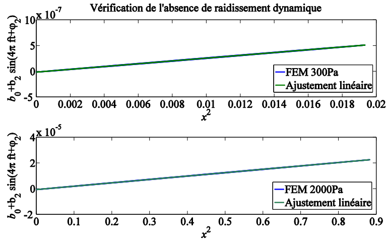
Fig. 86 Simulations non-linéaires transitoires par éléments finis: Evolution de la composante statique et de la composante dynamique à 2\omega du déplacement axial en fonction du déplacement du centre de la poutre.
