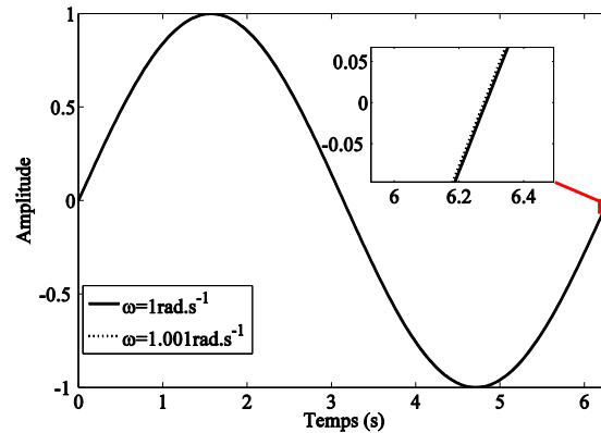
Fig. 37 Illustration du problème de détermination de la fréquence instantanée pour un résonateur à haut facteur de qualité : Différence, sur une période, entre deux signaux sinusoïdaux d'amplitude unitaire et de fréquences proches à \pm 1\% (pulsations de 1\text{rad.s}^{-1} et de 1,001\text{rad.s}^{-1} ).
