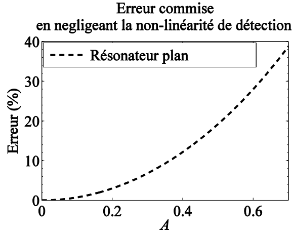
Fig. 79 Erreur commise en approximant la détection par une détection linéaire pour un résonateur plan.
