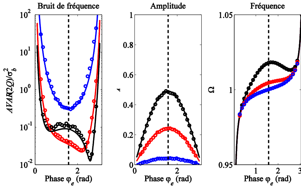
Fig. 69 Evolution de la variance des fluctuations de fréquence pour un résonateur à non-linéarité cubique fortement non-linéaire ( \gamma Q > 1 ) actionné par des forces d'amplitude croissante et soumis à un bruit blanc additif. Les lignes continues correspondent à l'équation (252). Les cercles correspondent à des simulations en régime transitoire effectuées dans les mêmes conditions.
