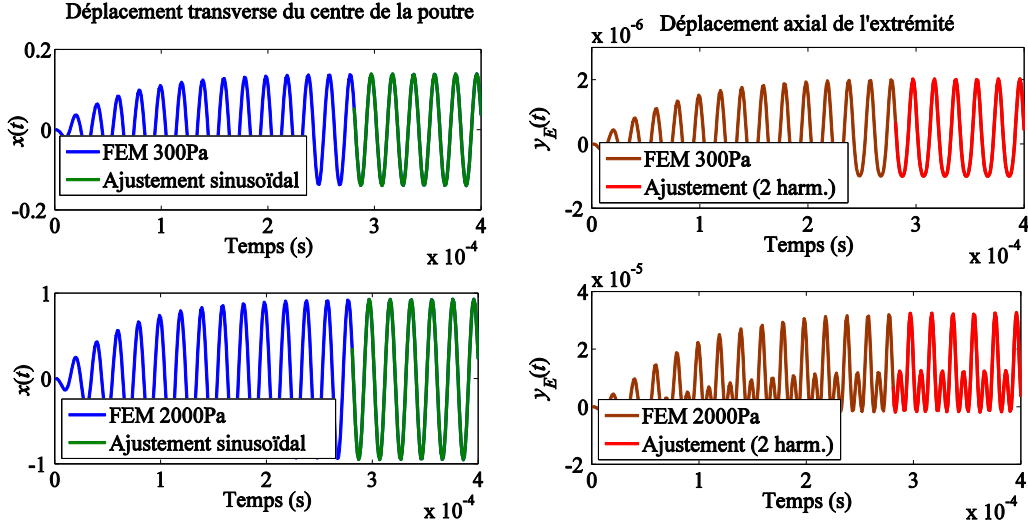
Fig. 85 Simulations non-linéaires transitoires par éléments finis pour deux pressions d'amplitudes différentes. Gauche : Mouvement transverse normalisé du centre de la poutre et ajustements x(t) = A \sin(\omega t + \varphi) . Droite : Mouvement axial normalisé de l'extrémité imparfaitement encastree et ajustement par y_e(t) = b_0 + b_1 \sin(\omega t + \varphi_1) + b_2 \sin(2\omega t + \varphi_2) .
