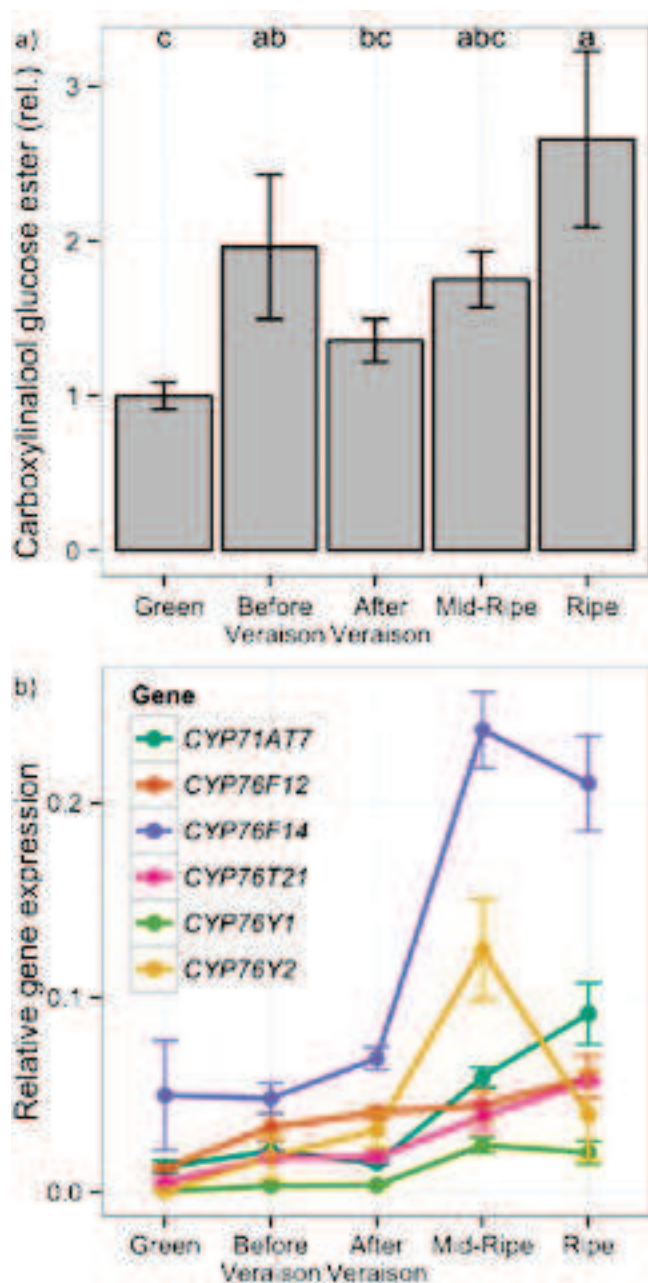
Figure 5. Evolution de la concentration en ester de glucose de (E)-8-carboxylinalool et de l'expression des gènes candidats pendant la maturation de baies de raisin. a) Concentration relative ( \pm écart type) du glucose ester de (E)-8-carboxylinalool pendant le développement des baies de Gewurztraminer. L'analyse de variance monofactorielle a montré des différences significatives ( p=0,0016 ) entre les stades de développement (« Green » – baies vertes, « Before veraison » – avant véraison, « After veraison » – après véraison, « Mid-ripe » – baies mi-matures, « Ripe » – baies mûres). Les lettres indiquent des différences significatives entre les moyennes calculées par le test de Tukey HSD ( \alpha = 0,05 ). b) Expression des gènes candidats dans les baies de Gewurztraminer, mesurée par RT-PCR quantitative. Les barres d'erreur représentent l'écart type de 3 échantillons. L'expression des gènes candidats est normalisée par rapport à l'expression de 3 gènes constitutifs.
