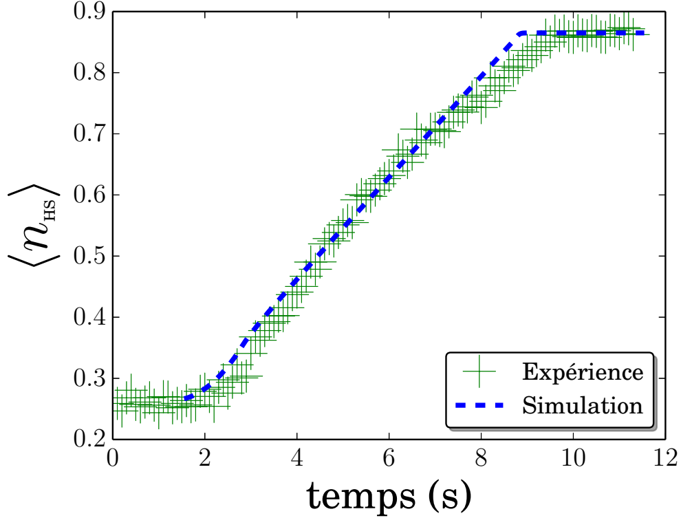
FIGURE 2.11 – Évolution temporelle de la fraction HS moyenne de la transformation LS vers HS d'un cristal [\{\text{Fe}(\text{NCSe})(\text{py})_2\}_2(m\text{-bpypz})] . Croix vertes et la ligne pointillée bleue représentent respectivement les données expérimentales et la simulation numérique de l'équation de réaction diffusion. Les valeurs des paramètres sont les mêmes que pour la figure 2.10, à T = 115.04\text{K} \simeq 1.02T_{eq} , pour D = 16.6\mu\text{m}^2\text{s}^{-1} et \Gamma \simeq 0.36\text{K}^{-1}\text{s}^{-1} .
