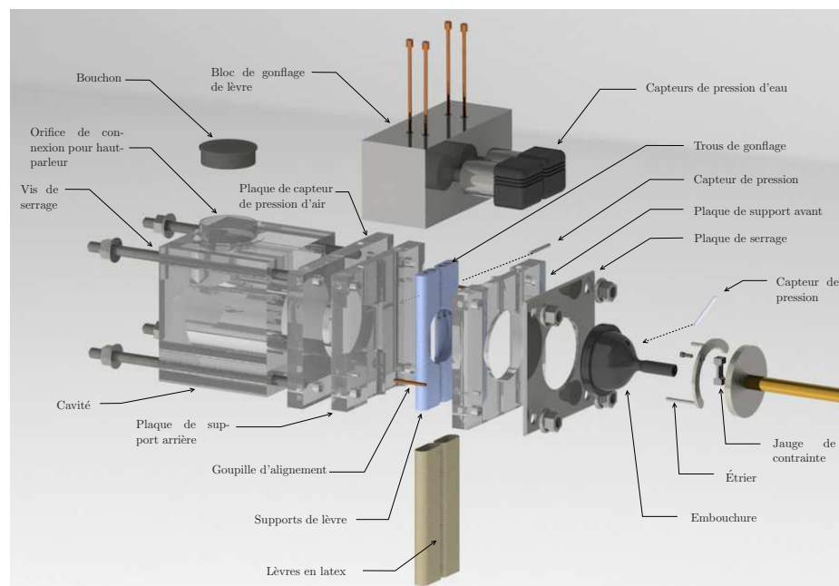
FIGURE 5.3 – Mod lisation 3D  clat e de la bouche artificielle et notation des  l ments : version   deux l vres vibrantes.
