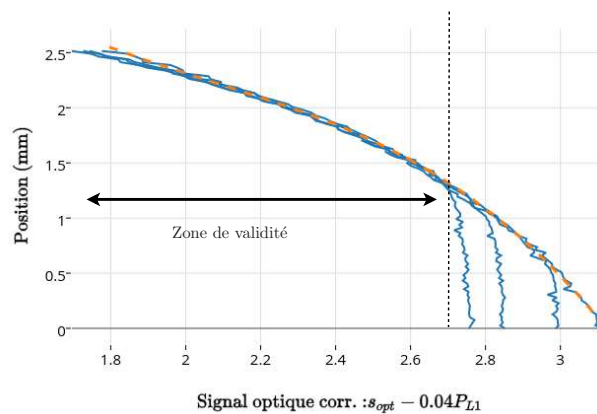
FIGURE 6.2 – (Haut) Résultat de l'expérience de balayage de plaque pour des pressions de lèvre de 20kPa, 15kPa, 10kPa et 5kPa; (Bas) Position en fonction du signal optique corrigé en pression et modèle estimé et zone de validité.
