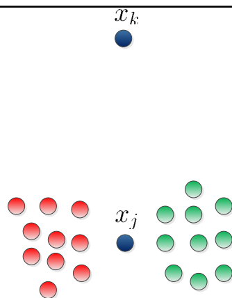
Figure 1. Le problème des partitions floues.
