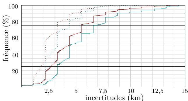
(e) Bulletin du RÉNASS : histogramme cumulé des incertitudes ( 1\sigma ) des événements en France métropolitaine (dont le Massif armoricain) et sur le Massif armoricain correspondant à l'incertitude maximum (trait plein) et minimum (trait pointillé) des longitude/latitudes ;
