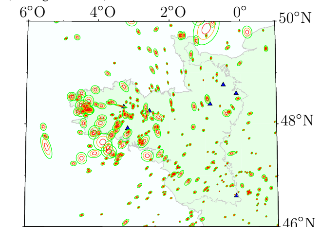
(d) Bulletin du LDG (détail de b) : 371 événements localisés avec, au plus, 7 stations sur le Massif armoricain ;
