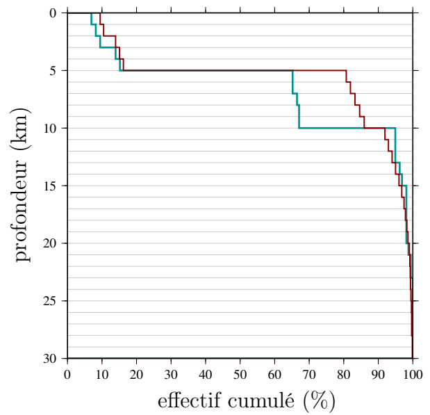
(b) Bulletin du RÉNASS entre 2011 et 2013.
