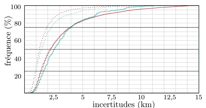
(f) Bulletin du LDG : histogramme cumulé des incertitudes ( 1\sigma ) des événements en France métropolitaine (dont le Massif armoricain) et sur le Massif armoricain correspondant à l'axe a (c.-à-d. le diamètre le plus grand de l'ellipse, trait plein) et l'axe b (trait pointillé) des ellipsoïde.
