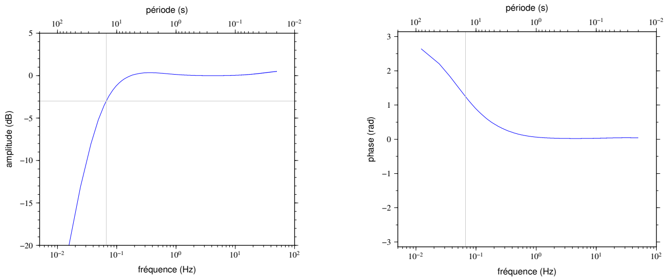
Figure VI-2 – Réponse instrumentale d'un capteur Titan-NoeMax (figure VI-1) ; le capteur a une fréquence propre de 4,5 Hz \pm 10\% et une fréquence de coupure d'environ 15 s pour -3 dB (JVALRESP, Instrumental Software Technologies, Inc.)
