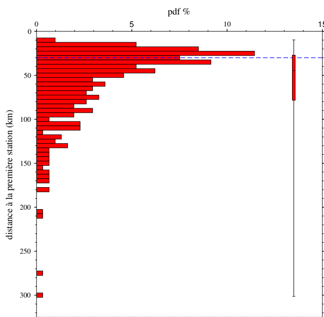
Figure IV.1-6 – Distribution des distances à la première station. La ligne bleue tiretée correspond à la distance maximale préconisée par Bondár & coll. (2004). La « boîte à moustache » représente la médiane, les quartiles et les valeurs extrêmes.
