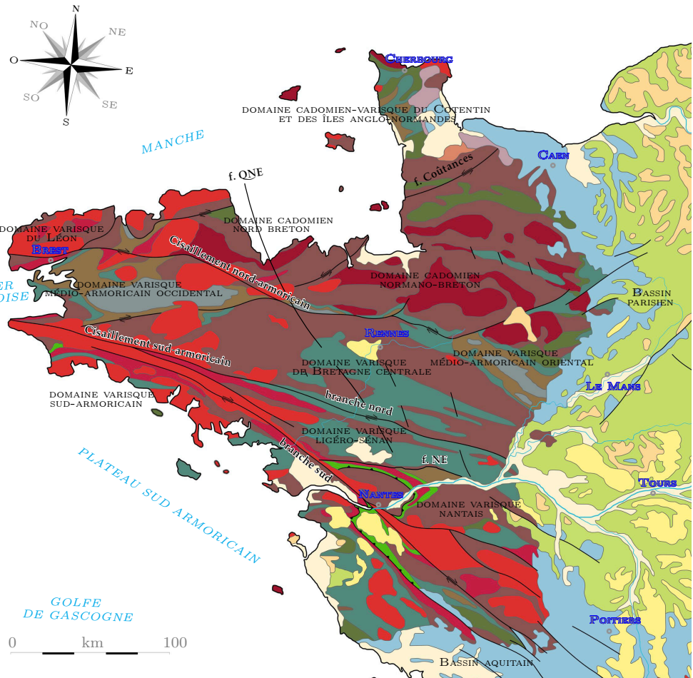
Figure I.2-3 – Carte géologique schématisée simplifiée du Massif armoricain (modifiée d'après, Chantraine & coll., 2003 ; Aertgeerts, 2016) : f. QNE : faille de Quessoy–Nort-sur-Erdre (composée de nombreuses failles de quelques dizaines de kilomètres, sa signature n'est pas continue en surface); f. NE : faille de Nort-sur-Erdre.
