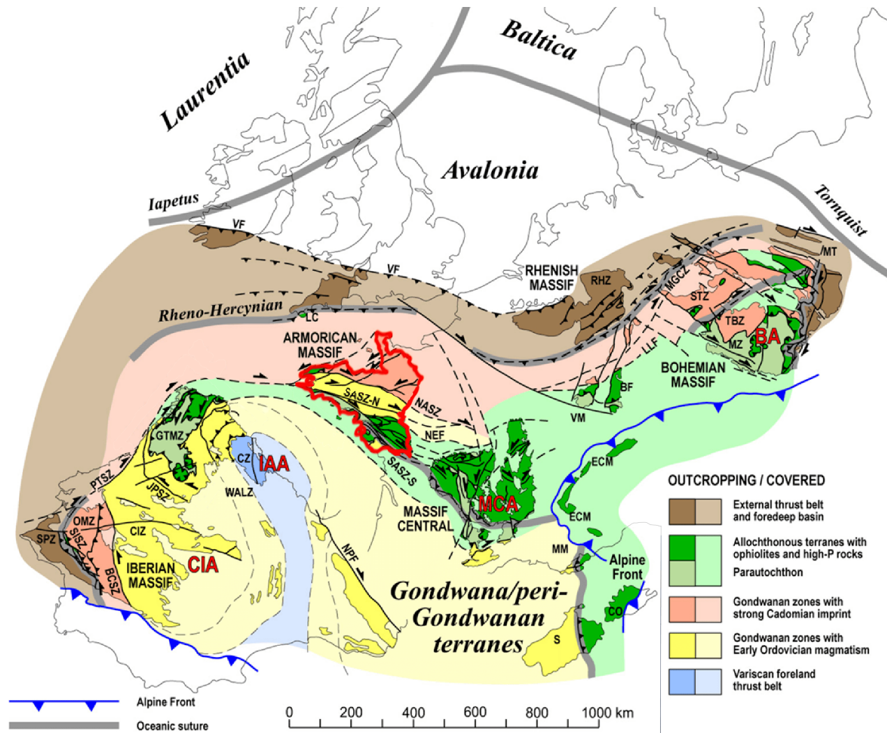
Figure I.2-1 – Schéma tectonique de la Ceinture varisque d'Europe de l'Ouest étendue sur près de 3000 km, depuis la péninsule Ibérique jusqu'à la Bohême (d'après Ballèvre & coll., 2014). Le Massif armoricain est entouré en rouge.
