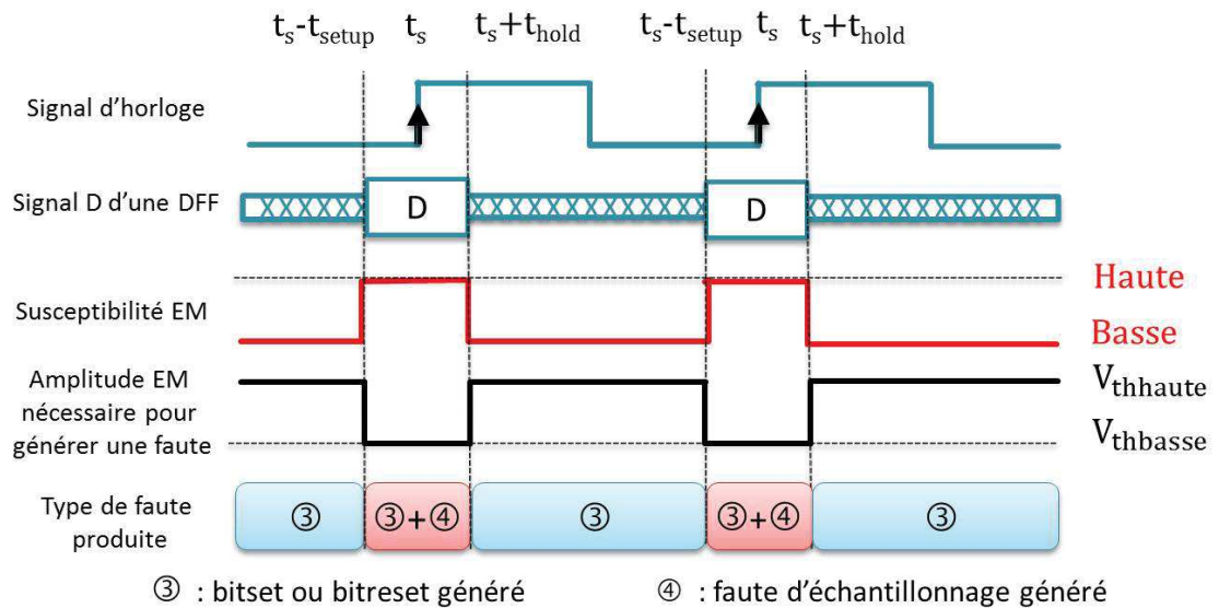
FIGURE 4.16: Modèle 'faute d'échantillonnage'
