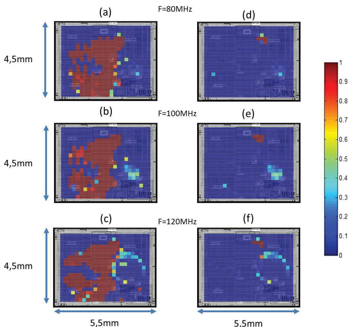
FIGURE 5.10: Cartographies de la probabilité, (a,b,c) d'induire un comportement erroné quelconque avec une impulsion EM et (d,e,f) une faute de chiffrement
