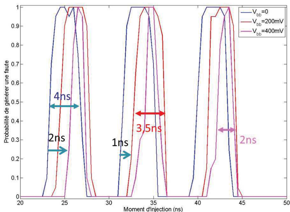
FIGURE 5.15: Probabilité de générer une faute sur un AES hardware implémenté sur un micro-contrôleur 32bit en fonction du moment d'injection ( t_{pulse} ) pour 3 valeurs de tension de polarisation du substrat et avec une sonde d'injection plate
