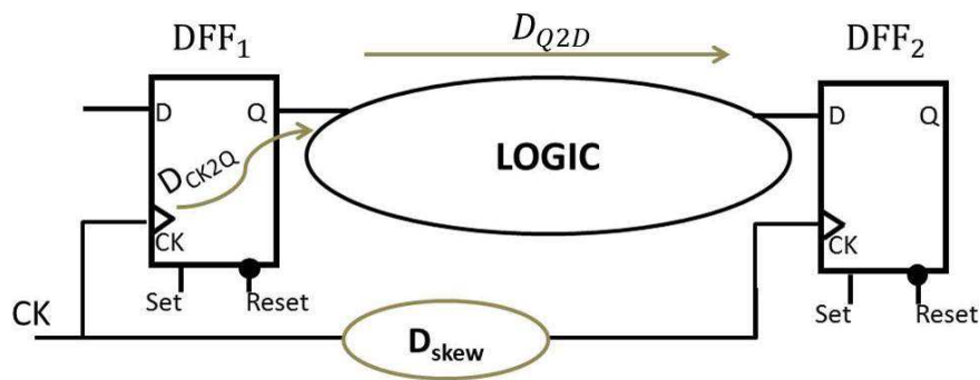
FIGURE 4.3: Schéma d'un circuit synchrone
