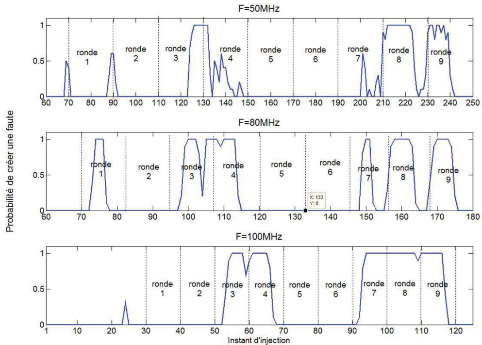
FIGURE 5.13: Probabilité de générer une faute sur un AES hardware implémenté sur un micro-contrôleur 32bit en fonction du moment d'injection ( t_{pulse} ) pour 3 valeurs de fréquence de fonctionnement et avec une sonde d'injection plate
