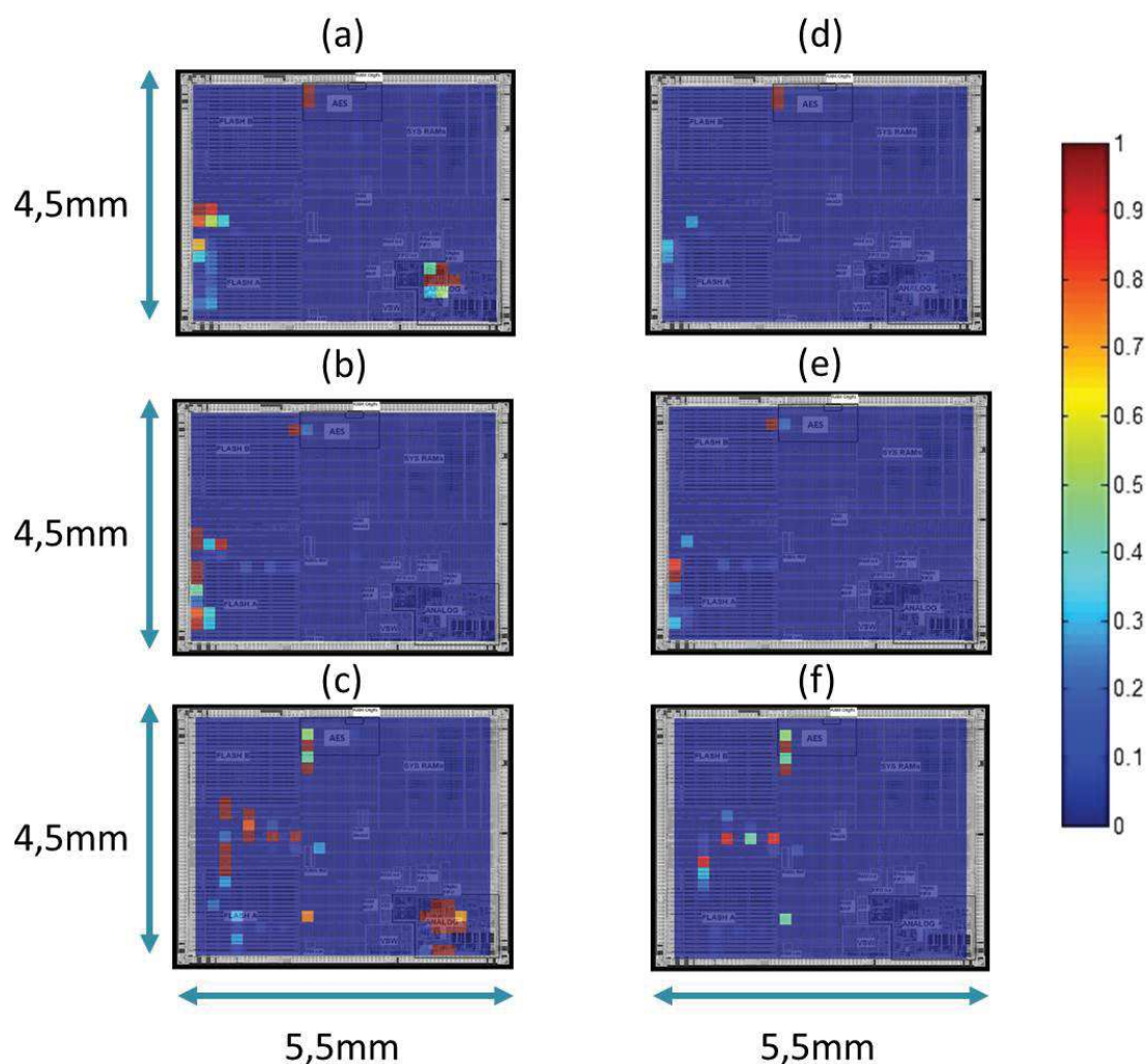
FIGURE 5.16: Zones de susceptibilité du micro-contrôleur pour n'importe quel type d'erreur avec des tension de polarisation du substrat de (a) 0mV, (b) 200mV et (c) 400mV. Zones de susceptibilité du micro-contrôleur pour une erreur sur le texte chiffré avec des tension d'alimentation de (d) 0mV, (e) 200mV et (f) 400mV
