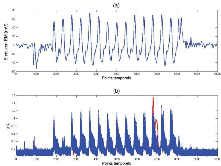
FIGURE 2.9: (a) Trace EM d'un chiffrement AES, (b) Evaluation de \Delta K_s pour une valeur de sous-clé dans le temps
