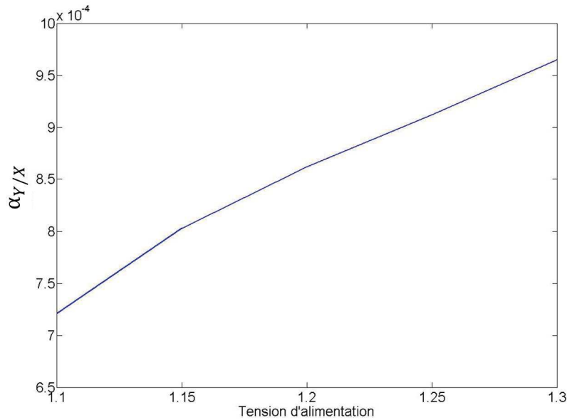
FIGURE 3.5: Coefficient \alpha_{Y/X} en fonction de la valeur de V_{dd}
