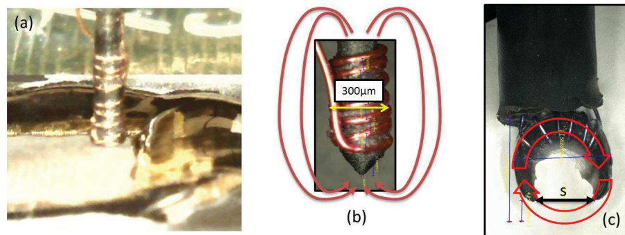
FIGURE 4.2: (a) Sondes d'injection plate, (b) Sonde d'injection appointée, (c) Sonde d'injection oméga
