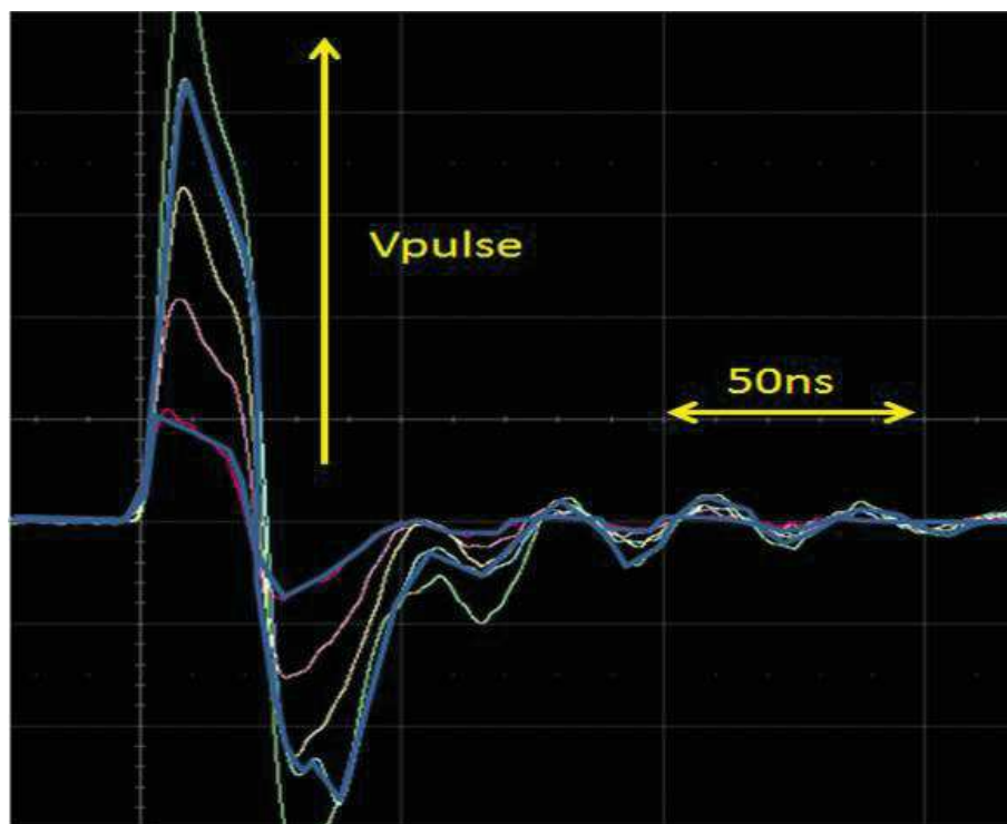
FIGURE 4.14: Image d'un champ EM émis par une sonde d'injection lors d'une injection EMP
