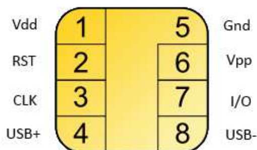
FIGURE 2.4: Connecteur d'une carte à puce défini dans la norme ISO.7816
