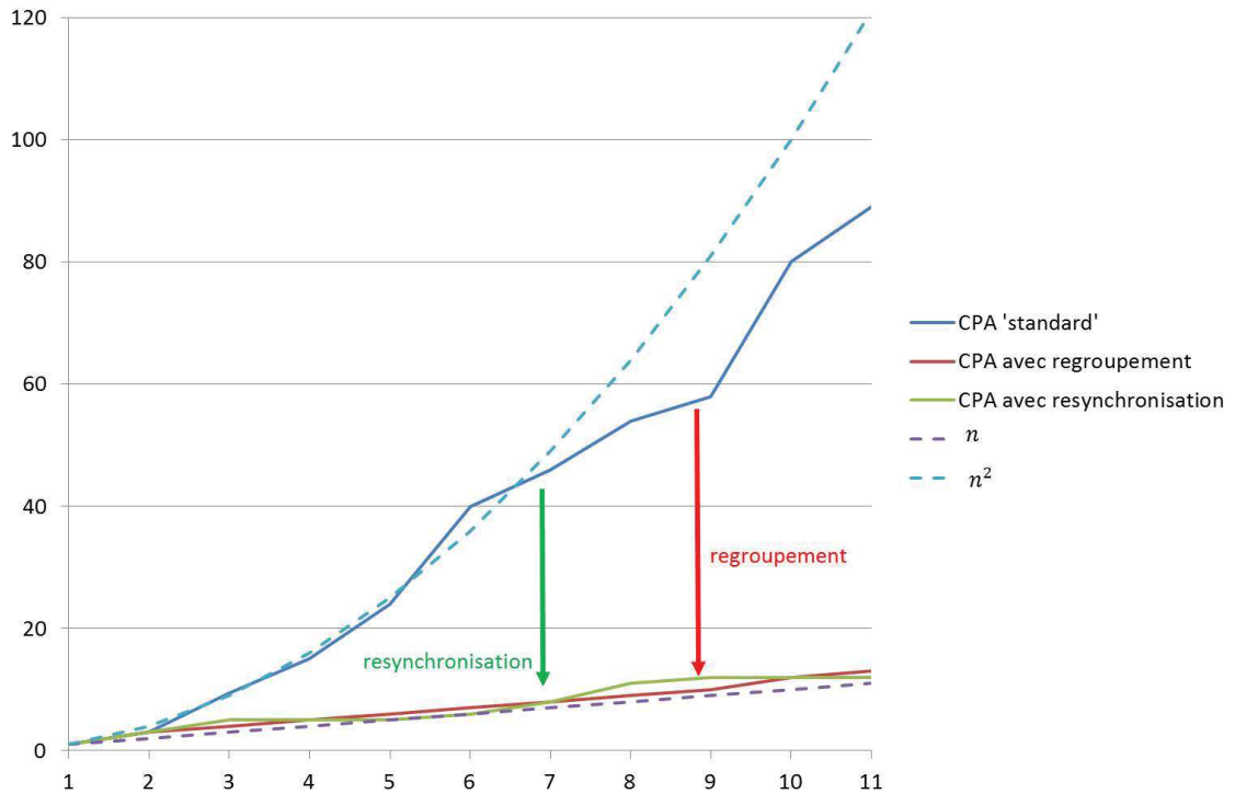
FIGURE 3.14: Evolutions du rapport de robustesse \frac{S_n}{S_1} en fonction du nombre n de couples utilisés avec une CPA 'standard', une CPA avec resynchronisation et une CPA avec regroupement
