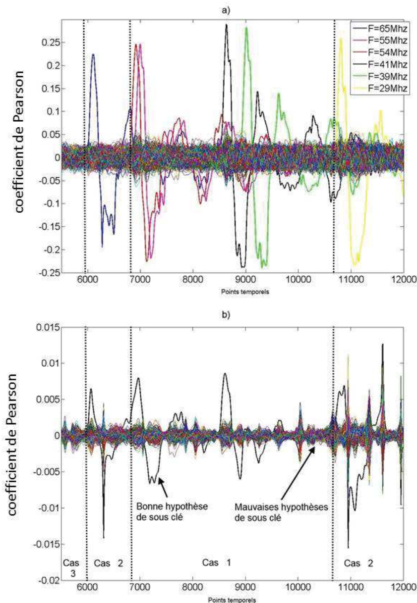
FIGURE 3.9: (a)Évolution de la corrélation associée à chaque hypothèse de sous clé pour les six couples (V, F) pris séparément, (b) évolution de la corrélation associée à chaque hypothèse de sous clé lorsque la RDVFS est activée avec les six couples (V, F)
