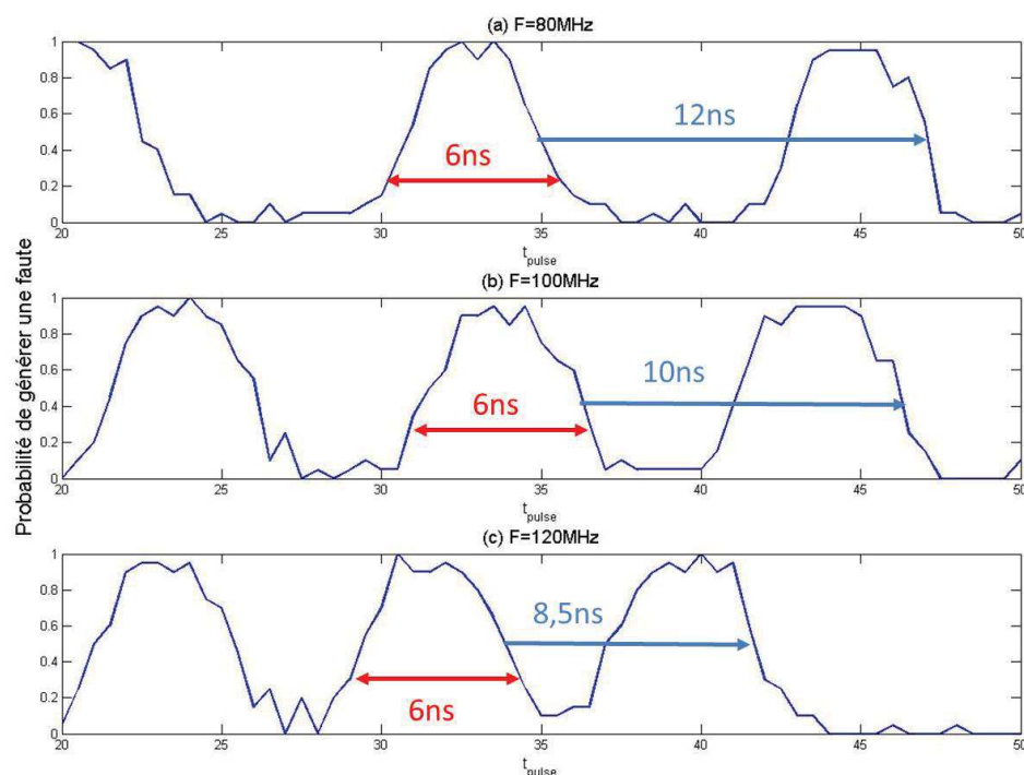
FIGURE 5.11: Probabilité de générer une faute sur un AES matériel implémenté sur un micro-contrôleur 32bit en fonction du moment d'injection ( t_{pulse} ) pour 3 valeurs de fréquence de fonctionnement
