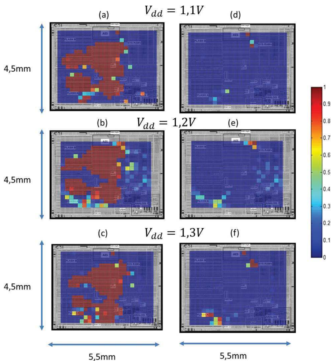
FIGURE 5.6: Cartographie de la probabilité d'induire (a,b,c) n'importe quel type de fautes avec une injection EMP lorsque le circuit est alimenté sous 1.1V(a), 1.2V(b) et 1.3V(c), (d,e,f) des fautes de chiffrement dans l'AES matériel alimenté sous 1.1V(d), 1.2V(e) et 1.3V(f)
