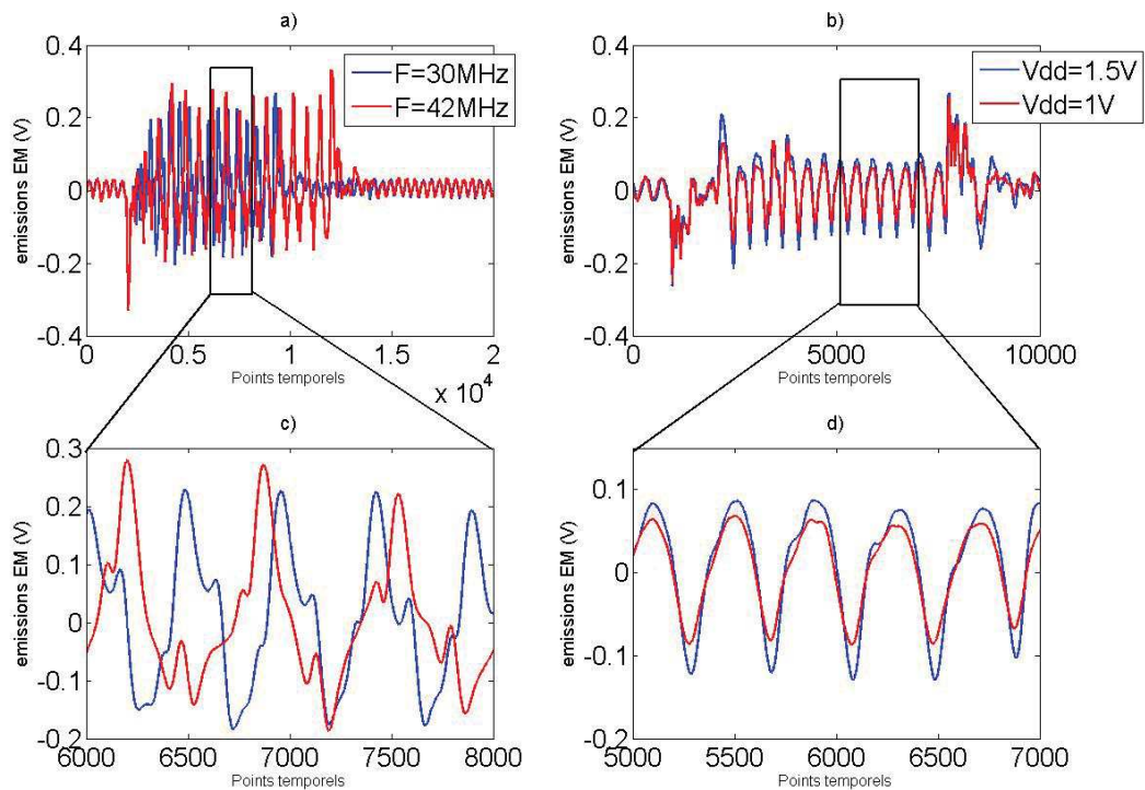
FIGURE 3.2: (a) et (c) rayonnement EM relatif à un chiffrement AES pour F = 30\text{MHz} et F = 42\text{MHz} , (b) et (d) rayonnement EM relatif à un chiffrement AES pour V_{dd} = 1\text{V} et V_{dd} = 1.5\text{V}
