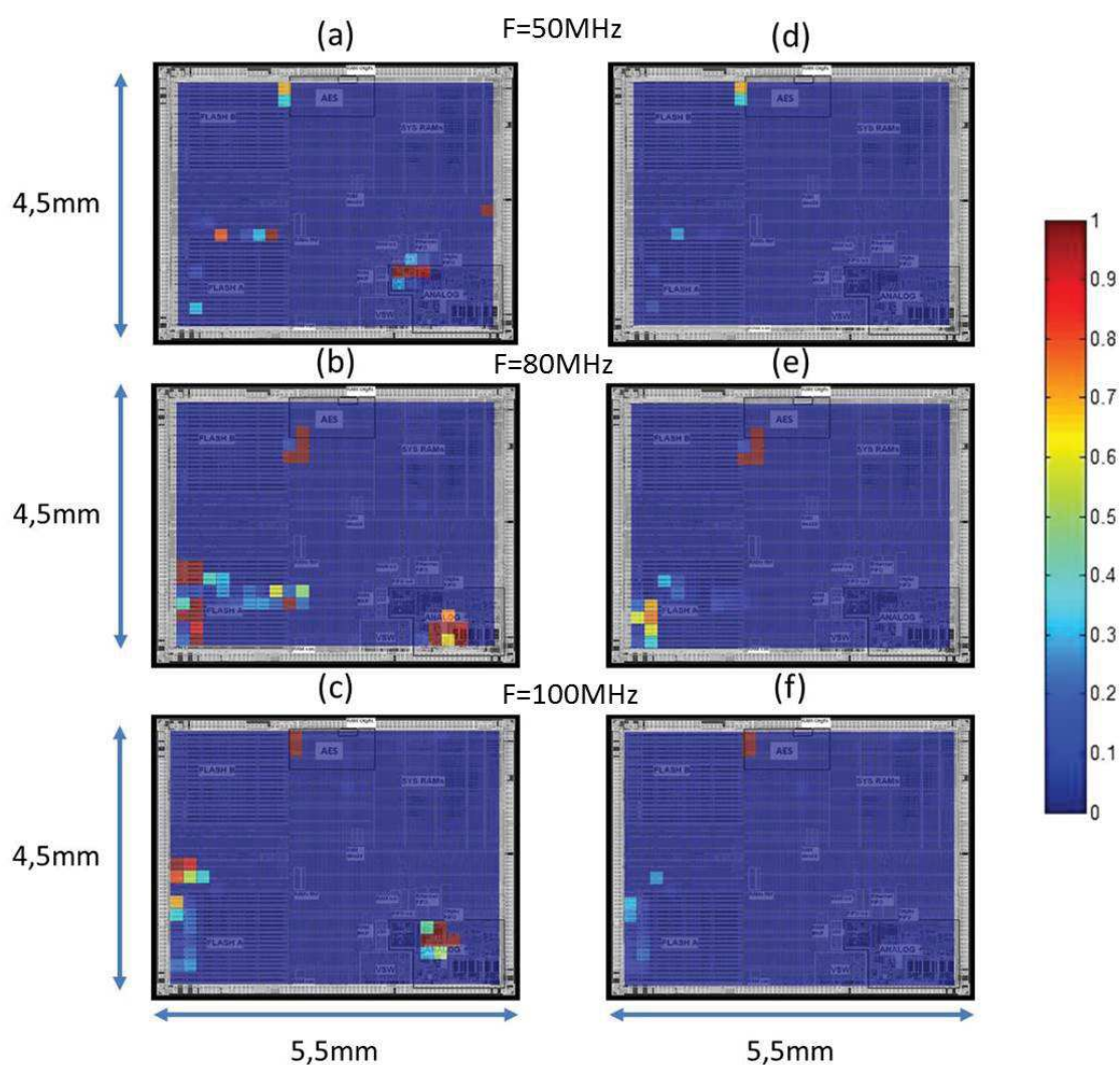
FIGURE 5.12: Cartographies de la probabilité (a,b,c) d'induire n'importe quel comportement erroné avec l'injection BBI lorsque le circuit fonctionne à 50MHz(a), 80MHz(b) et 100MHz(c); (d,e,f) d'induire des fautes de chiffrement avec l'injection BBI lorsque le circuit fonctionne à 50MHz(d), 80MHz(e) et 100MHz(f)
