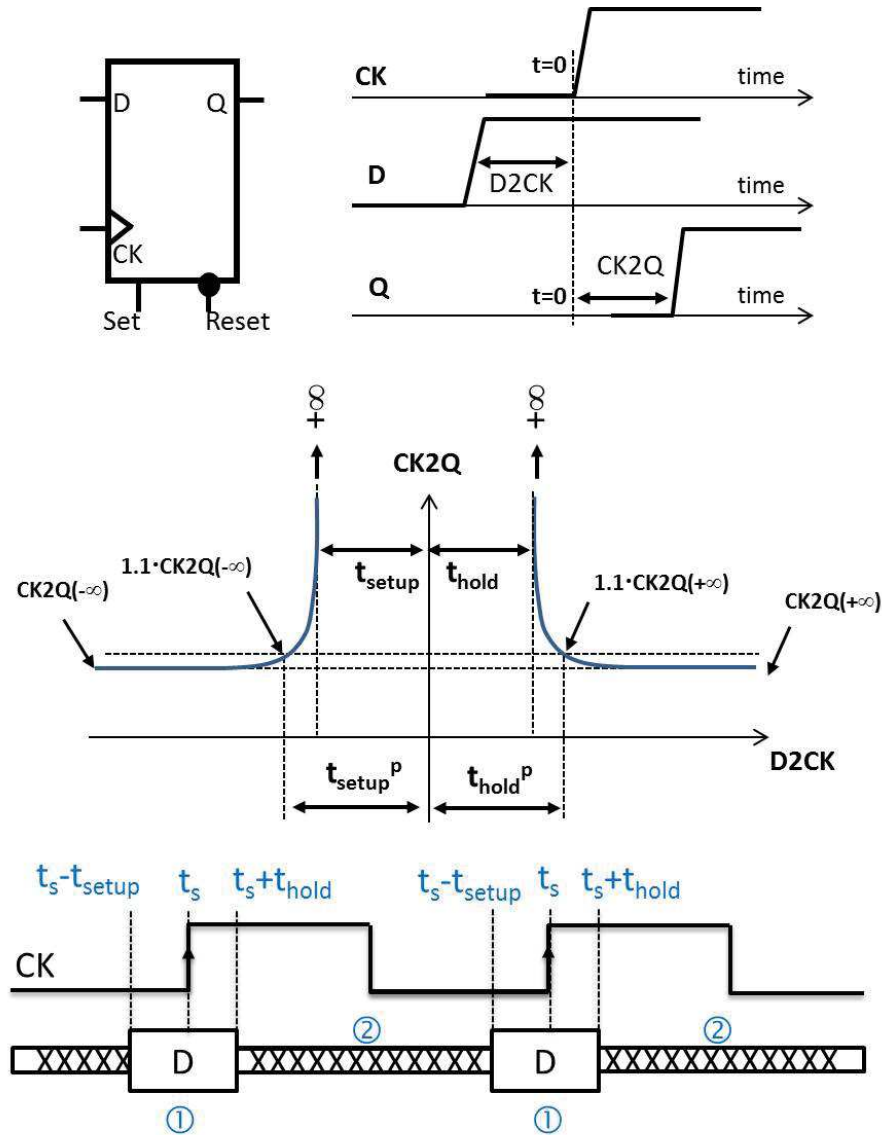
FIGURE 4.4: Symbole d'une DFF et définition du temps de setup ( t_{setup} ) et du temps de hold ( t_{hold} )
