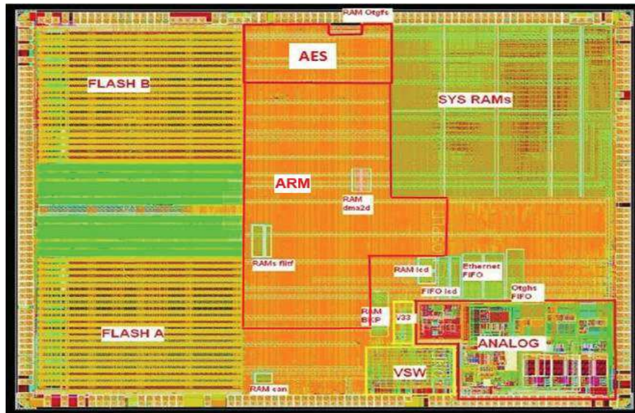
FIGURE 5.1: Placement des différents blocs du micro-contrôleur
