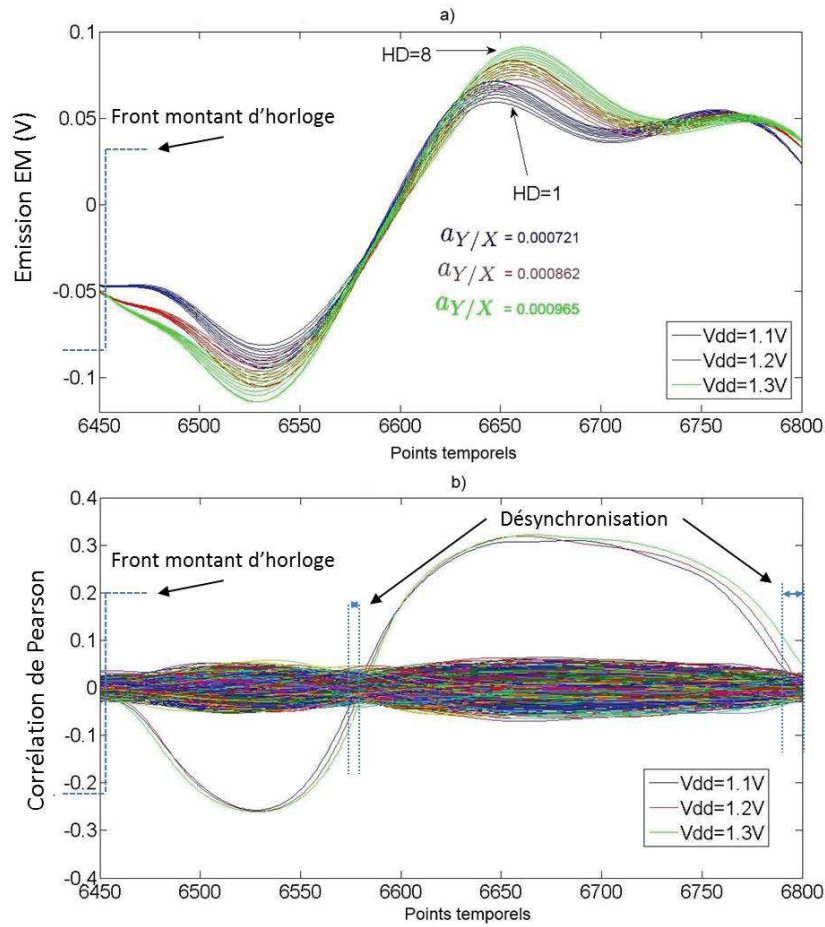
FIGURE 3.4: (a) Traces EM d'un AES pendant la fuite d'information pour trois valeurs de V_{dd} différentes, (b) valeurs de corrélation considérées par la CPA pour trois valeurs de V_{dd} différentes
