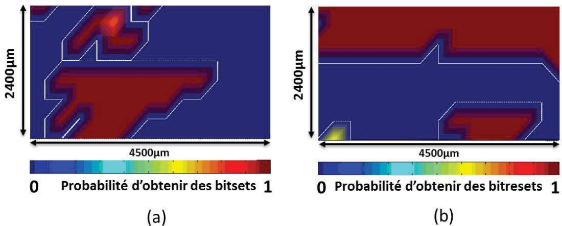
FIGURE 4.7: Probabilité de produire (a) une faute de type bitset avec un V_{pulse}=+140V et (b) une faute de type bitreset avec un V_{pulse}=-140V
