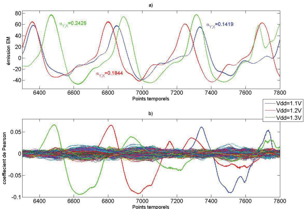
FIGURE 3.6: (a) Traces EM d'un AES pendant la fuite d'information pour trois valeurs différentes de V_{dd} , (b) valeurs de corrélation considérées par la CPA pour trois valeurs de V_{dd}
