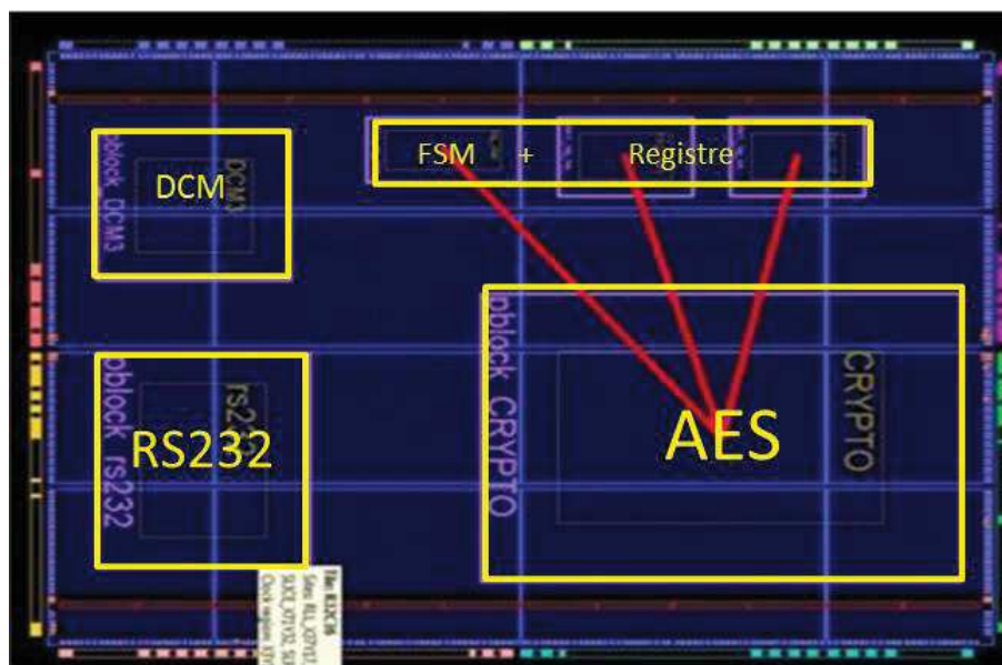
FIGURE 4.8: Placement des différents blocs du circuit de test
