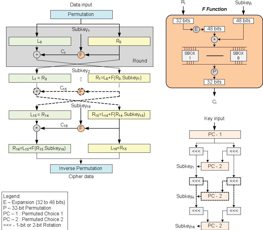
FIGURE 2.1: Structure du DES
