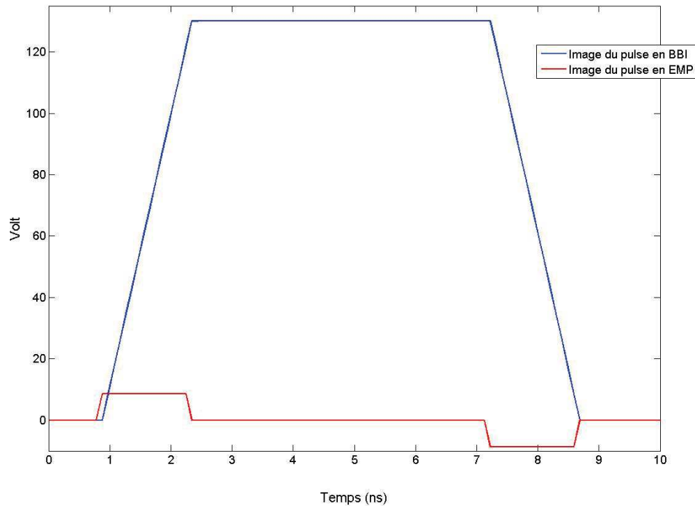
FIGURE 5.5: Image de l'impulsion perturbant le circuit pour l'injection EMP et BBI
