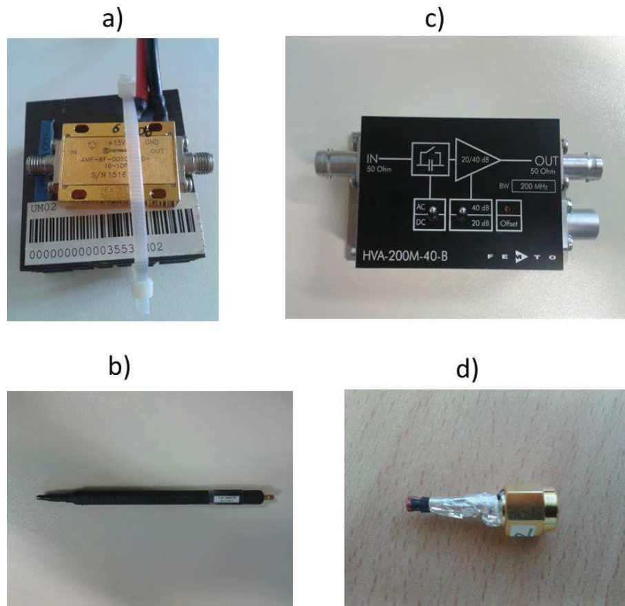
FIGURE A.2: Ancien et nouveau matériels du LIRMM. a) Amplificateur [100MHz,1GHz], b) sonde d'acquisition [30MHz,1GHz], c) amplificateur [10KHz,200MHz] et d) sonde d'analyse avec un cœur de ferrite
