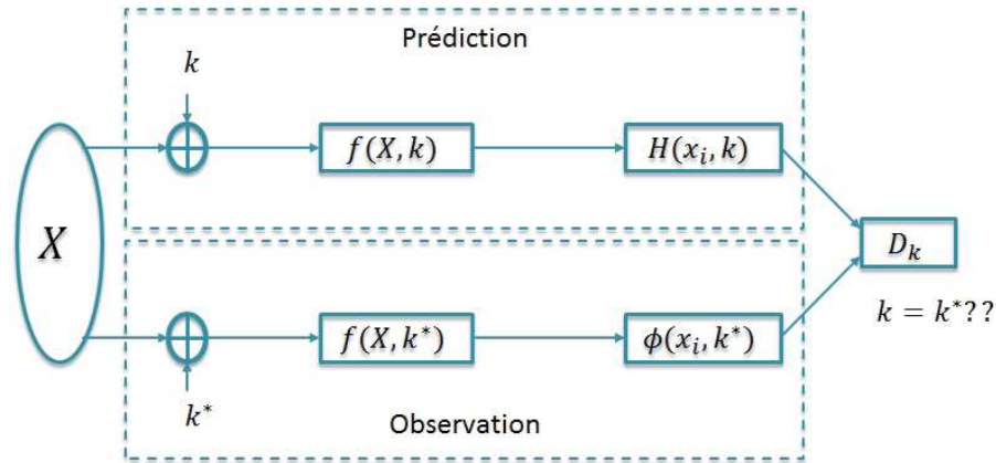
FIGURE 2.8: Principe d'une attaque verticale
