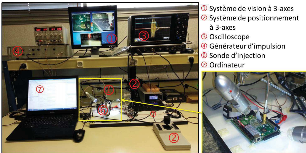
FIGURE 4.1: Plateforme d'injection EMP du LIRMM
