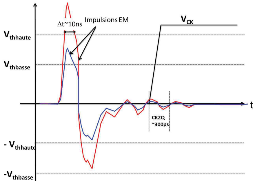
FIGURE 4.15: Image d'un champ EM émis par une sonde d'injection lors d'une injection EMP
