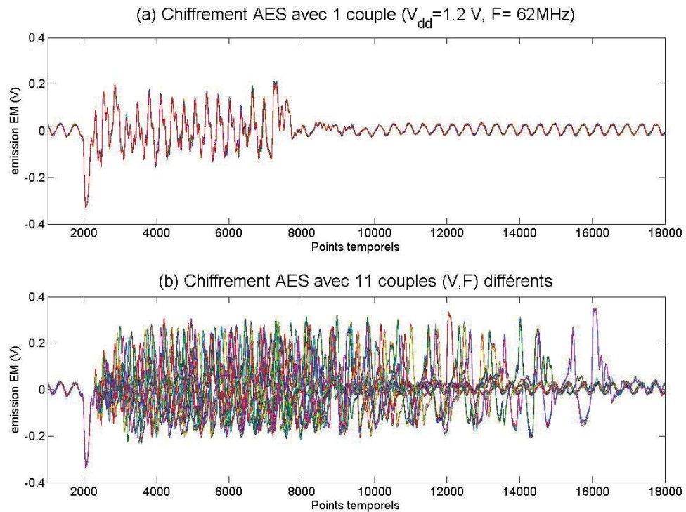
FIGURE 3.3: (a) Chiffrement AES avec (V, F) = (1.2\text{ V}, 62\text{ MHz}) fixe, (b) Chiffrement AES avec 11 couples (V, F) différents
