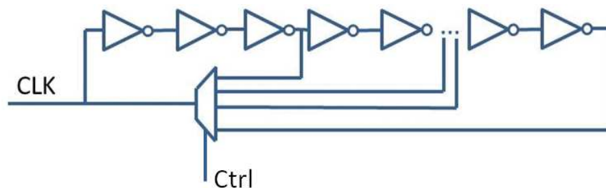
FIGURE 3.10: Oscillateur en anneau fournissant le signal d'horloge à l'AES.
