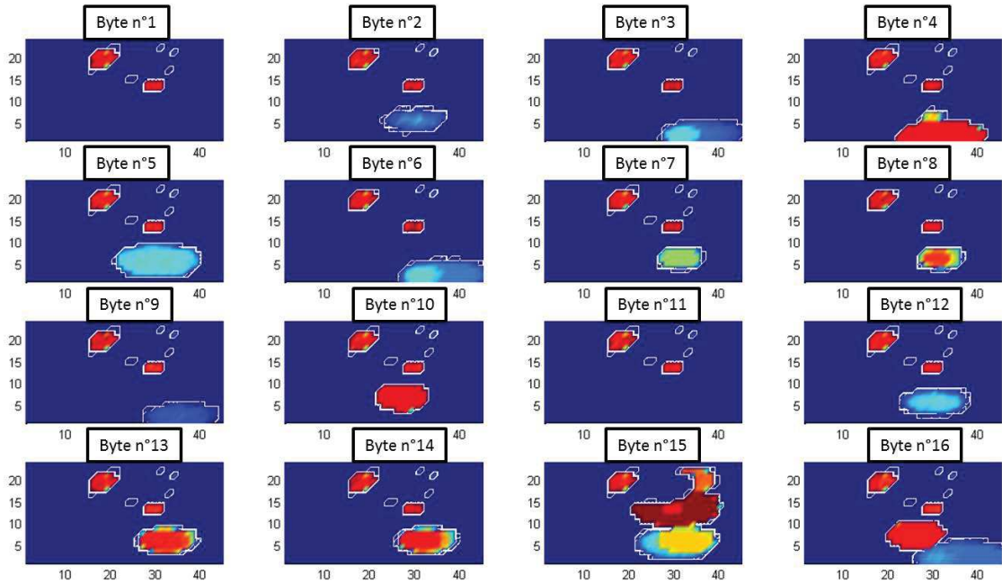
FIGURE 4.10: Probabilité de générer une faute pour chaque octet de l'AES en fonction de la position de la sonde d'injection ( \omega )
