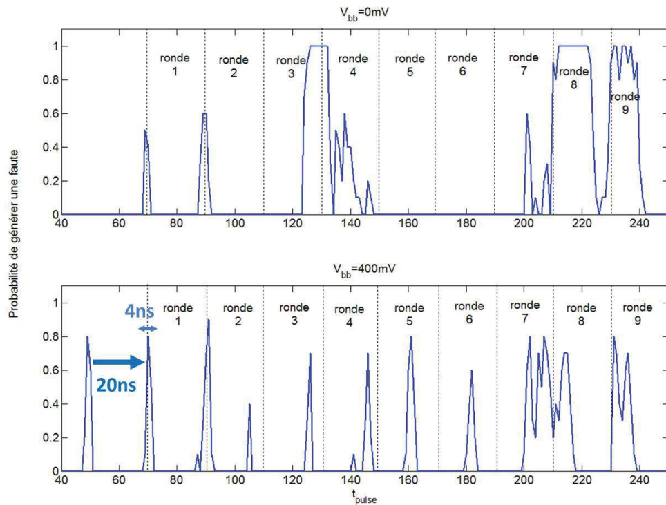
FIGURE 5.17: Probabilité de générer une faute sur un AES hardware implémenté sur un micro-contrôleur 32bit en fonction du moment d'injection ( t_{pulse} ) pour 2 valeurs de tension de polarisation du substrat
