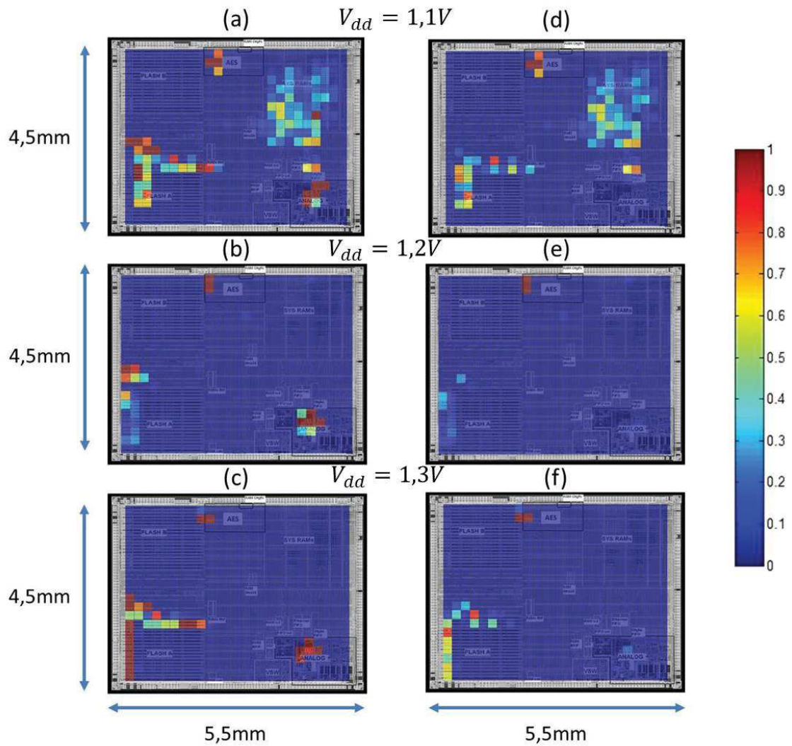
FIGURE 5.8: Cartographies (a,b,c) de la probabilité d'induire un comportement erroné quelconque lorsque le circuit est alimenté à 1.1V(a), 1.2V(b) et 1.3V(c). Cartographies (d,e,f) de la probabilité de générer un chiffre fauté lorsque le circuit est alimenté à 1.1V(d), 1.2V(e) et 1.3V(f)
