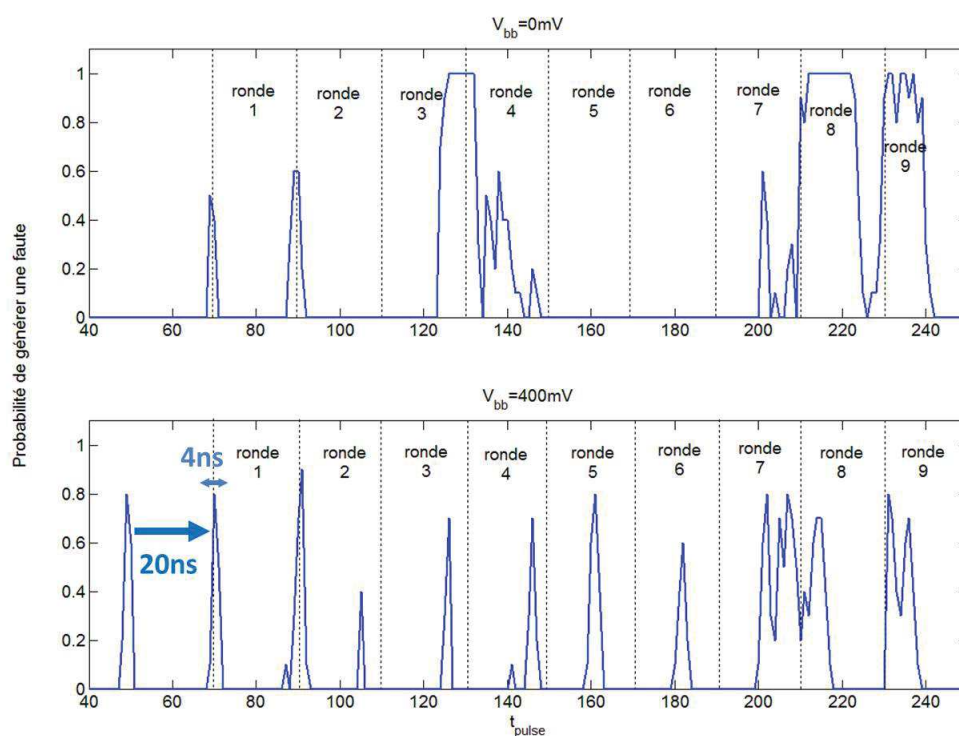
FIGURE 5.17: Probabilité de générer une faute sur un AES hardware implémenté sur un micro-contrôleur 32bit en fonction du moment d'injection ( t_{pulse} ) pour 2 valeurs de tension de polarisation du substrat
