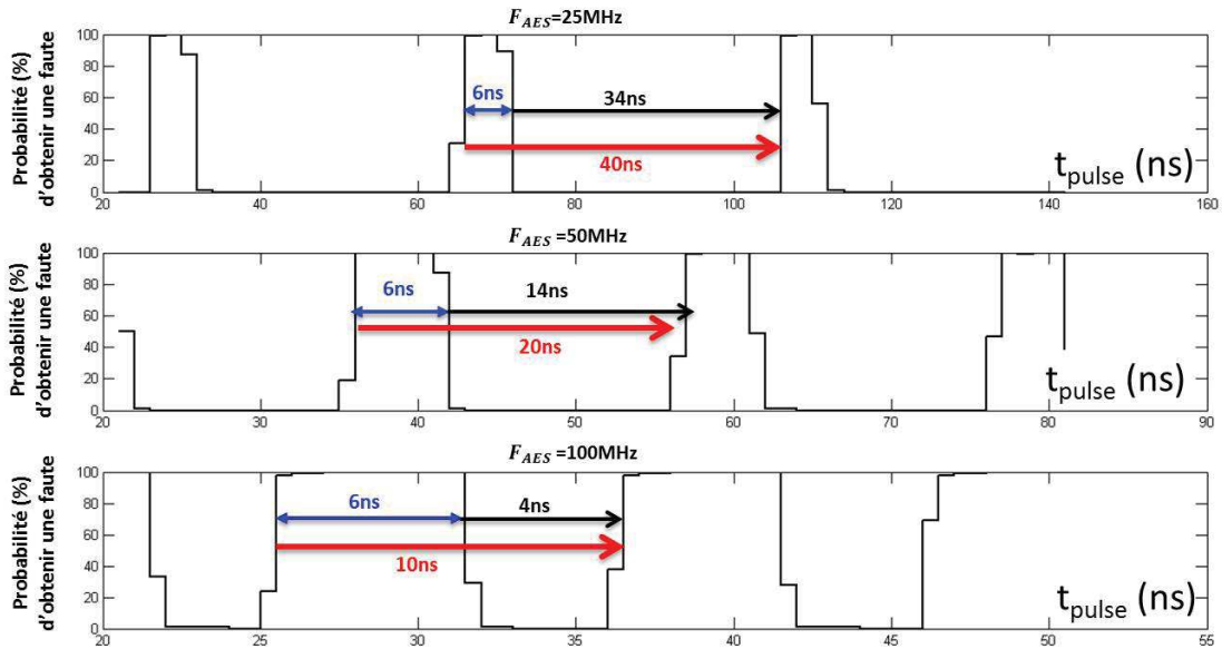
FIGURE 4.12: Probabilité de générer une faute sur un AES hardware implémenté sur un FPGA spartan3-1000 en fonction du moment de d'injection ( t_{pulse} ) pour 3 valeurs de fréquences différentes et avec une sonde d'injection oméga
