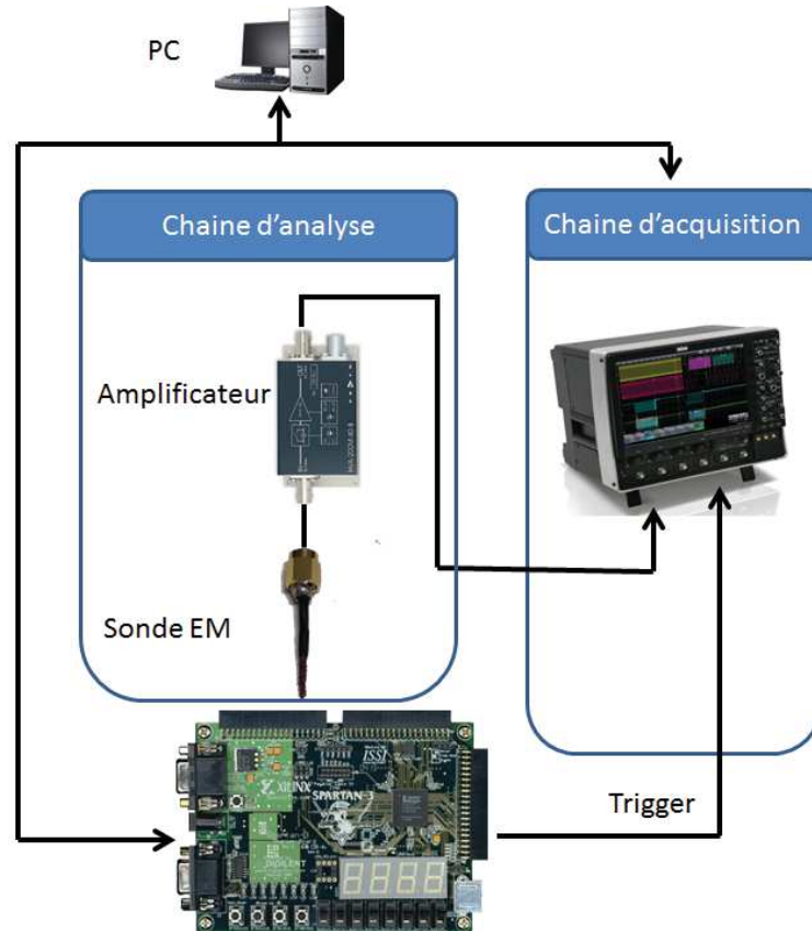
FIGURE 2.5: Banc d'acquisition de traces EM
