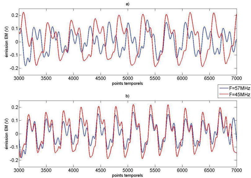
FIGURE 3.13: a) traces EM d'un chiffrement AES a deux fréquences différentes, b) traces EM d'un chiffrement AES resynchronisées
