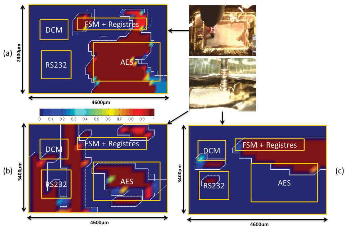
FIGURE 4.9: Probabilité de générer (a) un texte chiffré fauté avec la sonde d'injection oméga, (b) un texte chiffré fauté avec la sonde d'injection plate et (c) que le circuit soit muet avec la sonde d'injection plate
