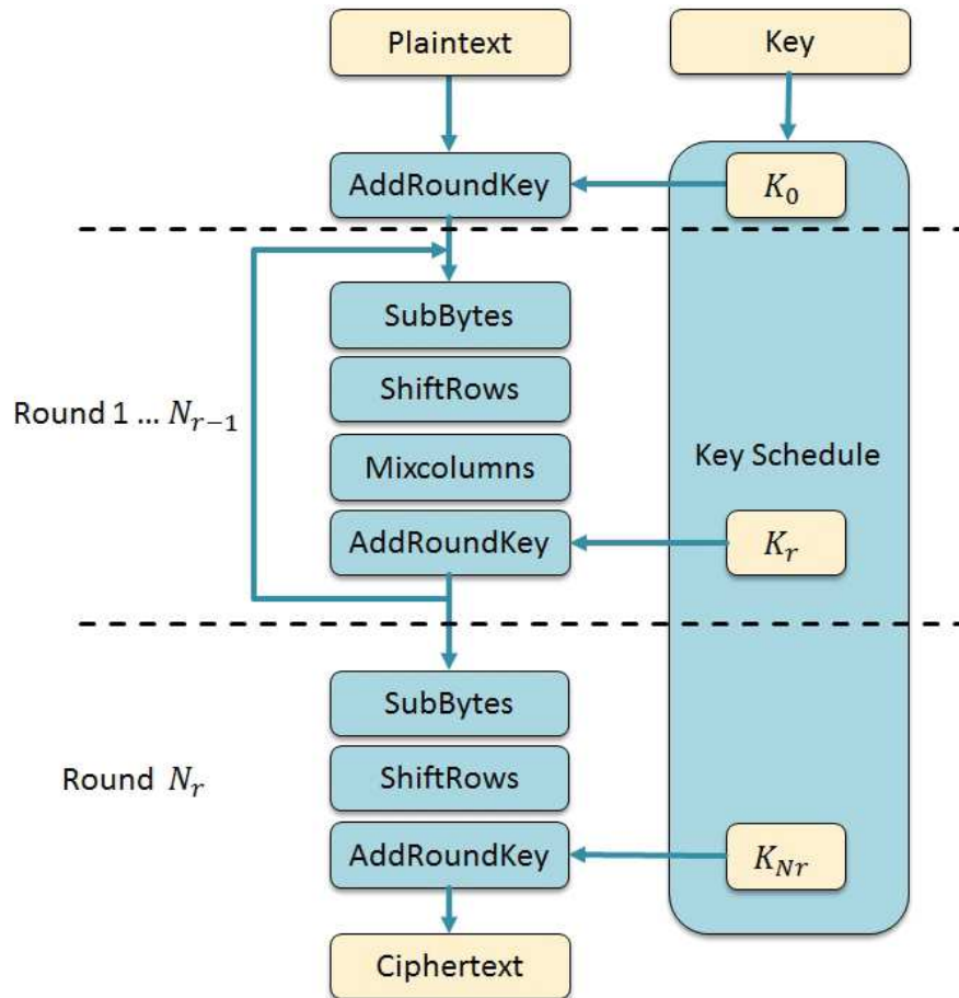
FIGURE 2.2: Structure de l'AES
