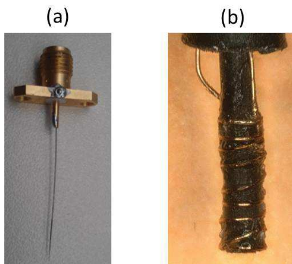
FIGURE 5.2: Sondes d'injection utilisées (a) sonde BBI et (b) sonde EMP
