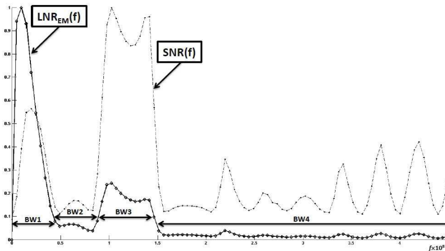
FIGURE A.1: Evolution du LNR_{EM}(f) et du SNR(f)
