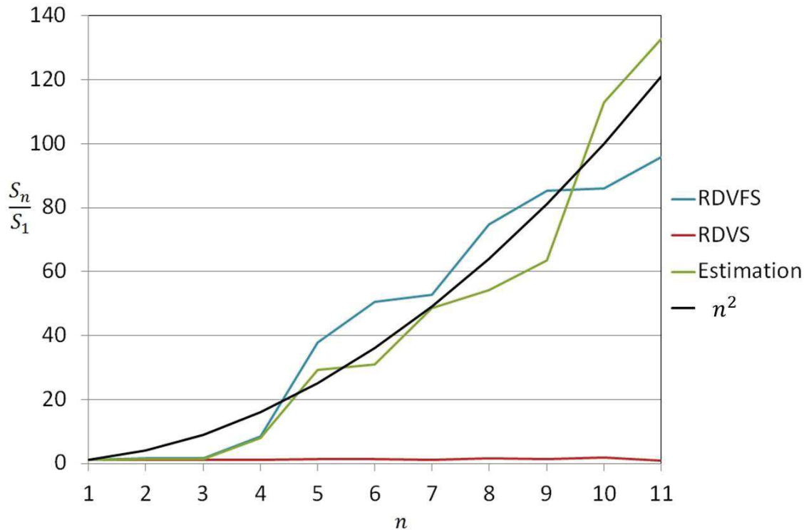
FIGURE 3.11: évolution du rapport de robustesse \frac{S_n}{S_1} en fonction du nombre n de couples (V,F) utilisés sur FPGA
