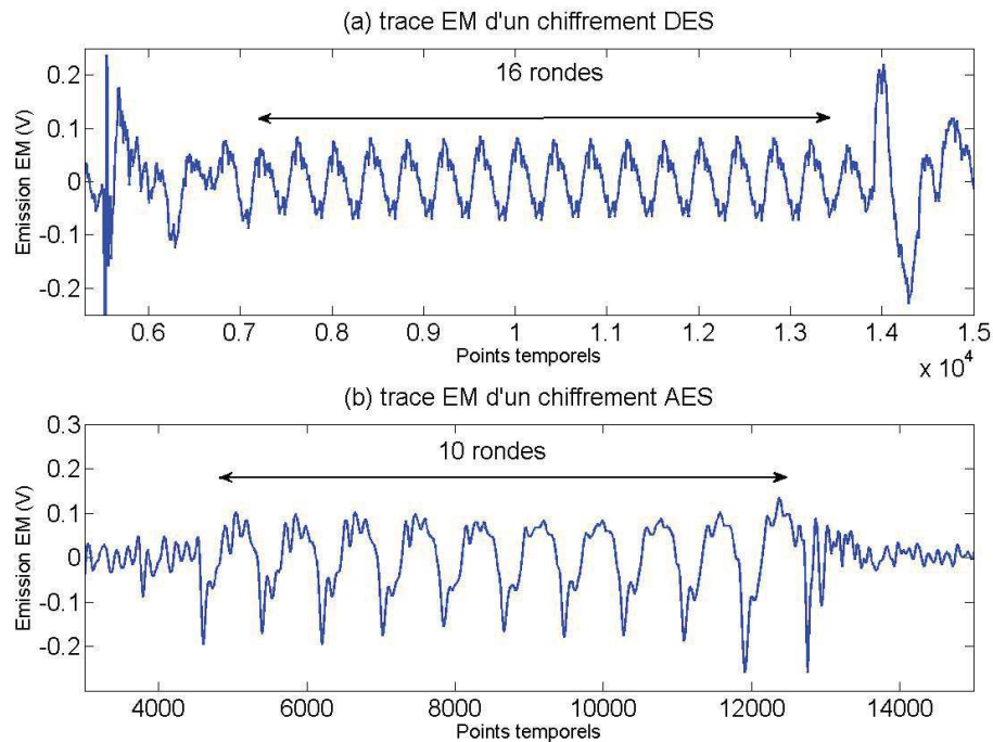
FIGURE 2.6: Traces EM collectées au dessus d'un circuit effectuant (a) un chiffrement DES et (b) un chiffrement AES
