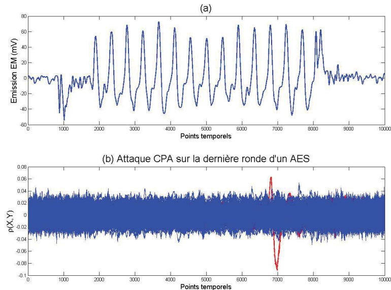
FIGURE 2.10: (a) Trace EM d'un AES, (b) Attaque CPA réalisée sur un AES
