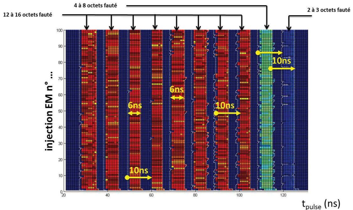
FIGURE 4.11: Nombre d'octets fautés à une position (X,Y) fixe en fonction du moment d'injection ( t_{pulse} ) pour 100 injections avec F_{AES} = 100MHz et une sonde d'injection oméga
