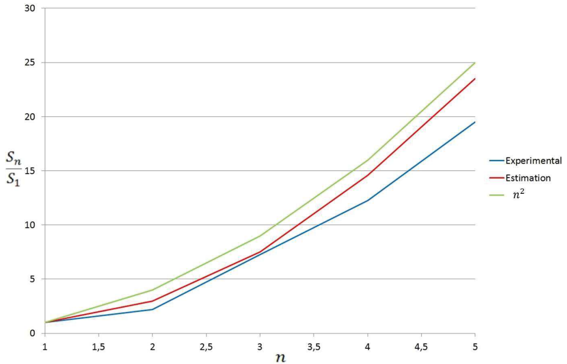
FIGURE 3.12: évolution du rapport de robustesse \frac{S_n}{S_1} en fonction du nombre de triplets n utilisés sur un micro-contrôleur 32 bits
