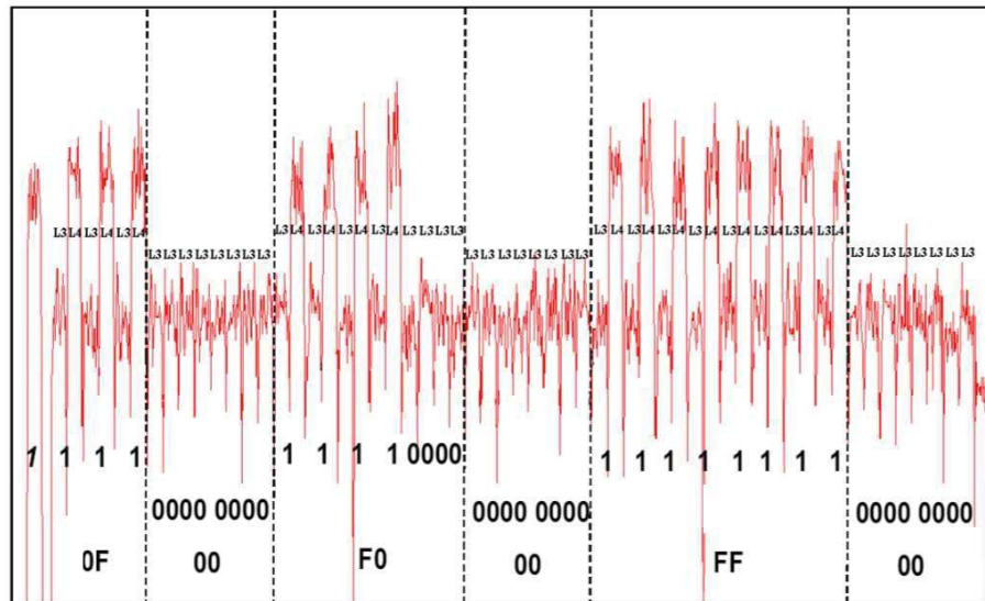
FIGURE 2.7: SPA sur la consommation d'un RSA non protégé
