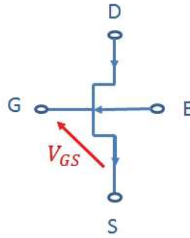
FIGURE 3.1: Transistor MOSfet à canal N
