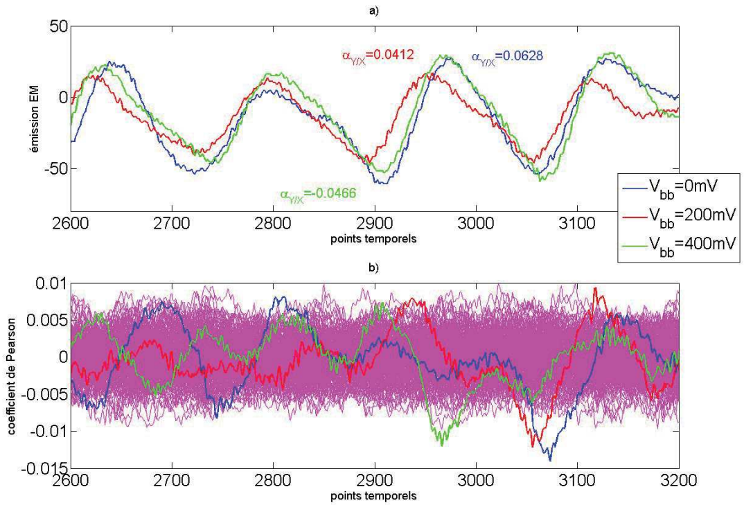
FIGURE 3.8: (a) Traces EM d'un AES pendant la fuite d'information pour trois valeurs différentes de V_{bb} , (b) corrélations considérées par la CPA pour trois valeurs différentes de V_{bb}
