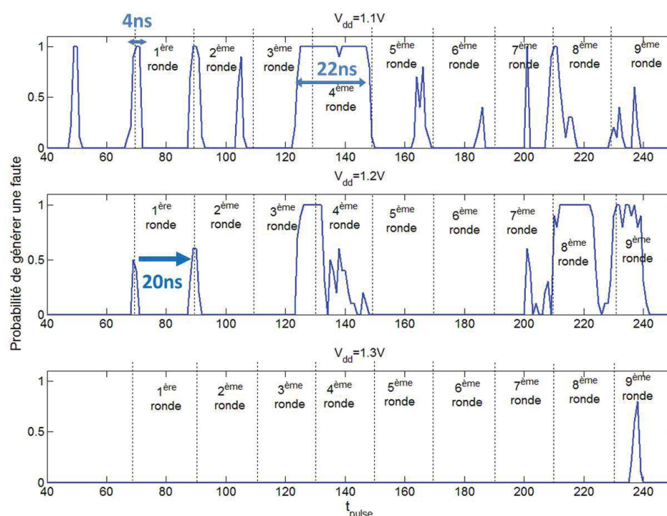
FIGURE 5.9: Evolution avec t_{pulse} de la probabilité d'induire une faute de chiffrement dans l'AES matériel du microcontrôleur et ce pour trois valeurs de tension d'alimentation
