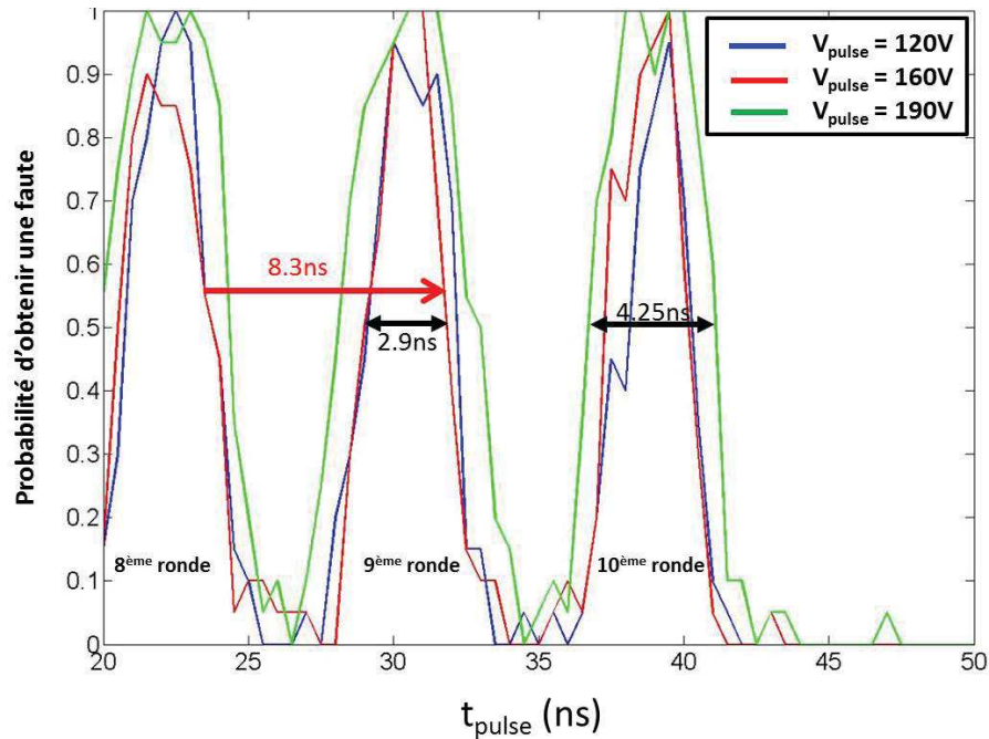
FIGURE 4.13: Probabilité de générer une faute sur un AES matériel implémenté sur un micro-contrôleur 32bit en fonction du moment d'injection ( t_{pulse} ) pour 3 valeurs de V_{pulse} et avec une sonde d'injection oméga
