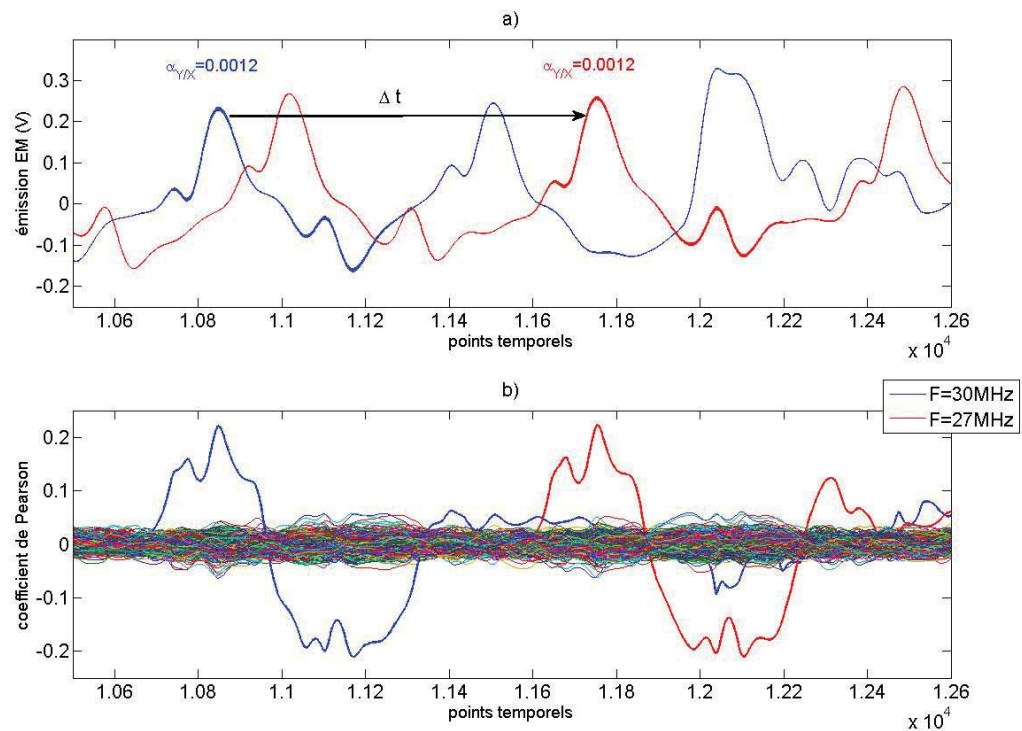
FIGURE 3.7: (a) Traces EM d'un AES pendant la fuite d'information avec deux valeurs différentes de F , (b) valeur de corrélation pour des attaques CPA avec deux valeurs différentes de F
