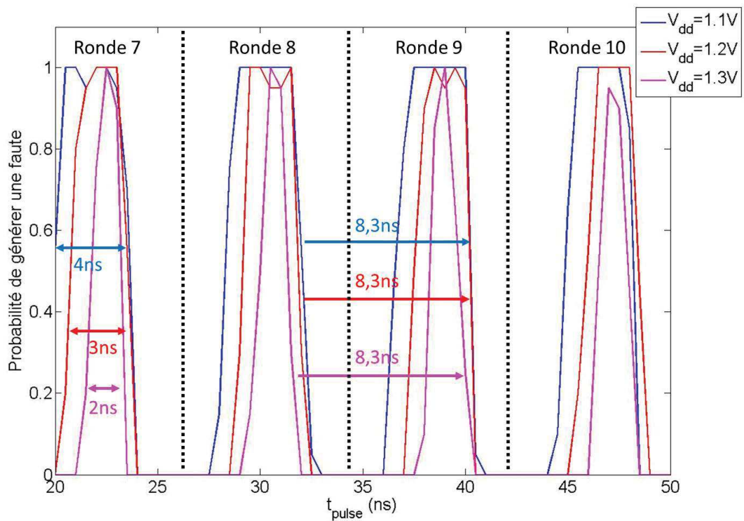
FIGURE 5.7: Probabilité de générer une faute sur un AES hardware implémenté sur un micro-contrôleur 32bit en fonction du moment d'injection ( t_{pulse} ) pour 3 valeurs de tension d'alimentation et avec une sonde d'injection plate
