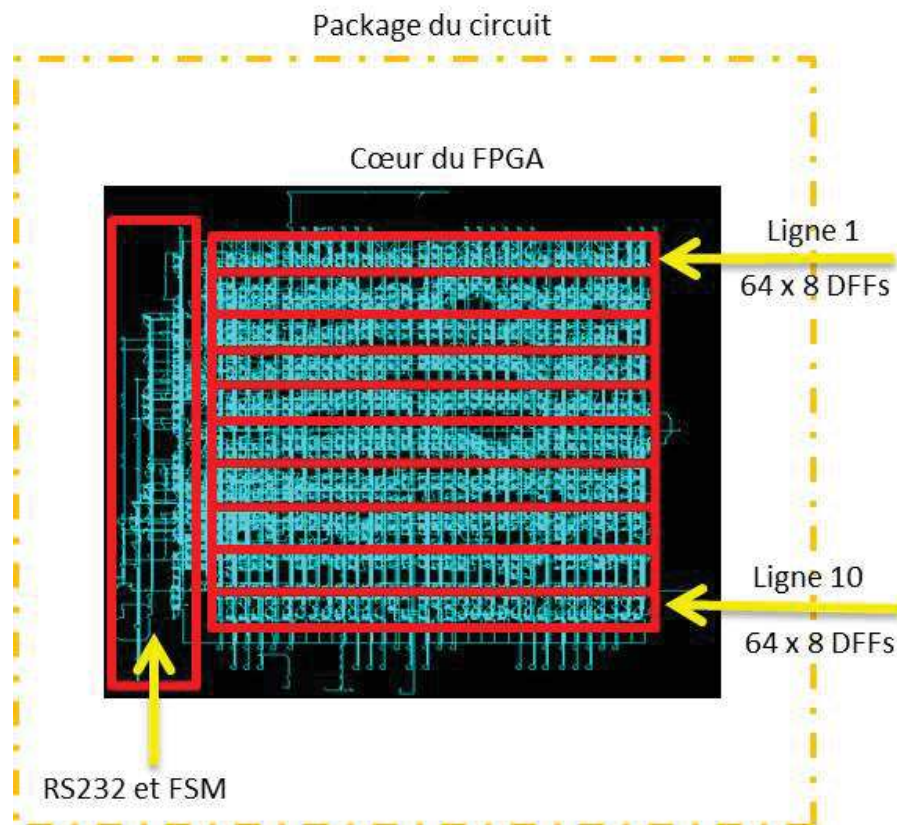
FIGURE 4.5: FIFO de 640x8 DFF implémentées sur FPGA pour démontrer l'occurrence des fautes de type bitset et bitreset
