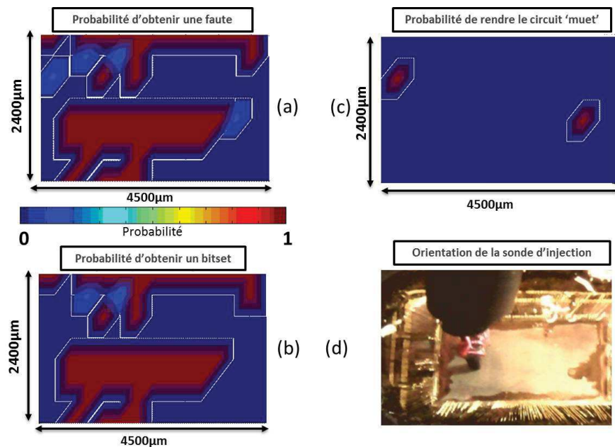
FIGURE 4.6: Probabilité de produire (a) une faute de n'importe quel type, (b) une faute de type bitset, (c) une faute de type 'muet'. (d) orientation de la sonde d'injection oméga
