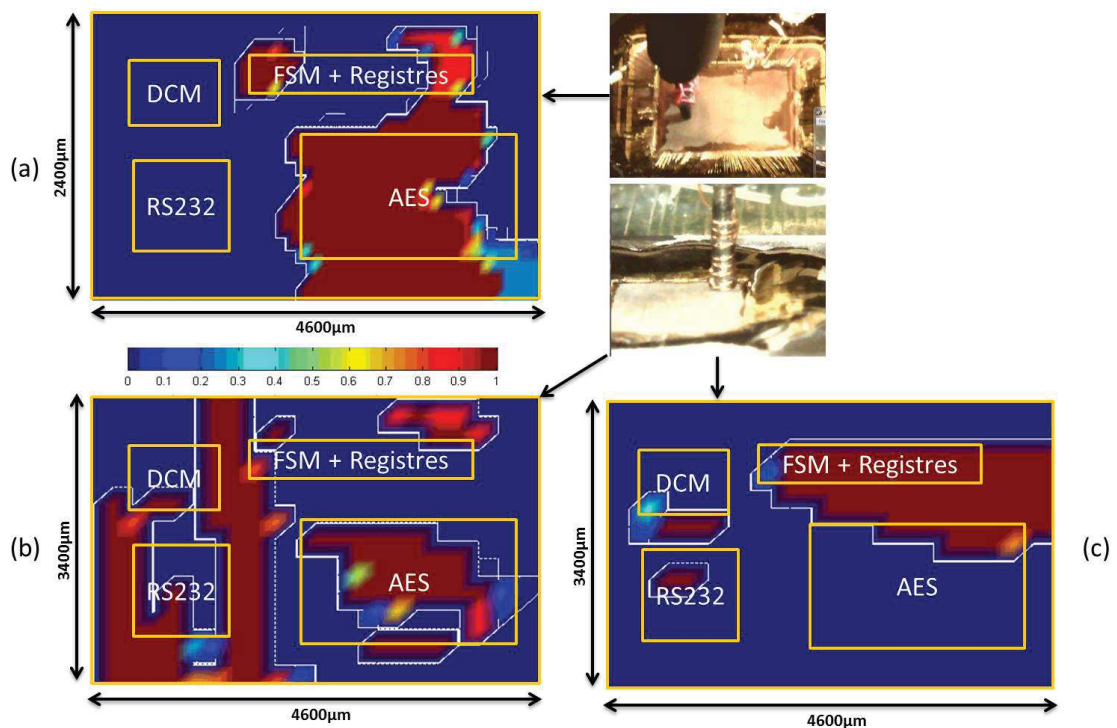
FIGURE 4.9: Probabilité de générer (a) un texte chiffré fauté avec la sonde d'injection oméga, (b) un texte chiffré fauté avec la sonde d'injection plate et (c) que le circuit soit muet avec la sonde d'injection plate
