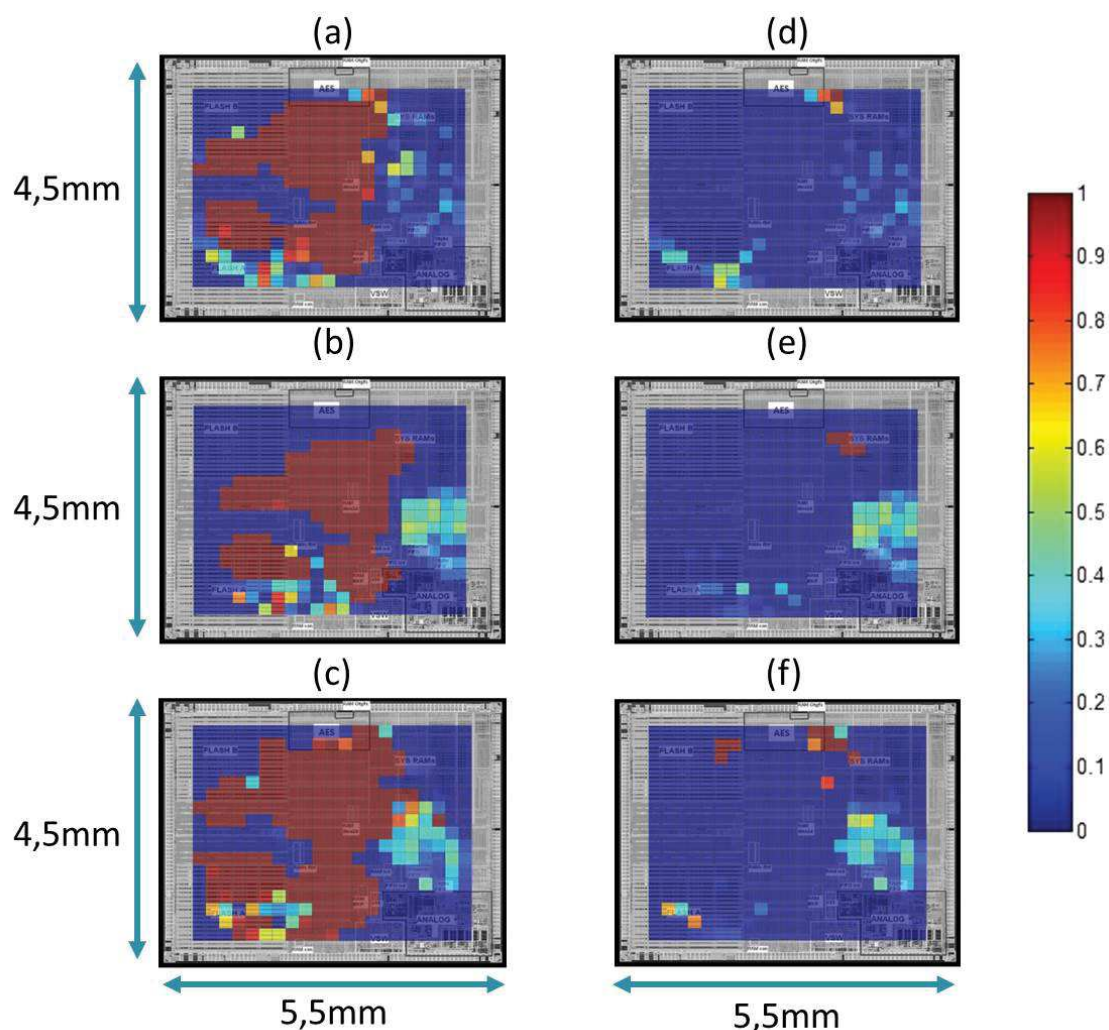
FIGURE 5.14: Cartographies (a,b,c) de la probabilité d'induire un comportement erroné quelconque lorsque le circuit a une polarisation de substrat de 0V(a), 200mV(b) et 400mV(c). Cartographies (d,e,f) de la probabilité de générer un chiffré fauté lorsque le circuit a une polarisation de substrat de 0V(d), 200mV(e) et 400mV(f)
