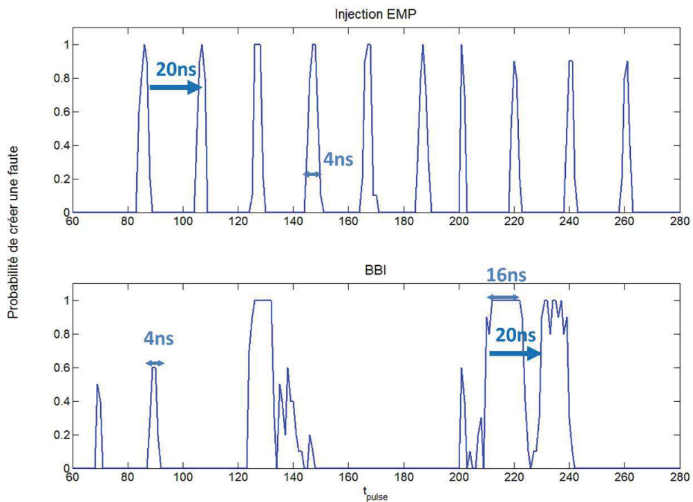
FIGURE 5.4: Probabilité de générer une faute en fonction de l'instant d'injection t_{pulse} de l'EMP et du pic de tension (BBI)
