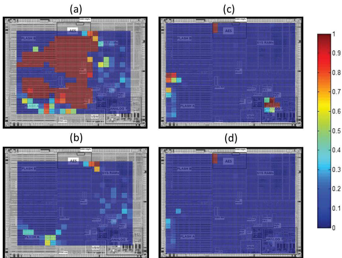
FIGURE 5.3: Probabilité d'induire : (a) et (c) des fautes de nature quelconque avec l'injection EMP (a) et BBI (c), (b) et (d) des fautes de chiffrement avec l'injection EMP (b) et BBI (d)
