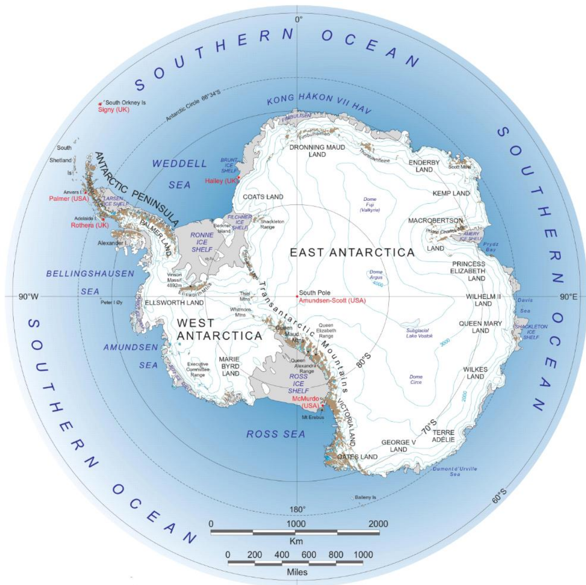
FIGURE 1.1 – Carte de l'Antarctique où l'on peut distinguer la partie orientale de l'Antarctique de l'occidentale séparée par la chaîne de montagnes transantarctiques avec la Péninsule qui s'allonge à l'ouest du continent. Le gris représente les plates-formes de glace, le blanc la glace continentale et le marron les parties rocheuses non glacées. Les principales terres et stations dont certaines seront citées dans le manuscrit sont montrées. Source : British Antarctic Survey.
