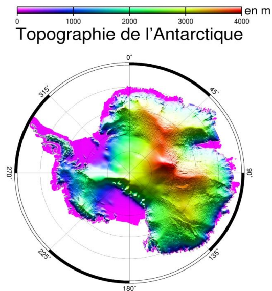
FIGURE 2.12 – Hauteur de glace mesurée par ERS1 et 2 en m. Crédits : Frédérique Rémy.
