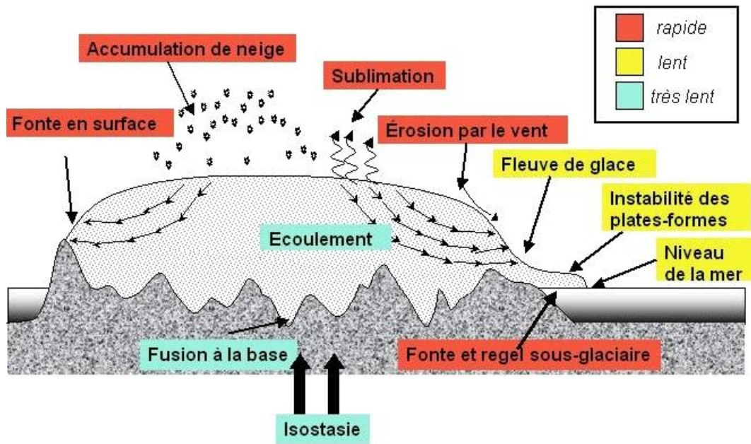
FIGURE 1.2 – Schéma des processus jouant sur la dynamique de l’Antarctique selon leur temps de réaction à une variation climatique. En rouge les processus rapides, en jaune les processus de durée intermédiaire, en bleu les processus lents. Crédits : Frédérique Rémy.
