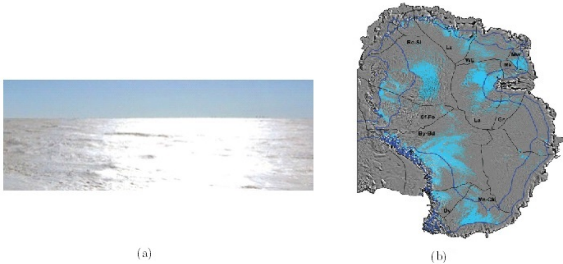
FIGURE 1.5 – Photo d’une surface vitrée en Antarctique (a), répartition sur l’Antarctique de l’Est de ces zones (b). Crédits : NSIDC et Frezzotti et al. [2002a] .
