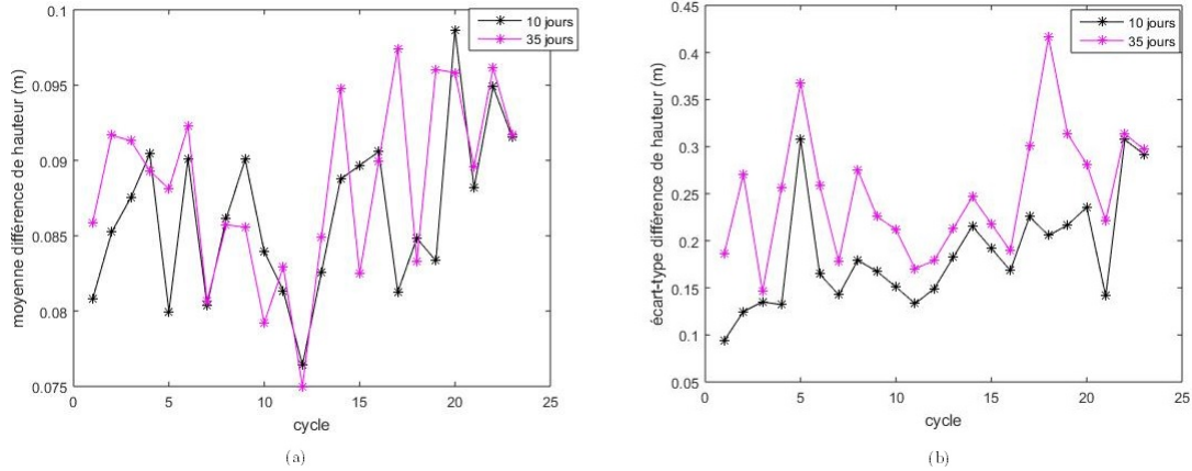
FIGURE 4.14 – Evolution par cycle sur tout le continent de la moyenne de la différence de hauteur (a) et de l'écart-type (b) en m.
