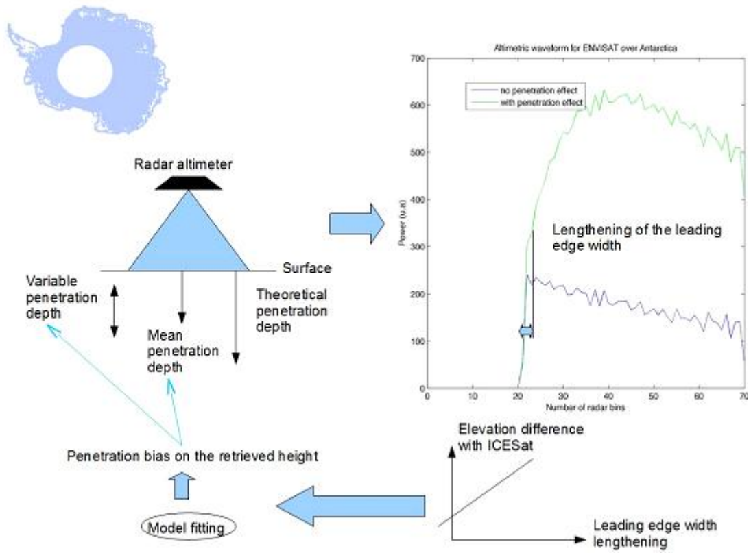
FIGURE 3.1 – Schéma récapitulatif de l'étude.
