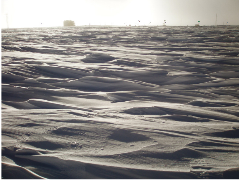
FIGURE 1.3 – Photo de sastrugi en Antarctique. Crédits : Alan Light.
