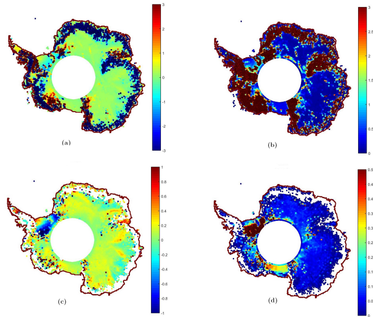
FIGURE 4.8 – Moyenne aux points de croisement de la différence de hauteur de glace en mètres (a), écart-type associé (b), moyenne de la différence de hauteur après editing (c), écart-type associé (d).
