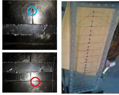
FIGURE 2.14 – Insertion des thermocouples dans les parois. Les marques rouge et bleus correspondent respectivement à une position en face du centre d’une chaufferette et entre deux chaufferettes. À droite : Insertion des 25 thermocouples dans la paroi en polycarbonate, À gauche : Zoom sur l’insertion de 2 thermocouples dans la paroi en acier inoxydable.
