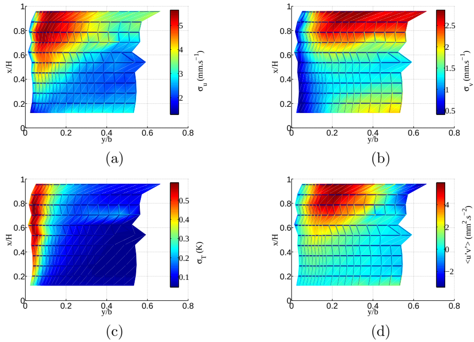
FIGURE 3.4 – (a) Fluctuations de vitesse verticale (b) Fluctuations de vitesse horizontale (c) Fluctuations de température (d) Tenseur de Reynolds. Les cartes sont construites par interpolation linéaire des mesures obtenues sur un maillage 11 \times 21 .
