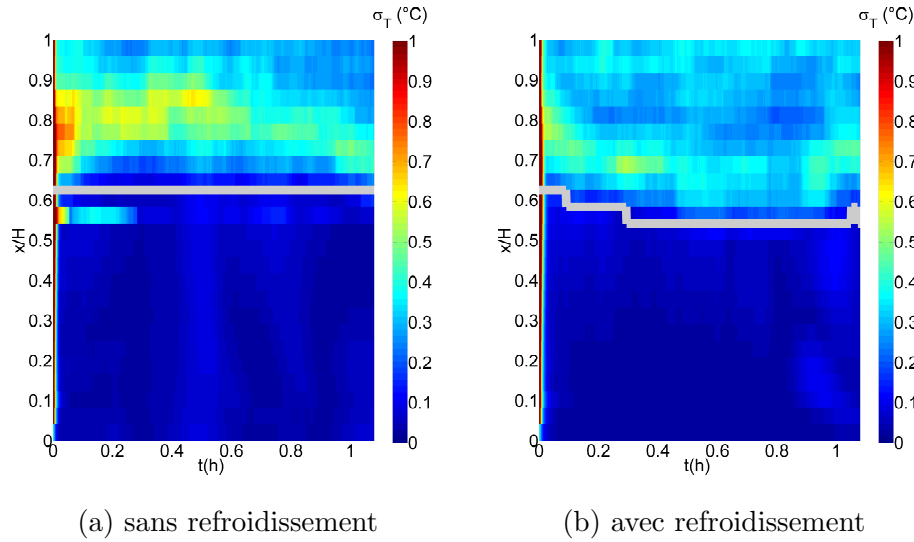
FIGURE 4.19 – Profils de la déviation standard de la température de la paroi chaude calculée sur une plage glissante 10 min pour deux expériences commençant avec une stratification thermique élevée. La courbe grise représente la position de la température maximale. (a) Cas sans refroidissement (Exp.12), (b) cas avec refroidissement (Exp.17).
