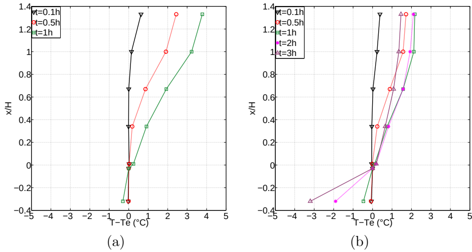
FIGURE 4.14 – Évolution des profils de stratification thermique externe (a) Exp.7 (sans refroidissement) (b) Exp.20 (avec refroidissement)
