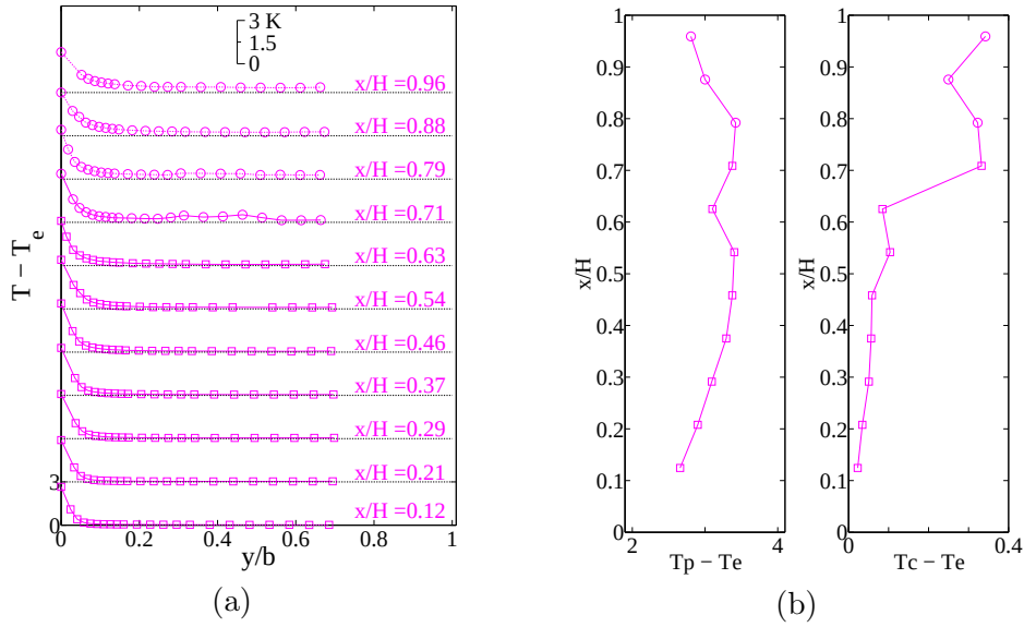
FIGURE 3.2 – Écarts de température mesurées par rapport à l'entrée. (a) Profils de température moyenne pour 11 positions verticales. Les marqueurs ( \square ) et ( \circ ) indiquent les parties du canal où \Delta U augmente et diminue respectivement. (b) Température de paroi à gauche et température au centre du canal à droite pour 11 positions verticale le long du canal.
