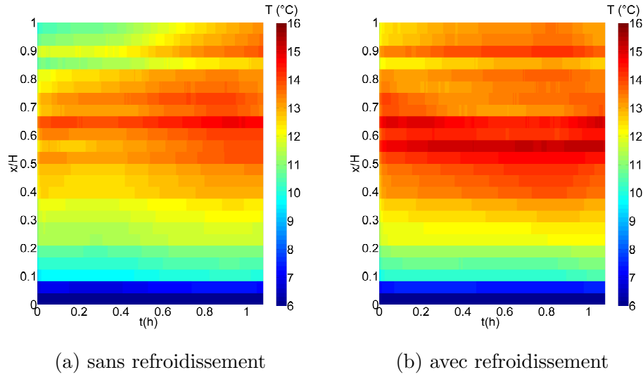
FIGURE 4.18 – Profils de température de la paroi chaude calculée sur une plage glissante 10 min pour deux expériences commençant avec une stratification thermique élevée (a) cas sans refroidissement (Exp.12) (b) cas avec refroidissement (Exp.17)
