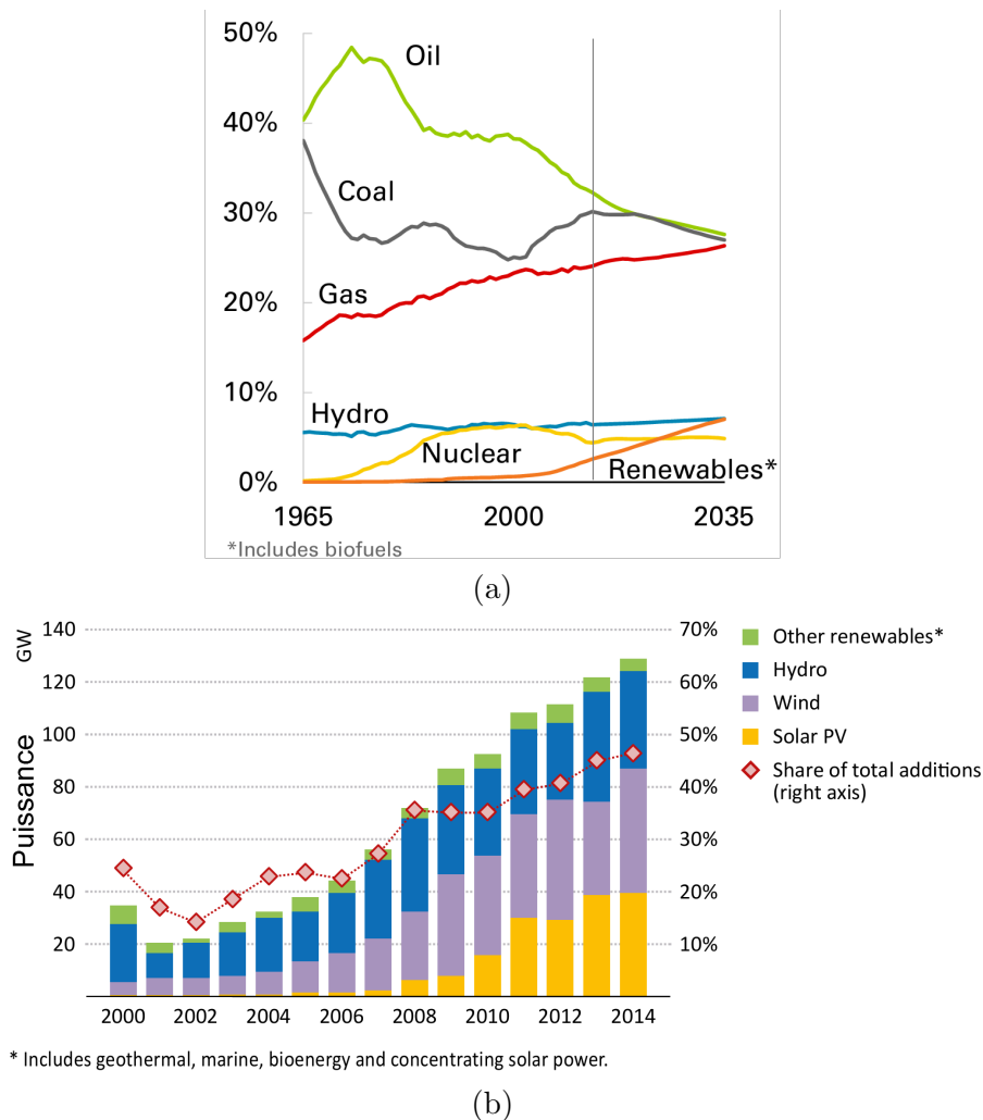
FIGURE 1.3 – (a) Évolution de l'énergie primaire par source au niveau mondial. Figure extraite de BP Energy Outlook 2035 [16]. (b) Répartition de la puissance installée annuellement en ressources renouvelables au niveau mondial et part de cette puissance installée par rapport à la puissance énergétique totale mondiale installée annuellement. Figure extraite du rapport de l'IEA [4].
