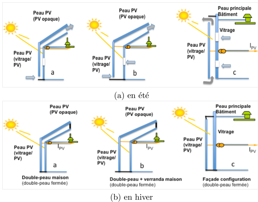
FIGURE 1.11 – Schémas de la double-peau photovoltaïque en été et en hiver. Schéma à gauche en configuration toiture façade, au centre en configuration toiture façade avec veranda, et à droite configuration façade.
