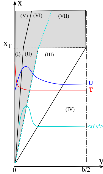
FIGURE 3.6 – Découpage du demi canal gauche. Les zones et leurs épaisseurs sont données dans la table 3.1
