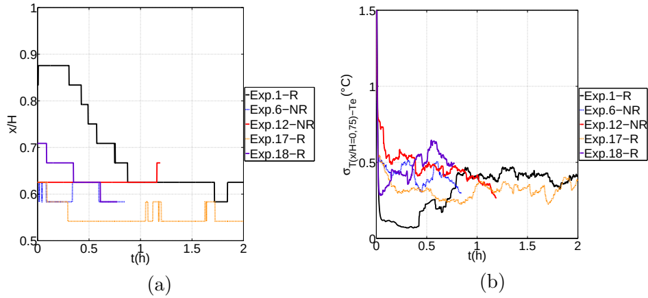
FIGURE 4.17 – (a) Évolution en temps de la position de la température maximale de paroi (calcul sur une plage glissante de 10 minutes) pour les 5 expériences commençant avec une stratification thermique élevée (b) Évolution de la déviation standard de la température de paroi à x/H = 0,75 (calcul sur une plage glissante de 10 minutes) pour les 5 expériences commençant avec une stratification thermique élevée
