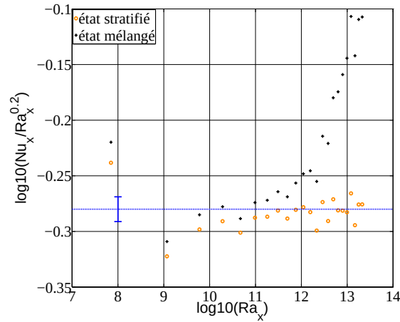
FIGURE 4.29 – Relation entre les nombres de Nusselt et Rayleigh : \log \left( \frac{Nu_x}{Ra_x^{0,2}} \right) en fonction de \log(Ra_x) . Une droite horizontale est tracée pour \log_{10} \left( \frac{Nu_x}{Ra_x^{0,2}} \right) = -0.28 . La barre d'erreur est également tracée.
