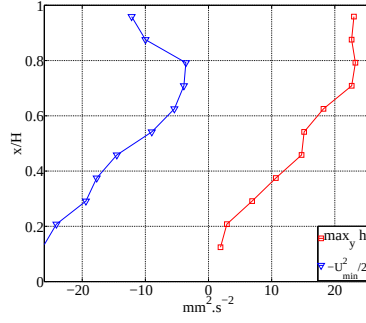
FIGURE 3.9 – -\frac{1}{2}U_{\min}^2 et \max_y h' en fonction de x/H
