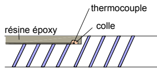
FIGURE 2.15 – Fixation des thermocouples dans la paroi en polycarbonate. (a) Schéma en coupe ; (b) rendu final.
