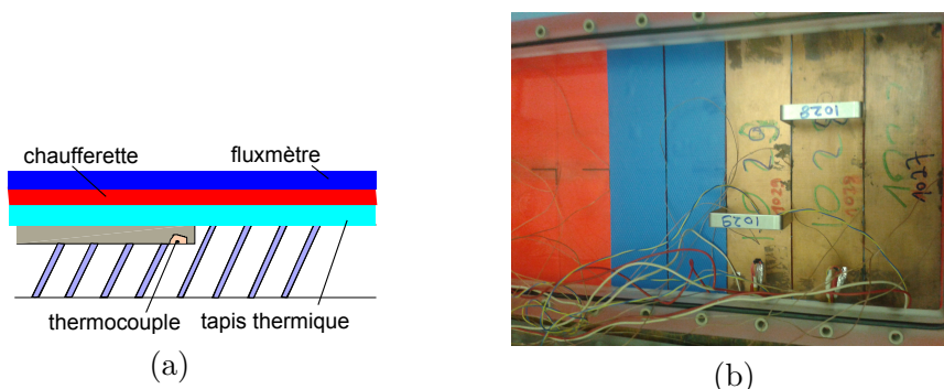
FIGURE 2.9 – (a) Schéma des tapis thermique (bleu) positionné entre la paroi et les chaufferettes. (b) Photo prise lors de la mise en place des chaufferettes : on voit deux tapis thermiques (bleu) ; trois chaufferettes (cuivre) et deux ponts de rigidification de paroi.
