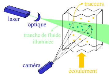
FIGURE 2.16 – Schéma d'un système de mesure par PIV
