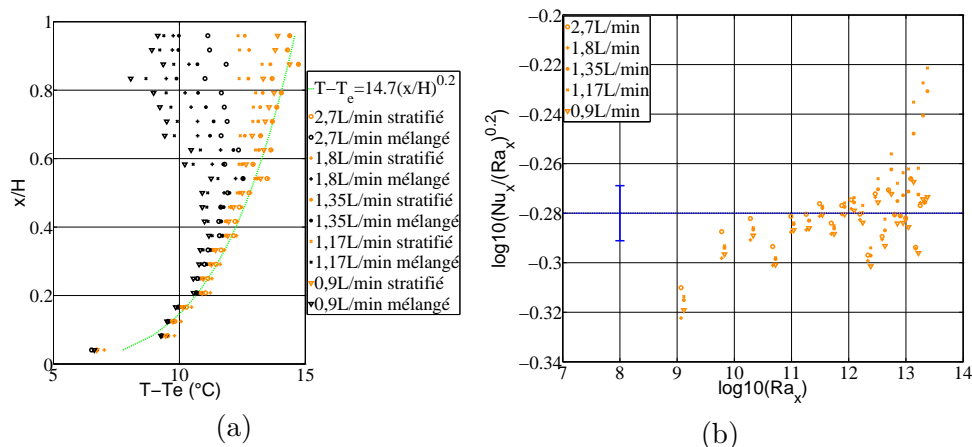
FIGURE 4.39 – Comparaison entre les expériences avec différents débits de pompe du circuit de refroidissement. (a) Profils de température moyenne pour l'état stratifié et mélangé (b) Relation Nu_x - Ra_x pour l'état stratifié
