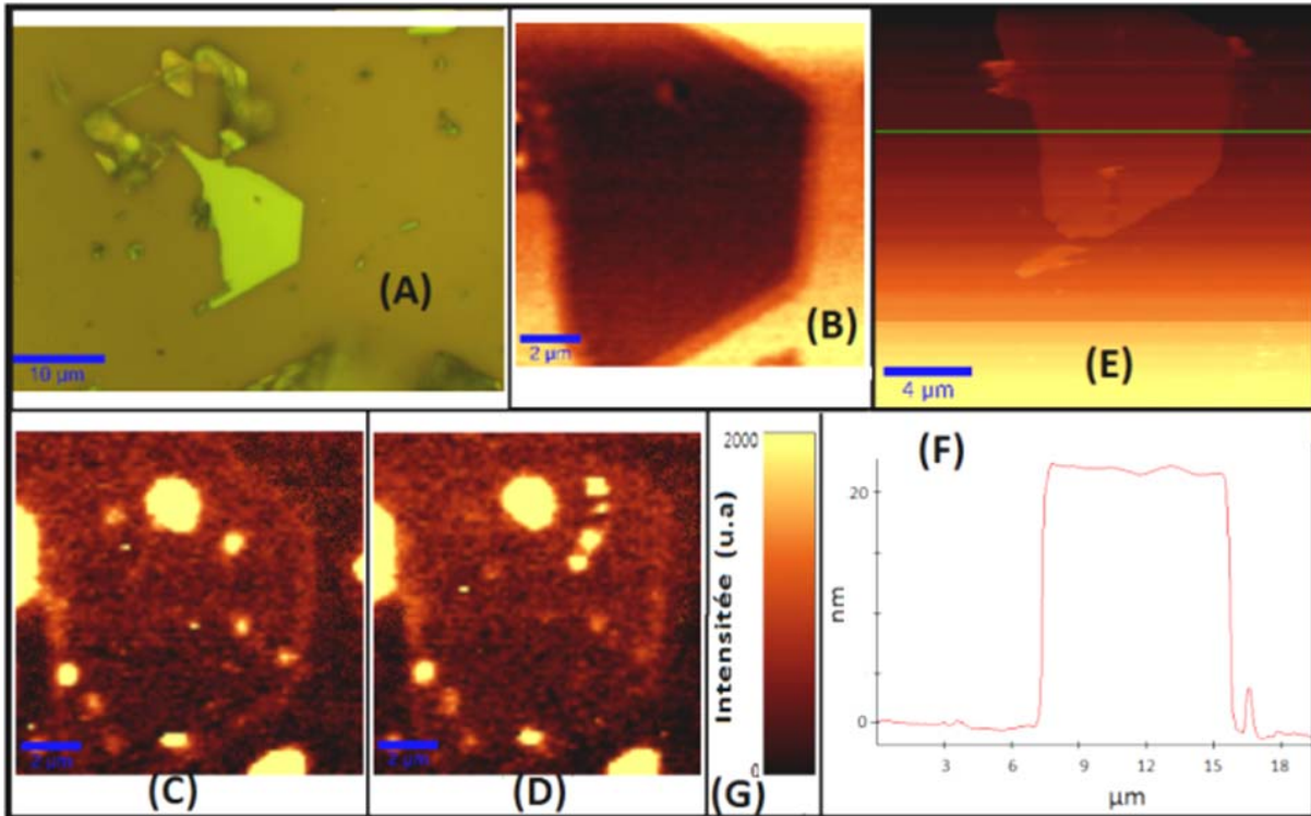
Figure 136: Image réalisée grâce à la nouvelle plateforme Raman-AFM-Résiscope développé au laboratoire. (A) image optique, (B) cartographie Raman du pic du silicium, (C) cartographie du pic D des GMF, (D) cartographie du pic 2D des GMF, (G) barre de référence de l'intensité Raman, (E) Image topographique par AFM et (F) profil tirée de l'image (E).
