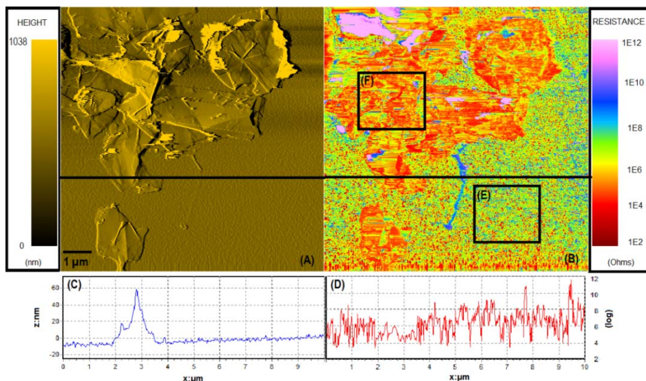
Figure 98 : Cartes topographique et électrique d'un dépôt par spray de la suspension 8 sur un substrat d'or; pointe PtIr à une force de 50 nN (A) image topographique. (B) Image de la résistance locale de la surface. (C) et (D) profil de la topographie et profil de résistance extrait de la ligne. (E) zone d'étude de la résistance de l'or. (F) zone d'étude de la résistance du graphène
