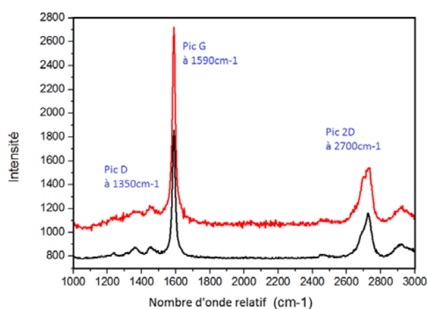
Figure 81 : Spectres Raman réalisés à une puissance de 1.6 mW et à \lambda = 532 nm pour le laser, de la suspension 4 déposé par spray sur un substrat de SiO 2 .
