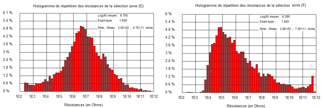
Figure 72: Histogramme de répartition des résistances, à la surface d'or de la Figure 71 (E) et aux feuillettes de graphène Figure 71 (F).
