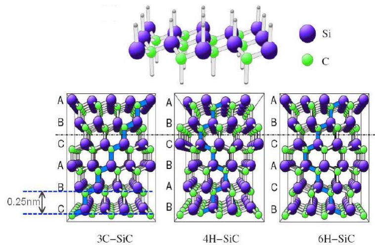
Figure 23 : Illustration des polytypes de SiC les plus couramment utilisés en épitaxie.
