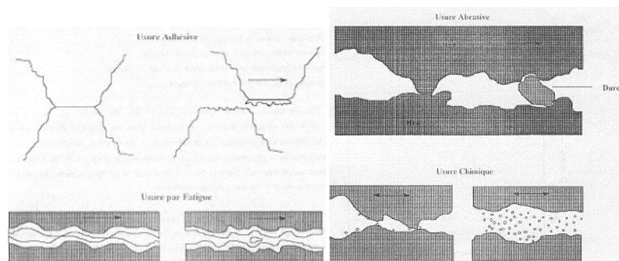
Figure 6: Les différents types d'usure [39]
