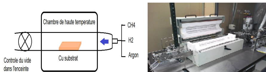
Figure 21 : Schéma et photographie d'une chambre CVD.
